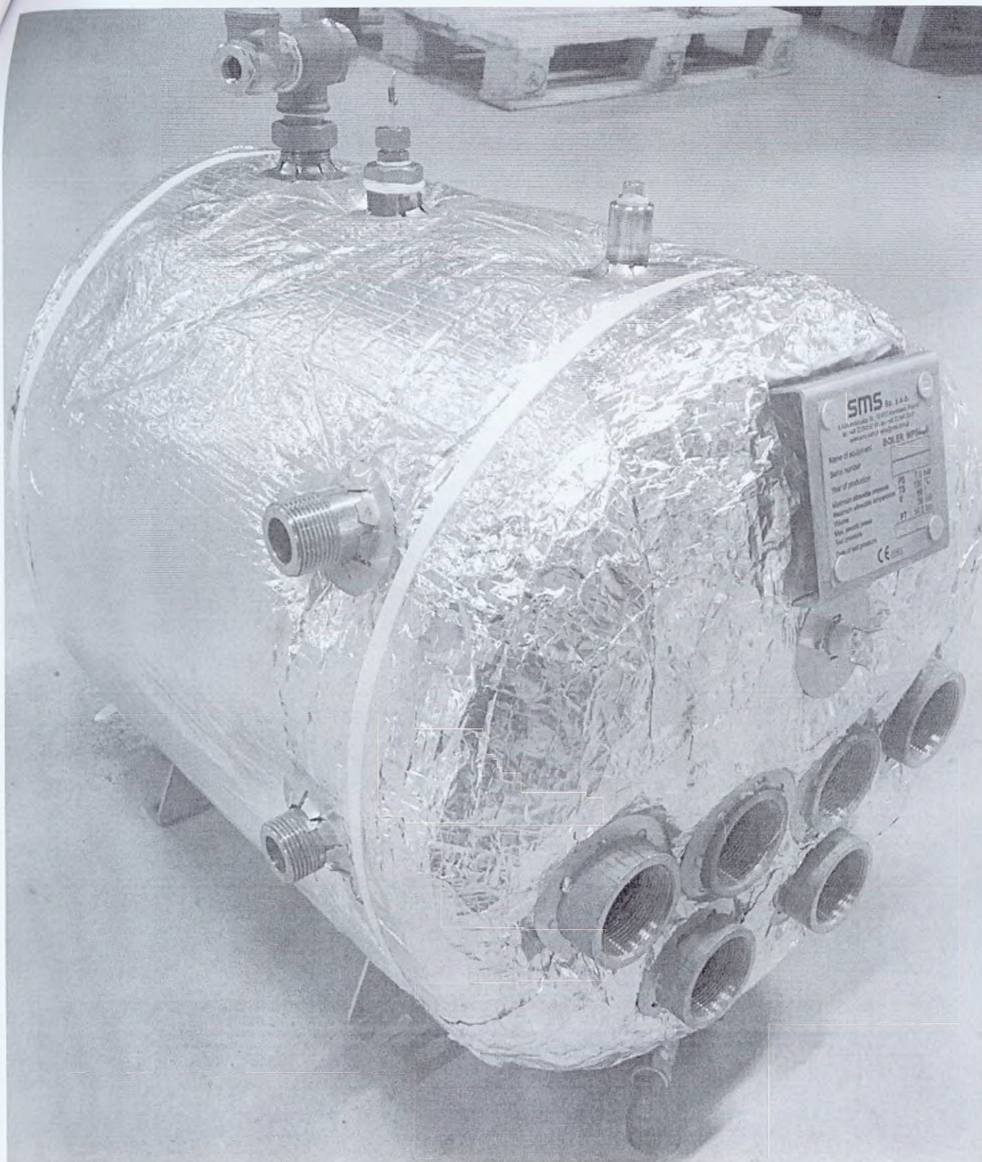
Стерилизатор паровой с автоматическим управлением PHS (ПиЭйчЭс) – 800 Парогенератор.
