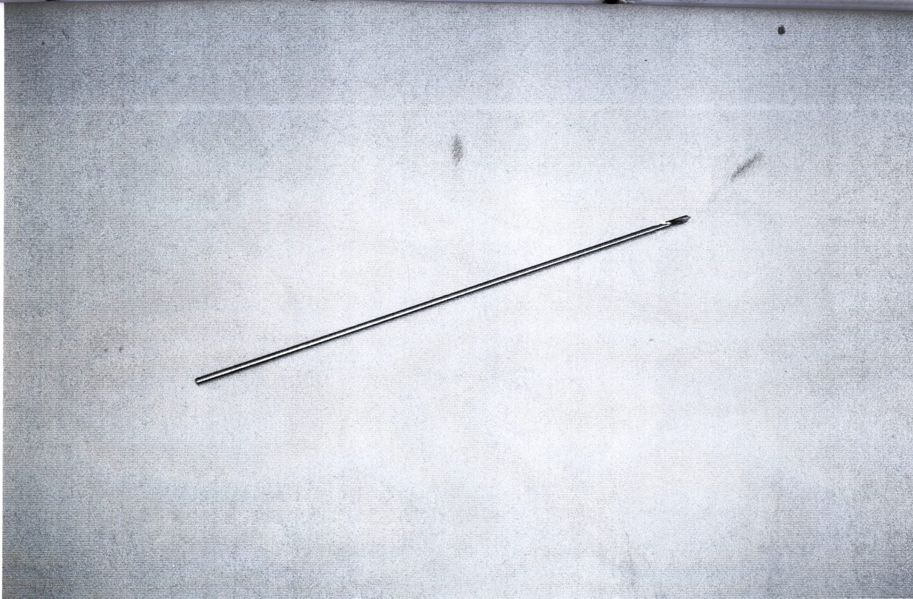
Принадлежности для фиксаторов наружных временных стерильных Dolphix для остеосинтеза: Сверло диаметр 3 мм, длина 165 мм.
