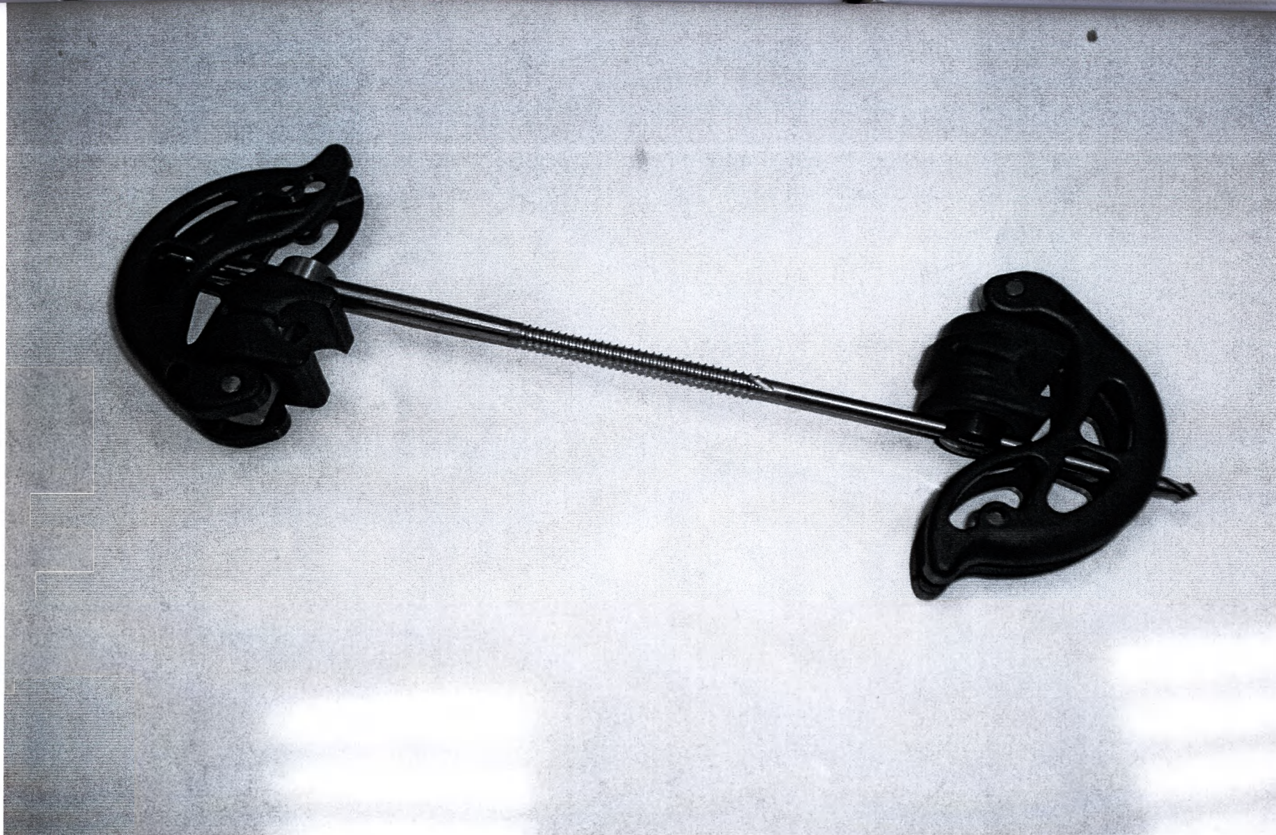
Фиксаторы наружные временные стерильные Dolphix для остеосинтеза в отдельных упаковках- Зажим с трансфиксирующим костным винтом- диаметр 5 мм, длина 220 мм.
