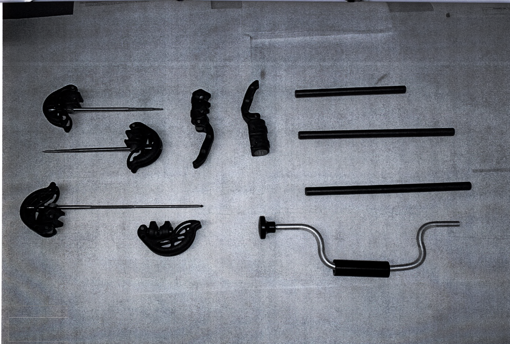
Набор Dolphix для переломов пилона: Зажим с костным винтом- диаметр 6 мм, длина 160 мм - 2 шт; Зажим с трансфиксирующим костным винтом- диаметр 5 мм, длина 220 мм - 1 шт; Зажим для соединения стержня со стержнем - 2 шт; Стержень рентгенопрозрачный - диаметр 12 мм, длина 200 мм- 1 шт; Стержень рентгенопрозрачный - диаметр 12 мм, длина 280 мм- 2 шт; Дрель ручная - 1 шт.
