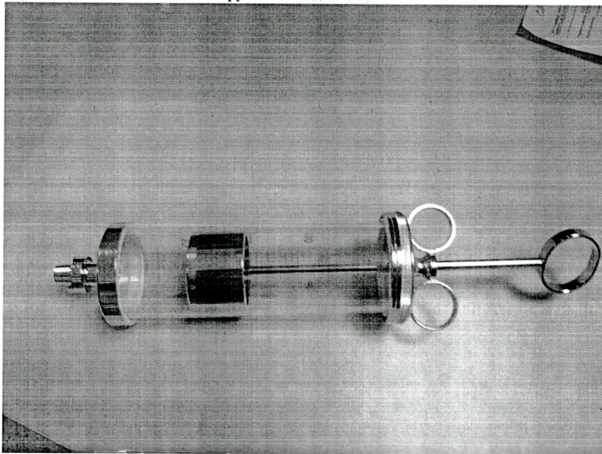
Рисунок 48. Трубки и устройства отсасывающие / ирригационные / внешние / внутренние/нагнетающие (Suction / irrigation/ outer/ inner/ insufflation tubes and unit)
