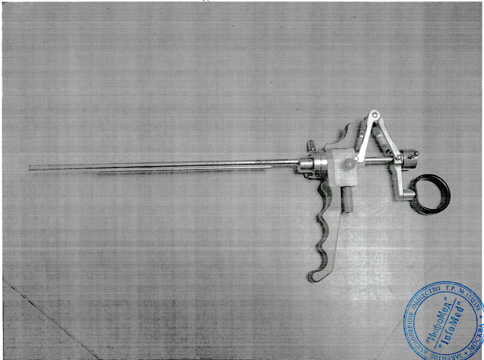
Рисунок 41. Рабочие элементы (Working elements)
