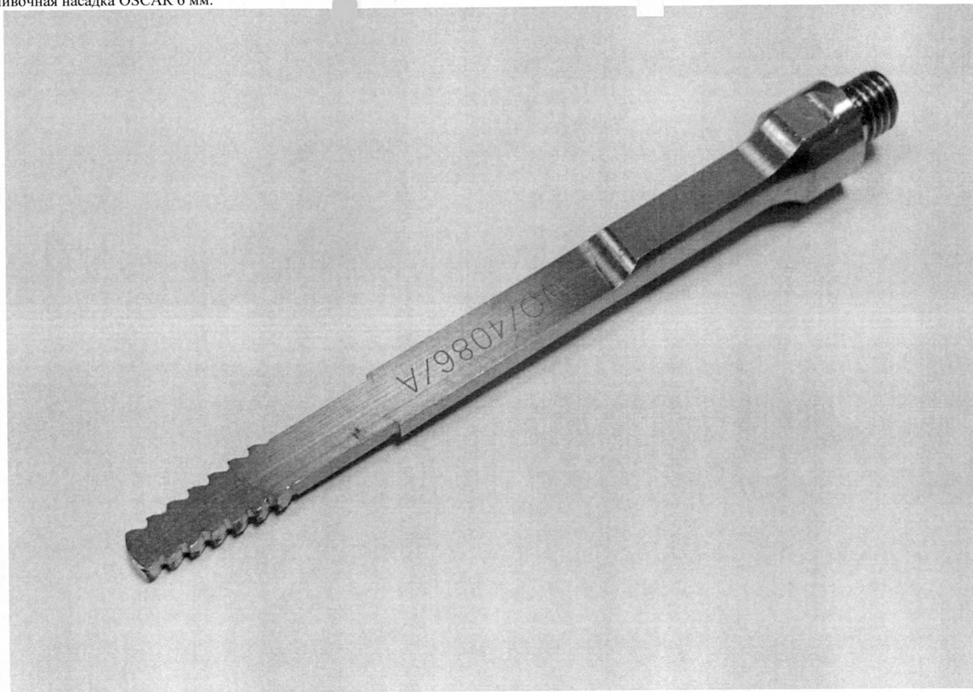
Прошивочная насадка OSCAR 6 мм.
