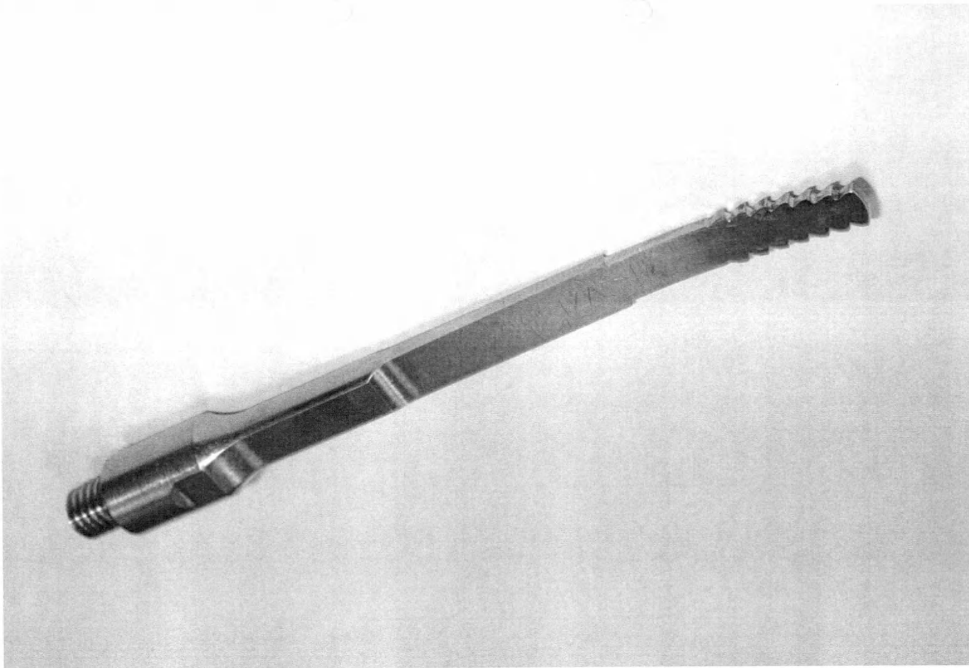
Одноразовая прошивочная насадка 6 мм, тонкий штифт 4 мм.
