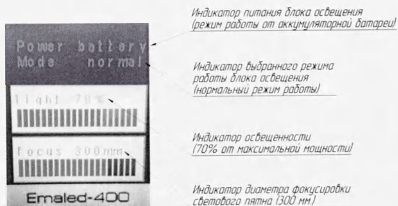
Рисунок А.20 – Индикация панели управления
