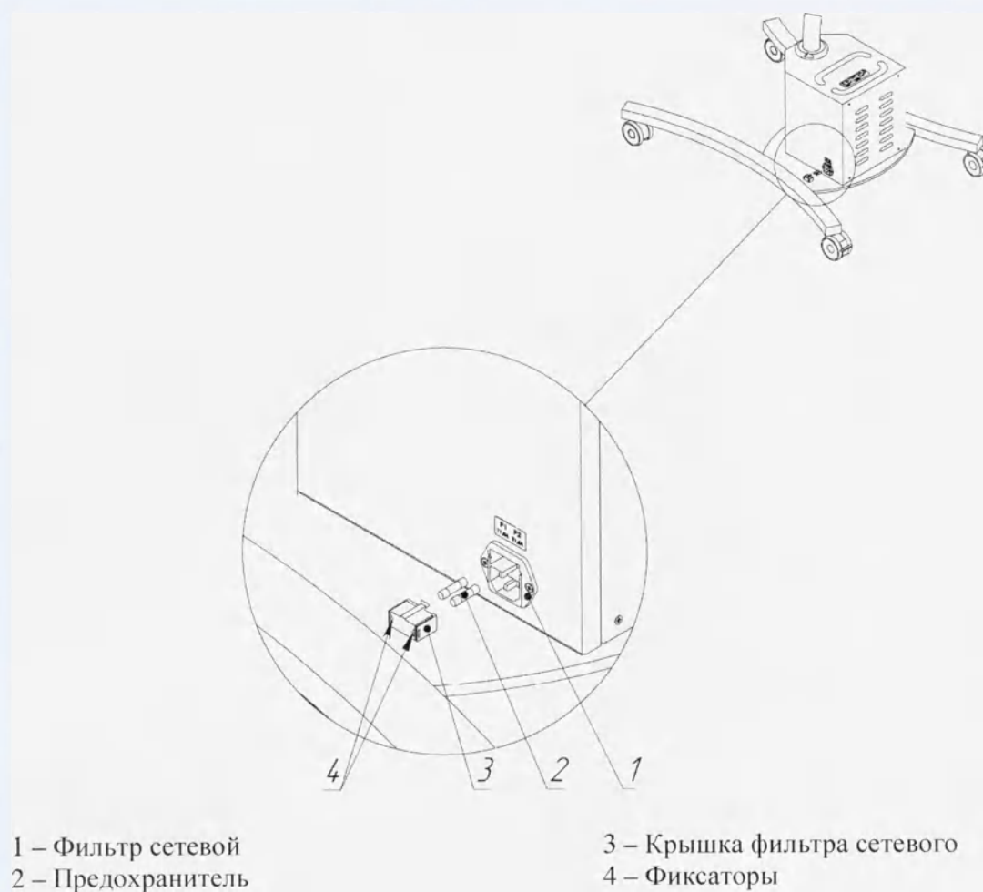
Рисунок А.19 – Замена предохранителей фильтра в блоке питания
