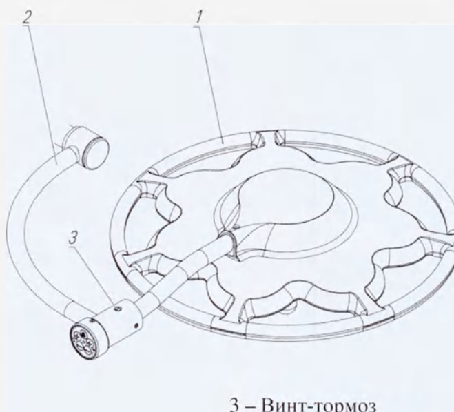
Рисунок А.13 – Настройка усилия поворота блока освещения
