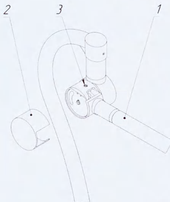
Рисунок А.11 – Монтаж блоков освещения с одним дуговым шарниром
