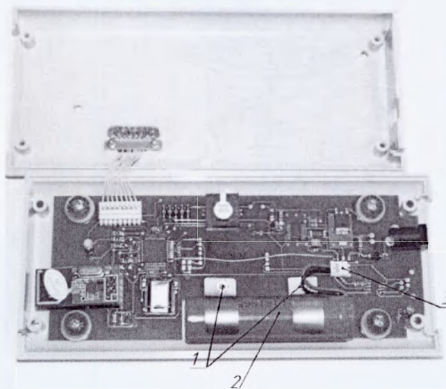
Рисунок А.30 – Задняя панель корпуса пульта управления видеокамерой
