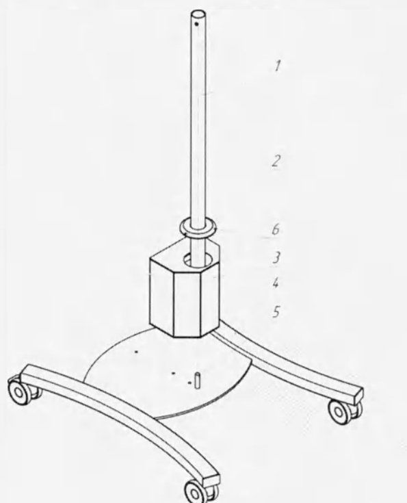
4 – Опора 5 – Болт М12х50 с шайбой 6 – Винт установочный
