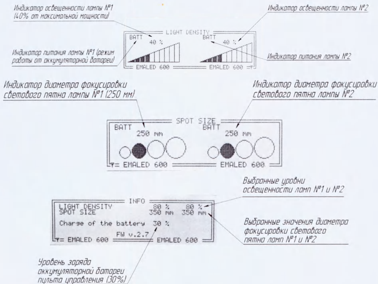
Рисунок А.24 – Индикация пульта управления
