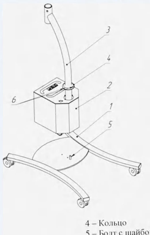
Рисунок А.3 – Установка блока питания на опору
