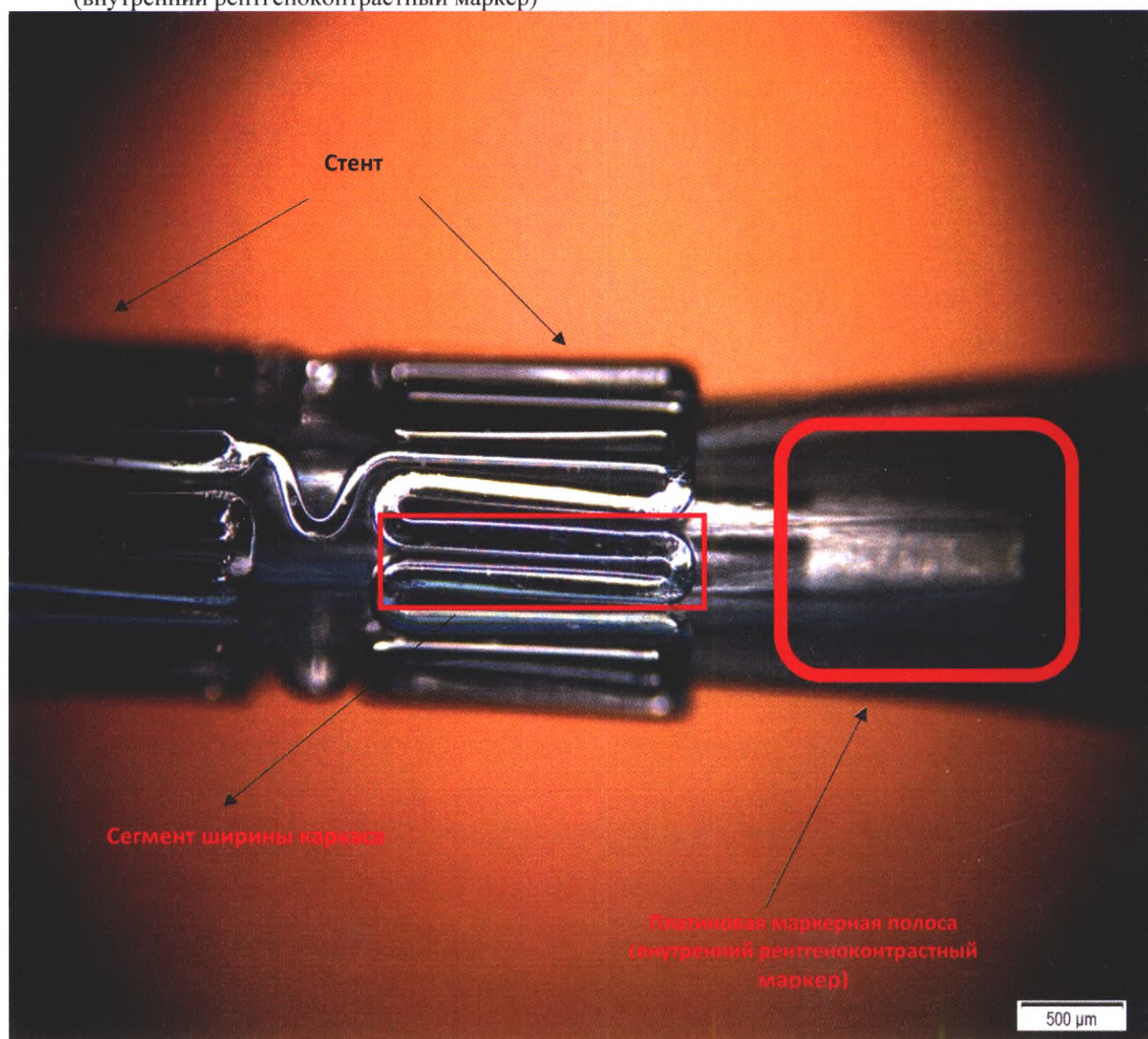
Фото 6. Стент под микроскопом, проксимальный конец, платиновая маркерная полоса (внутренний рентгеноконтрастный маркер)
