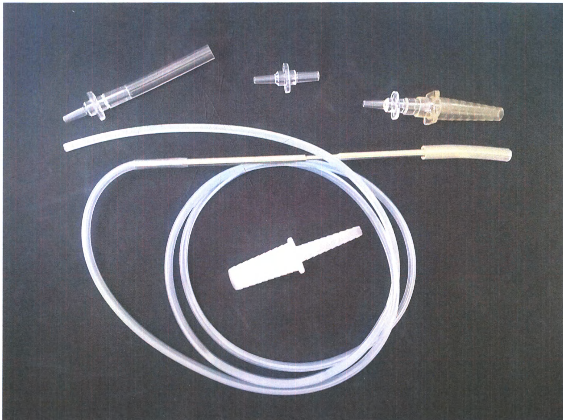
Общий вид изделия: Трубка дренажная силиконовая Biovac, одноразового использования, в исполнении MW-J3105.
