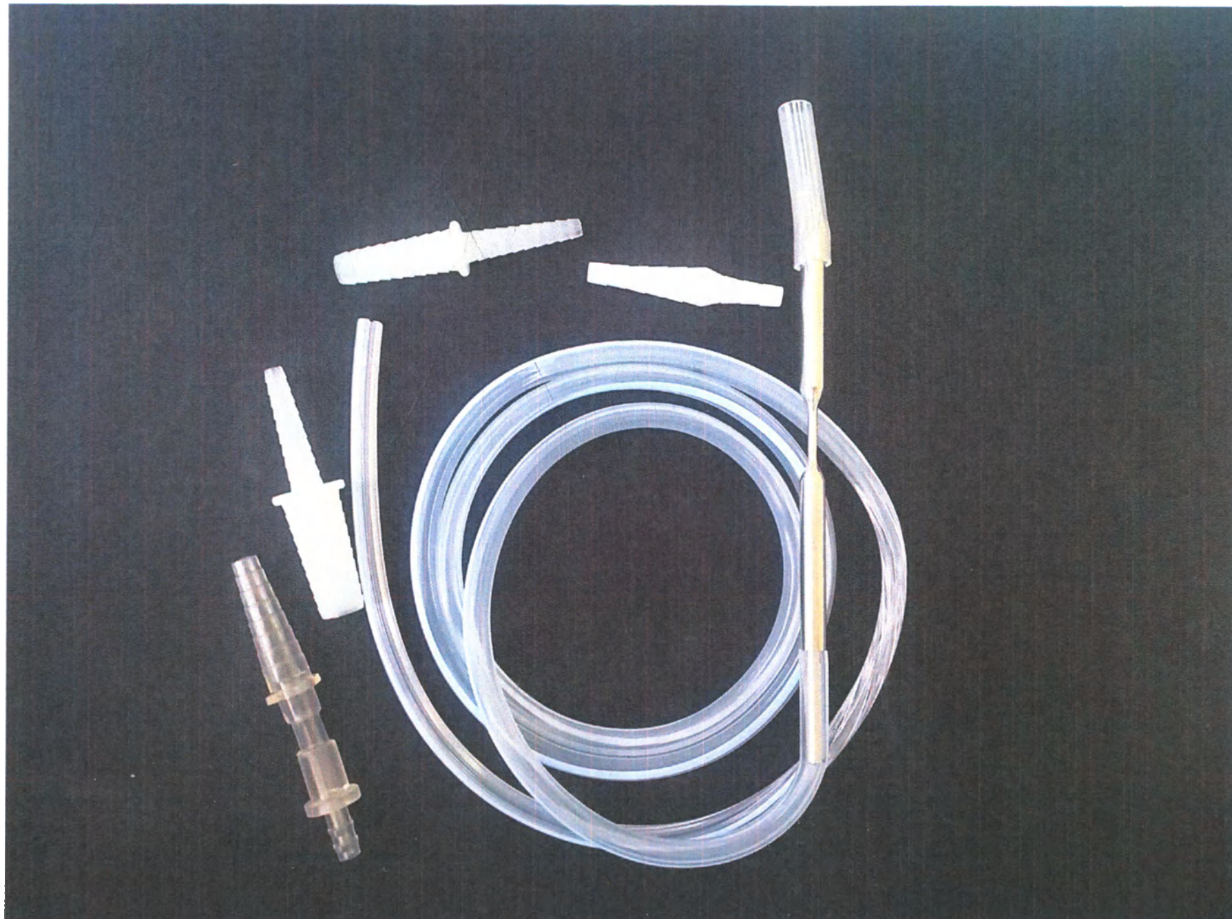
Общий вид изделия: Трубка дренажная силиконовая Biovac, одноразового использования, в исполнении MW-J3195.
