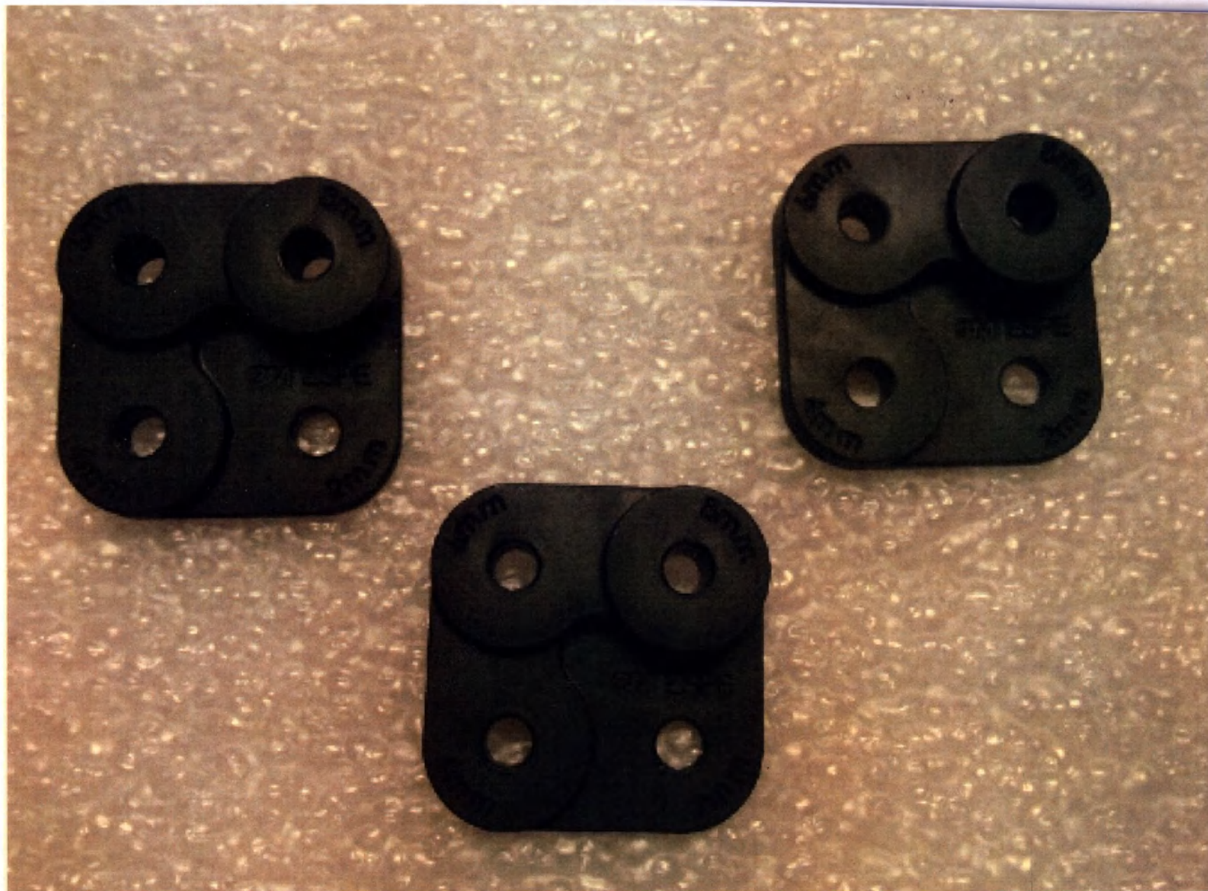
Рисунок 16 - Шаблон для проверки глубины полимеризации (Curing disks) 3 шт.
