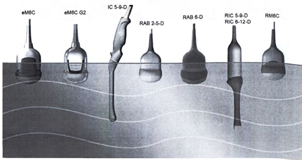
Рисунок 5-1 Уровни погружения датчиков
