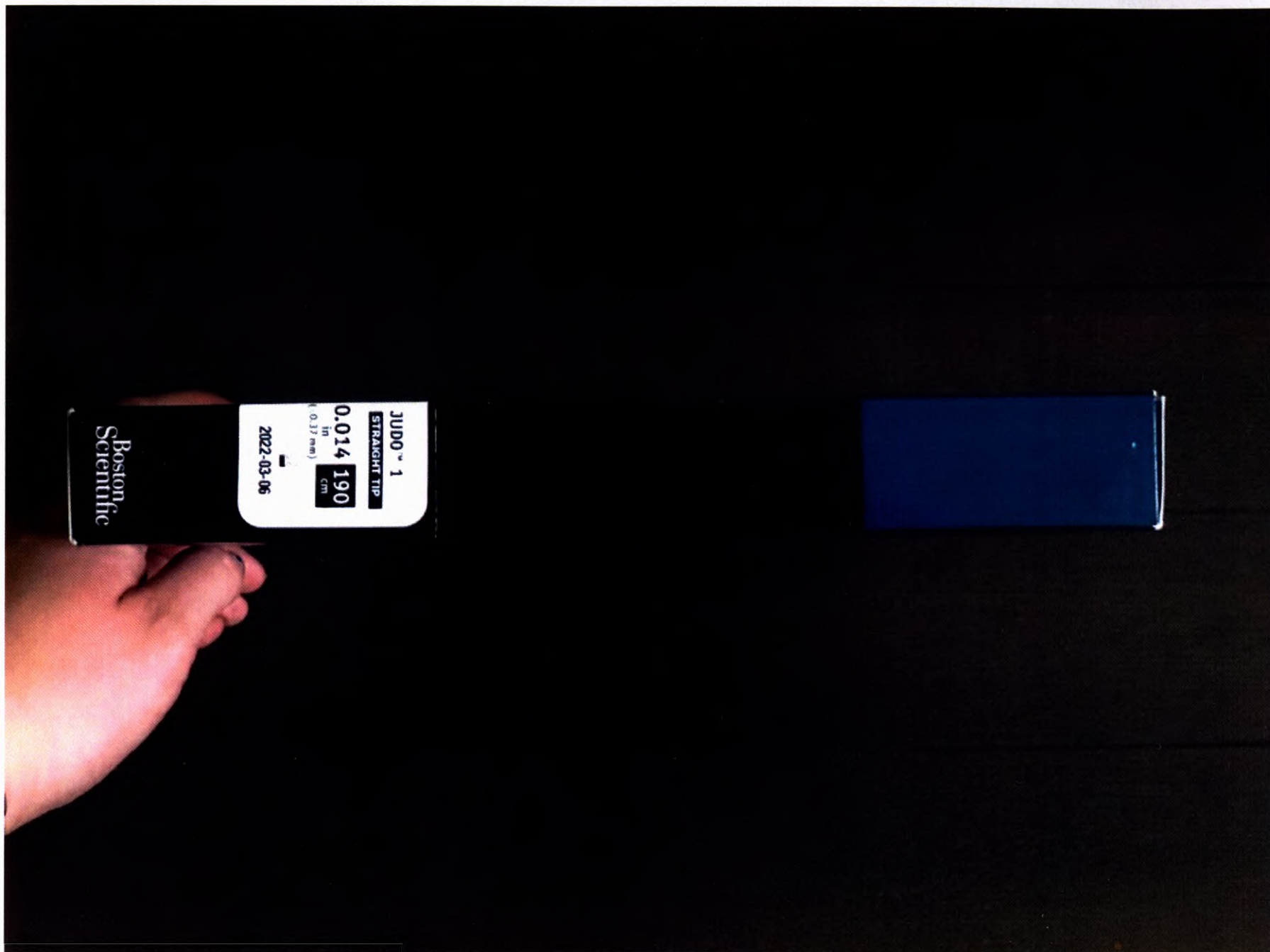
Проводник Judo 1 длиной 190 см, диаметром \leq 0,37 мм (0.014 дюйма), прямой кончик – Коробка (вид сбоку)
