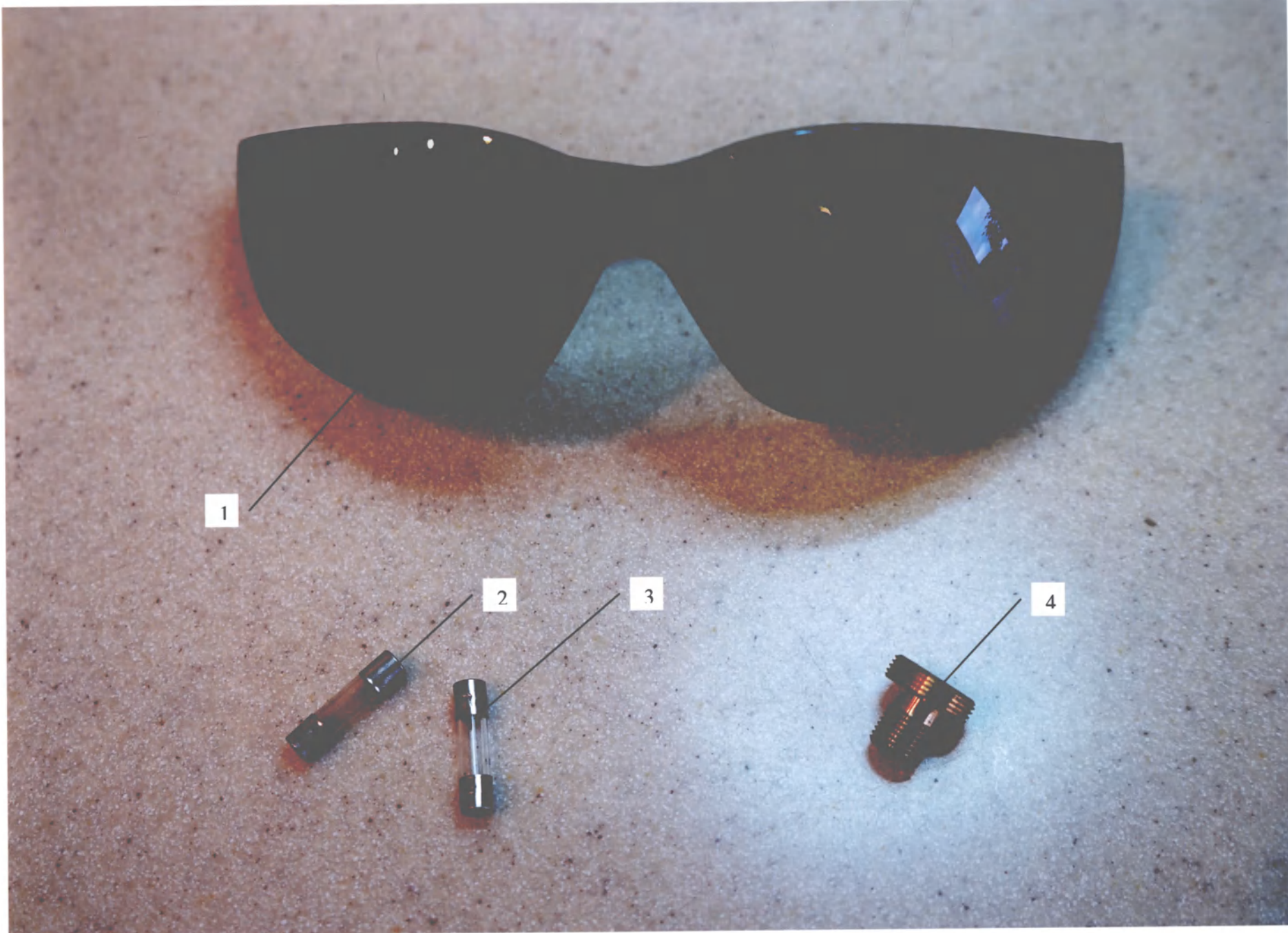
1 – очки защитные IZ-11001 (общие для моделей 01 и 02), 2 – вставка плавкая ВП1-1-1,0 А, 3 – вставка плавкая ВП1-1-0,5 А 4 – световодный соединитель (общий для моделей 01 и 02)
