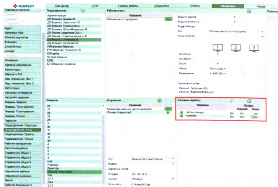
Рис. 38. Программа Numedy.DeviceManager.
