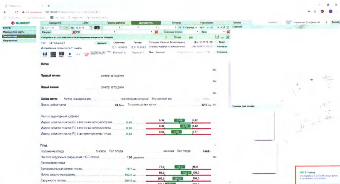
Рис. 39. Программа Numedy.PACS.
