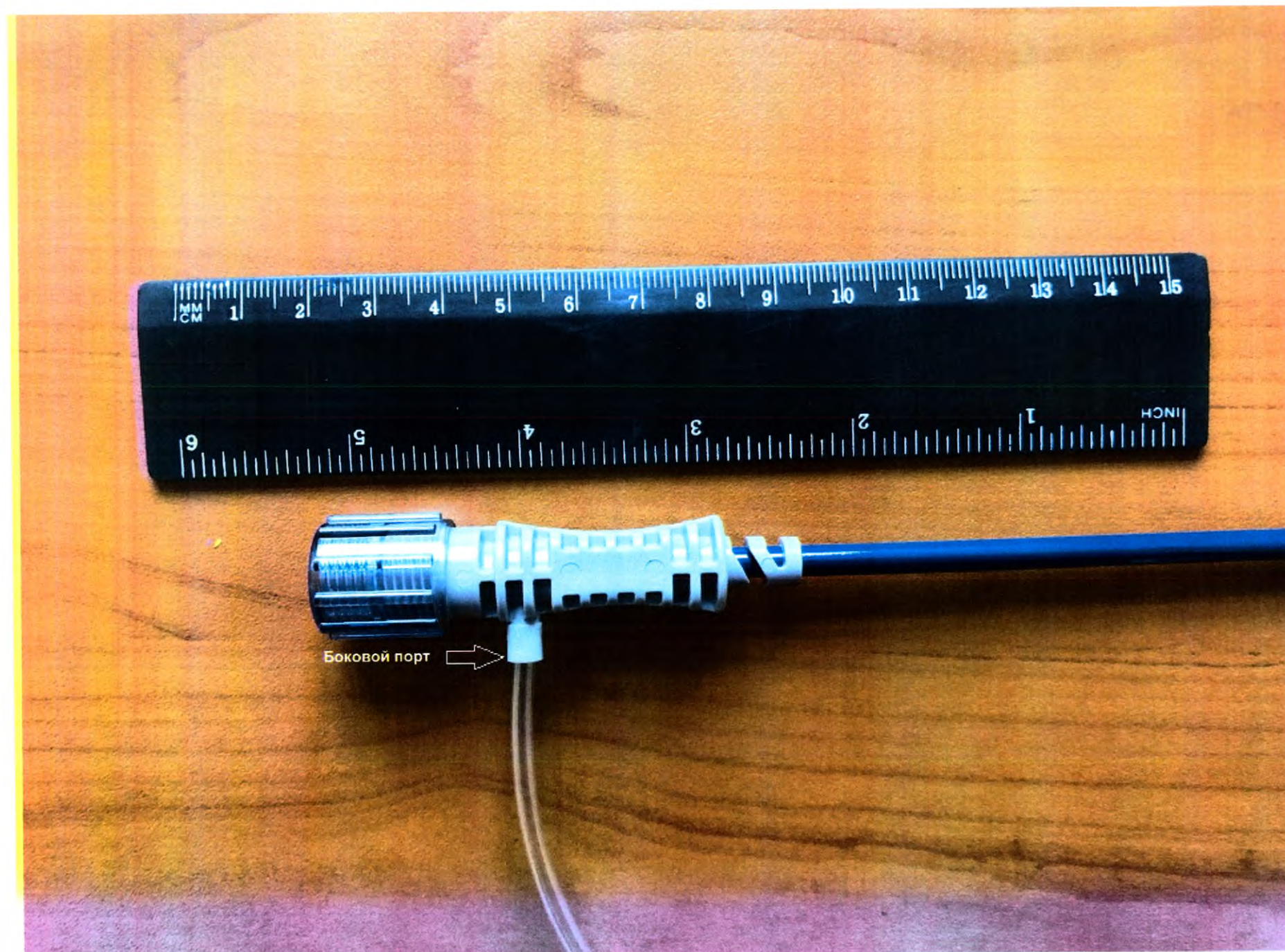
Хаб и боковой порт проксимальной части интродьюсера системы доступа Watchman TruSeal
