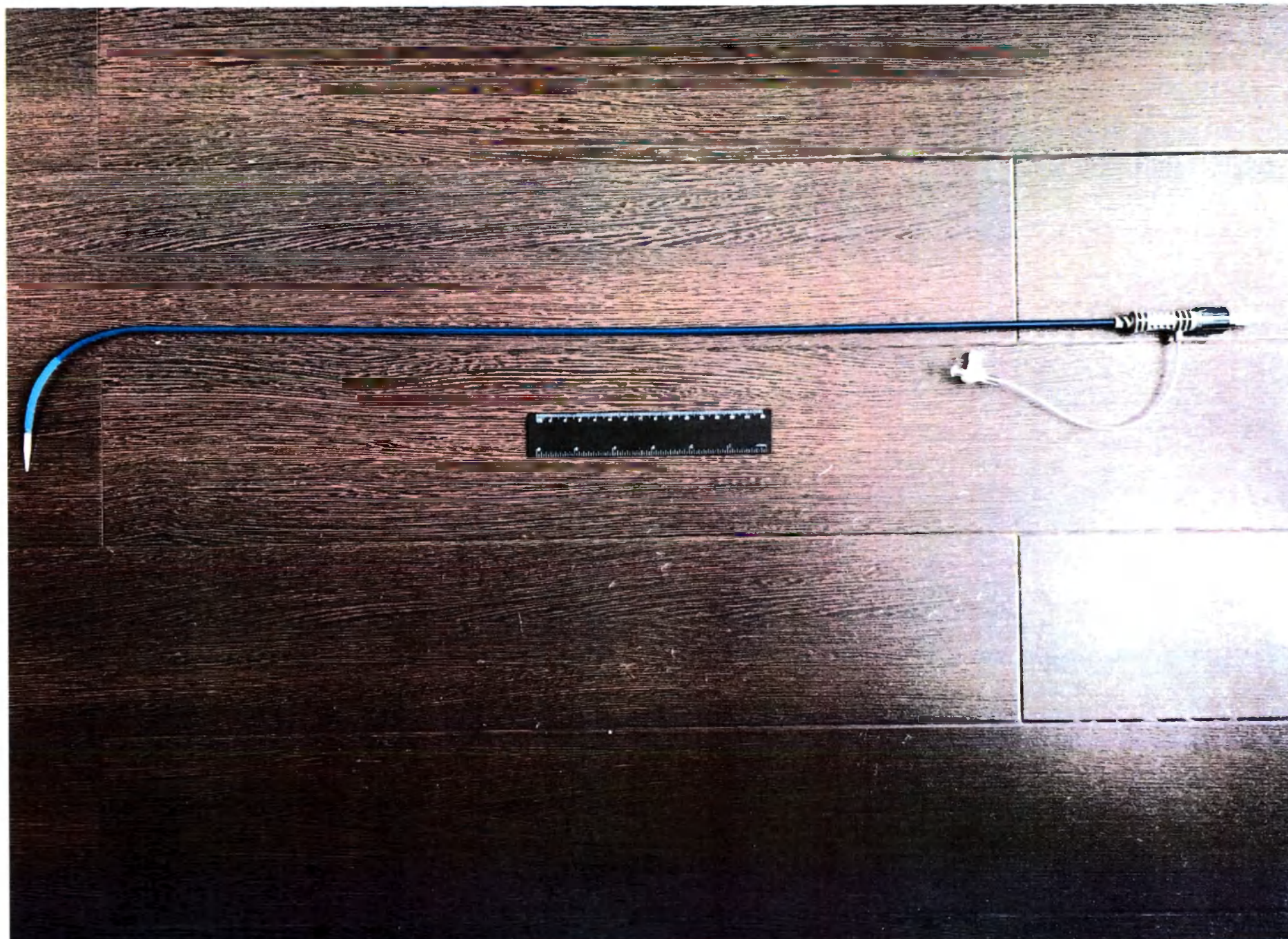
Собранный вид системы доступа Watchman TruSeal: интродьюсер доступа и дилататор
