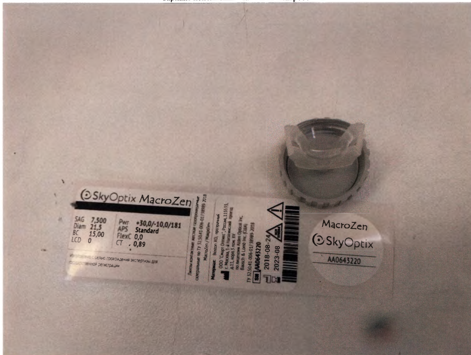
Рисунок 6. Общий вид и маркировка линзы контактные жесткие газопроницаемые склеральные по ТУ 32.50.41-006-01738989-2018, вариант исполнения MacroZen/ МакроЗен
