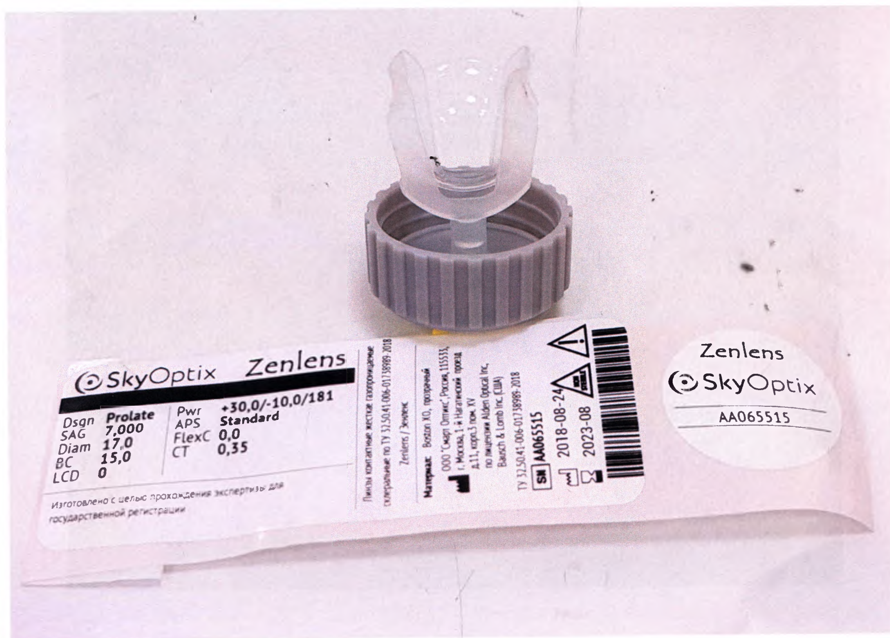
Рисунок 2. Общий вид линзы контактные жесткие газопроницаемые склеральные по ТУ 32.50.41-006-01738989-2018, вариант исполнения Zenlens / Зенленс
