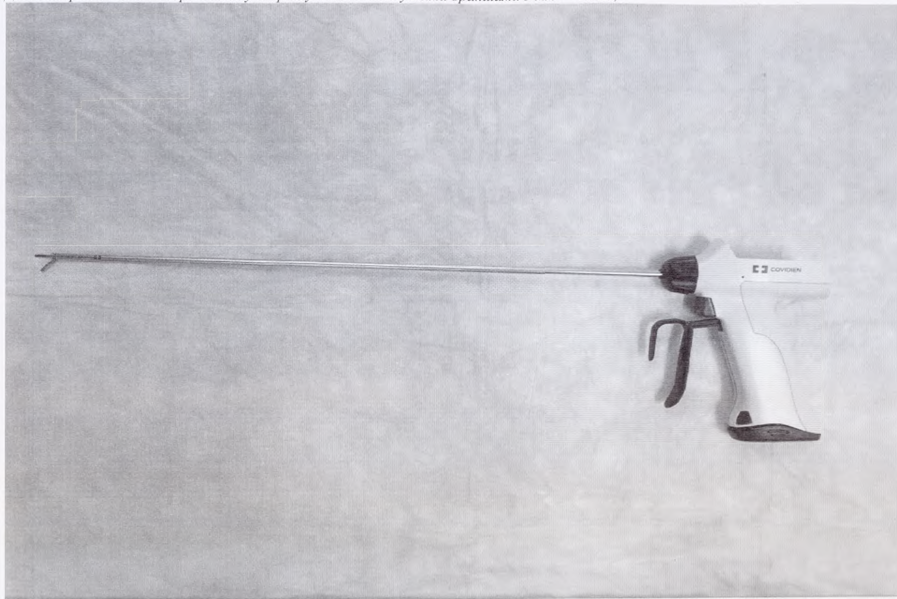
Диссектор Sonicision беспроводной ультразвуковой с изогнутыми браншами 5 мм — 48 см;
