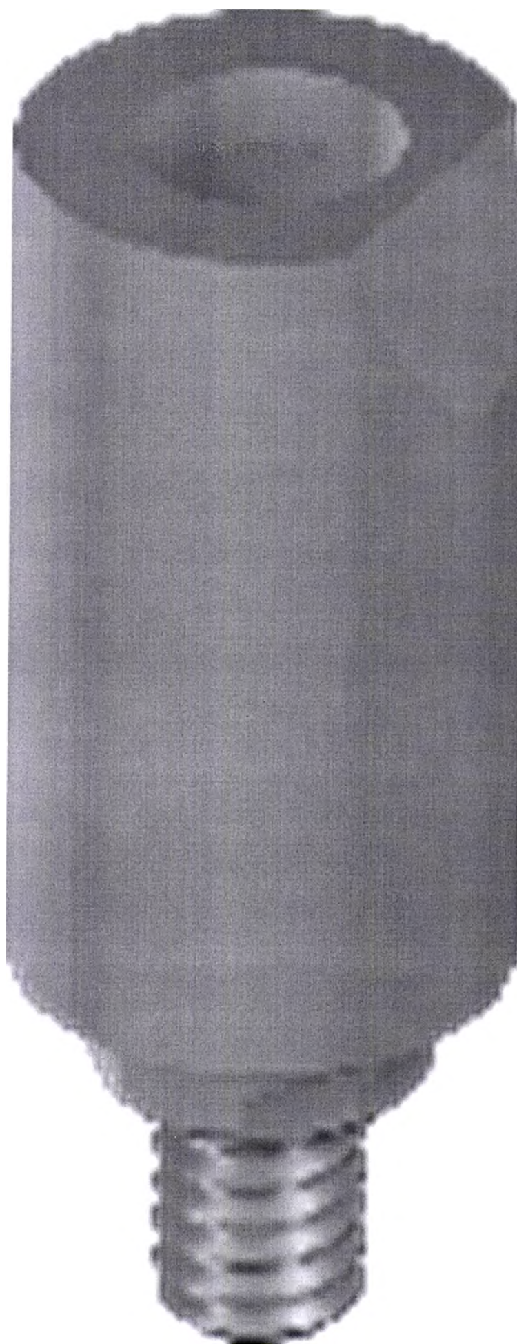
1.55. CARES RN Mono Scanbody, D 4.8 mm, H 10 mm, артикульный номер 048.168
