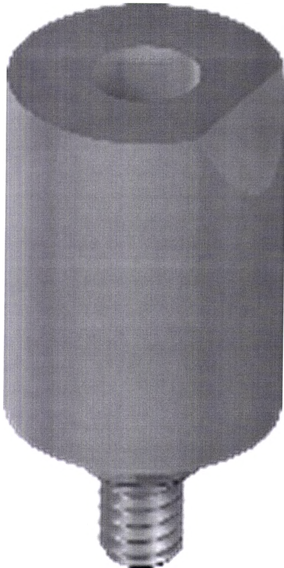
1.56. CARES WN Mono Scanbody, D 6.5 mm, H 10 mm, артикульный номер 048.169
