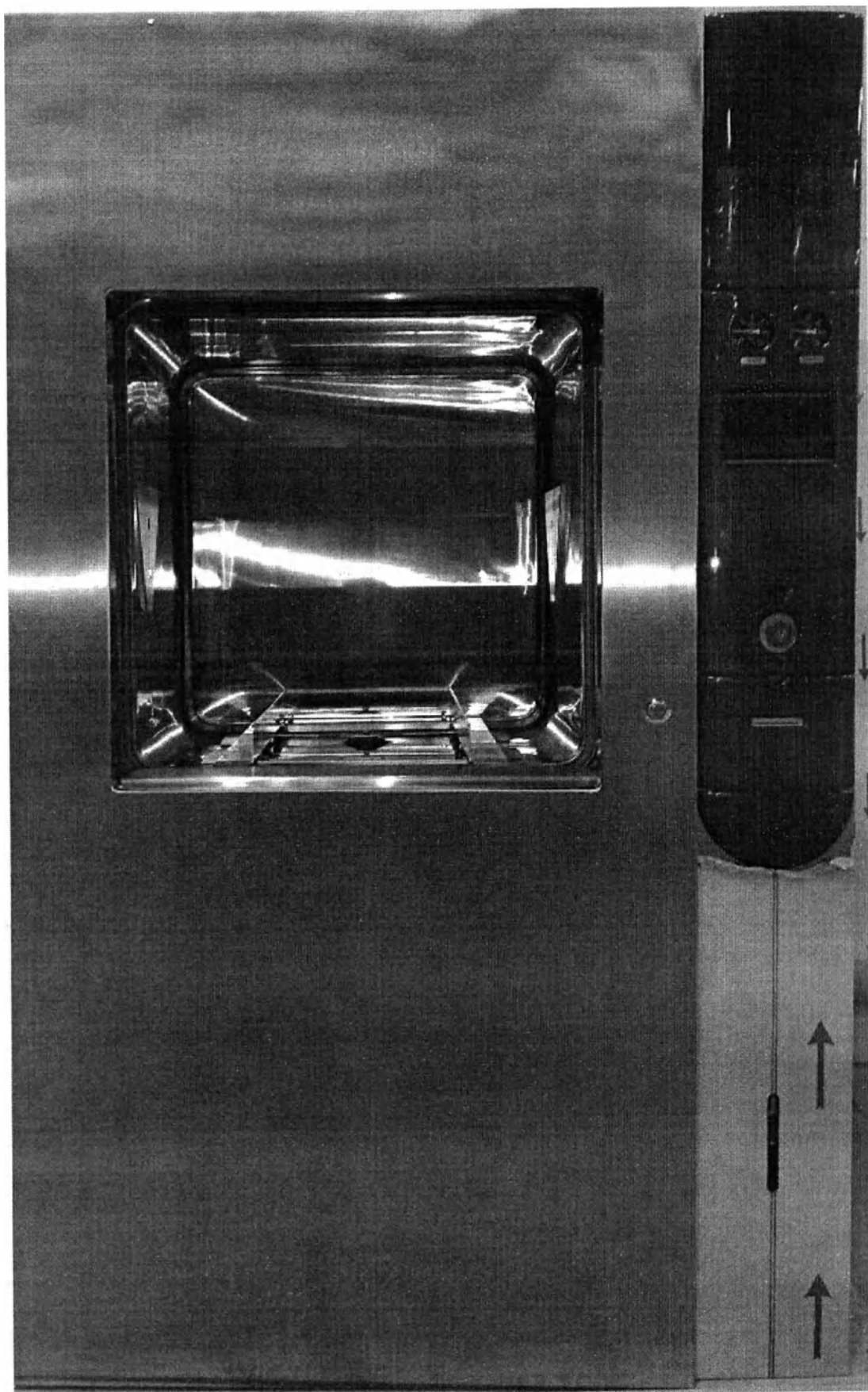
Стерилизатор паровой для обеззараживания медицинских отходов СМО-560 "ТЗМОИ".
