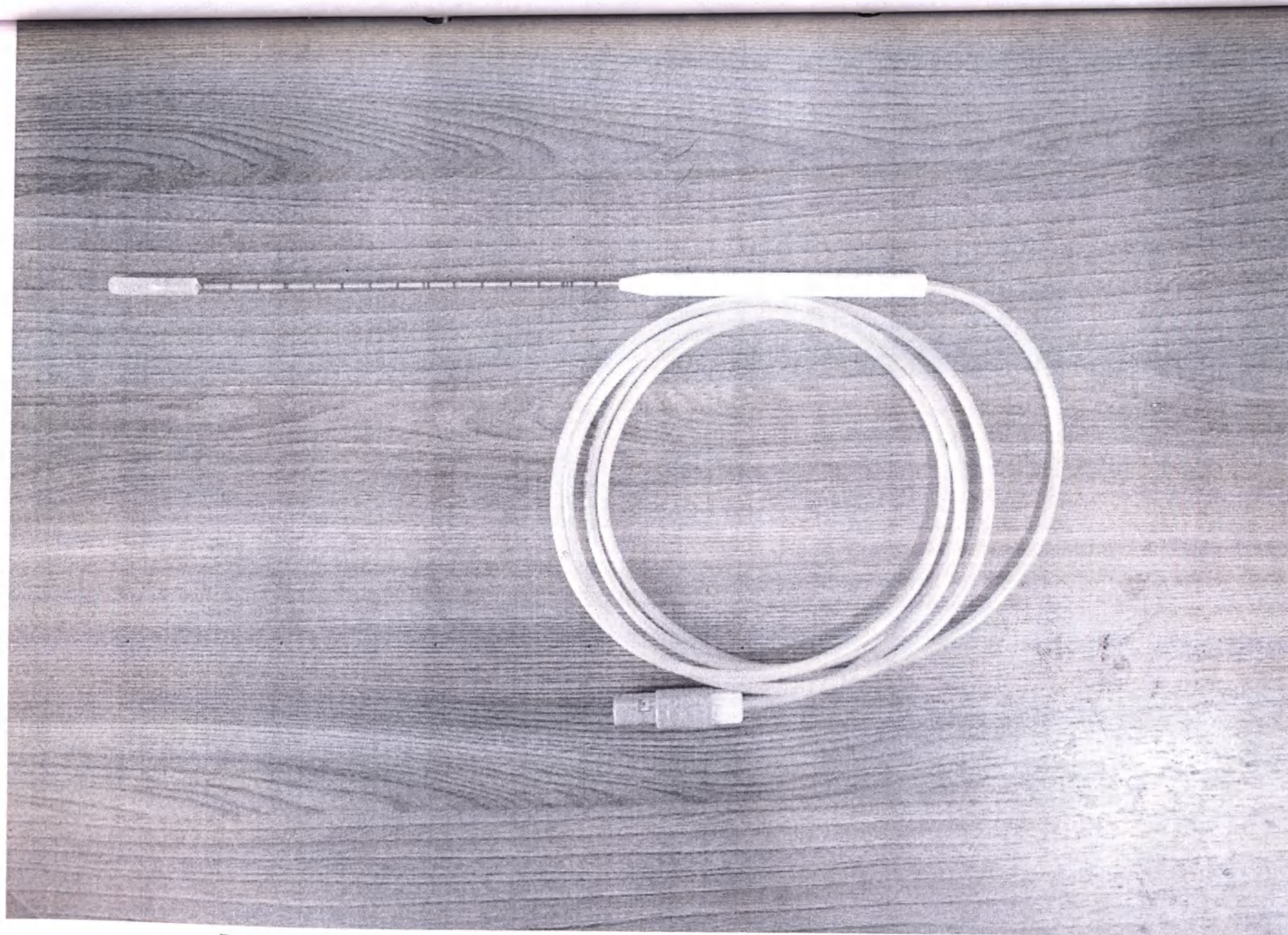
Рис. 4. Датчик температуры (FAT8000000): длина 200 мм, диаметр 2,0 мм, тип «троакар»
