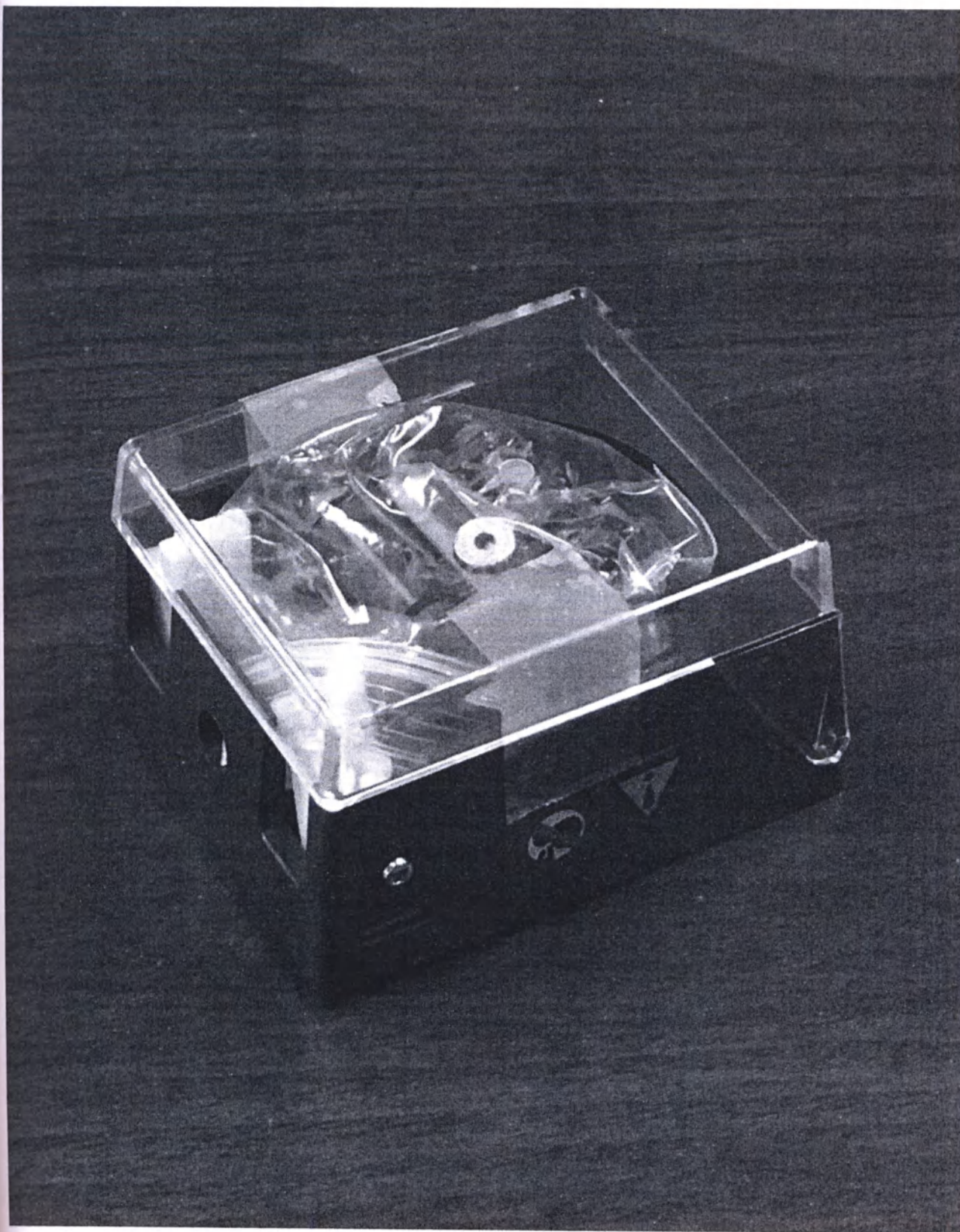
Ролик перистальтического насоса.
