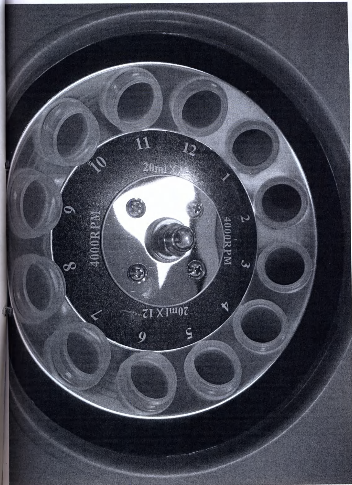
Рис. 8 – Маркировка ротора
