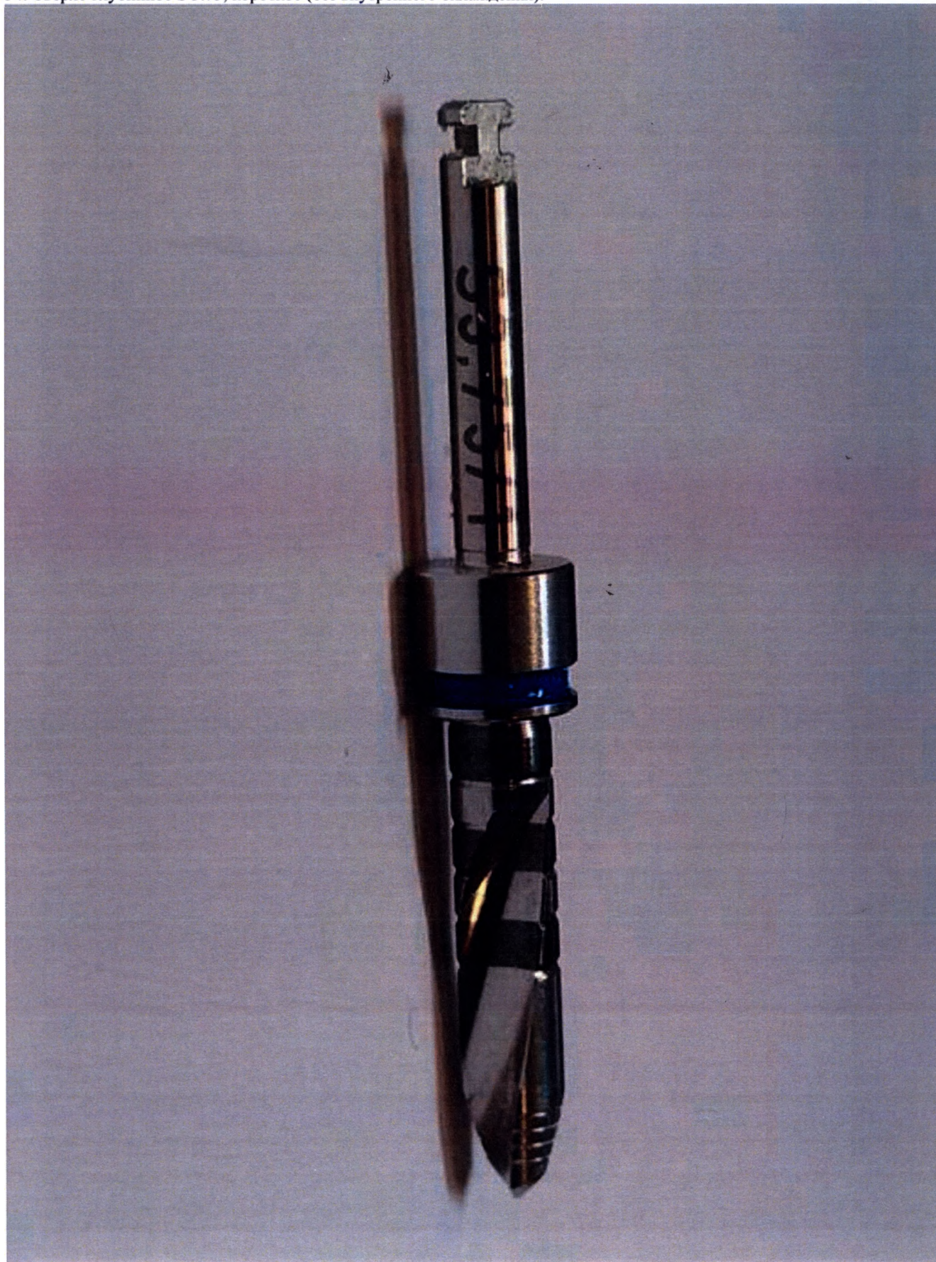
34. Сверло глубинное S 3.75, короткое (без внутреннего охлаждения).
