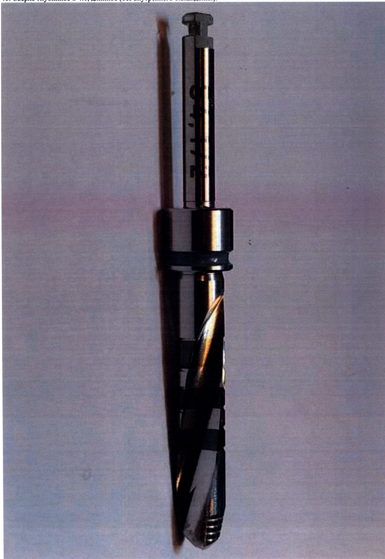
40. Сверло глубинное S 4.1, длинное (без внутреннего охлаждения).
