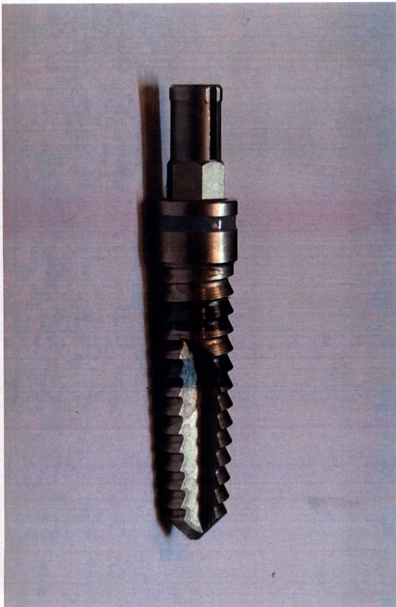
135. Метчик, нарезающий резьбу RI 4.1.
