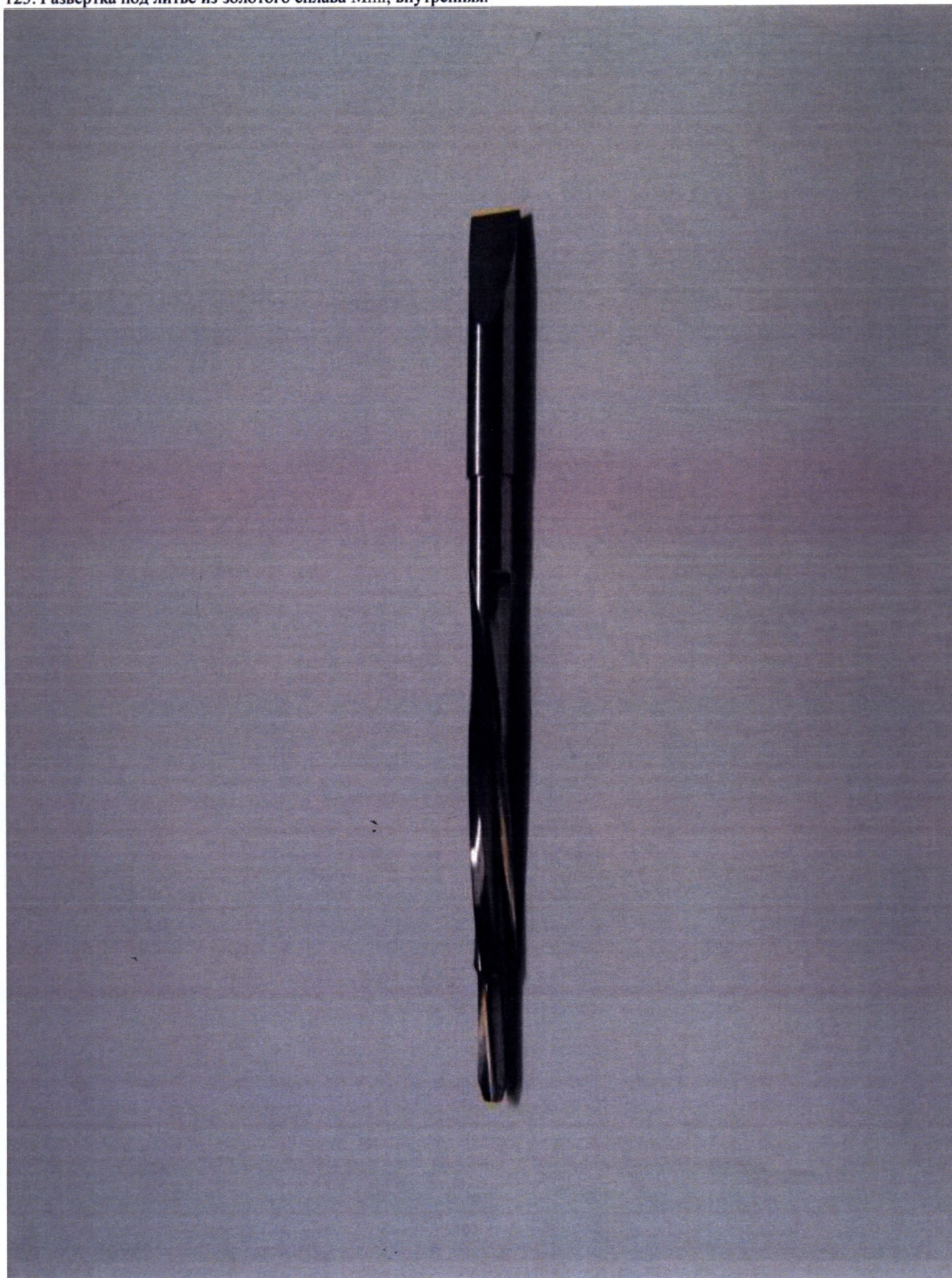
123. Развертка под литье из золотого сплава Mini, внутренняя.
