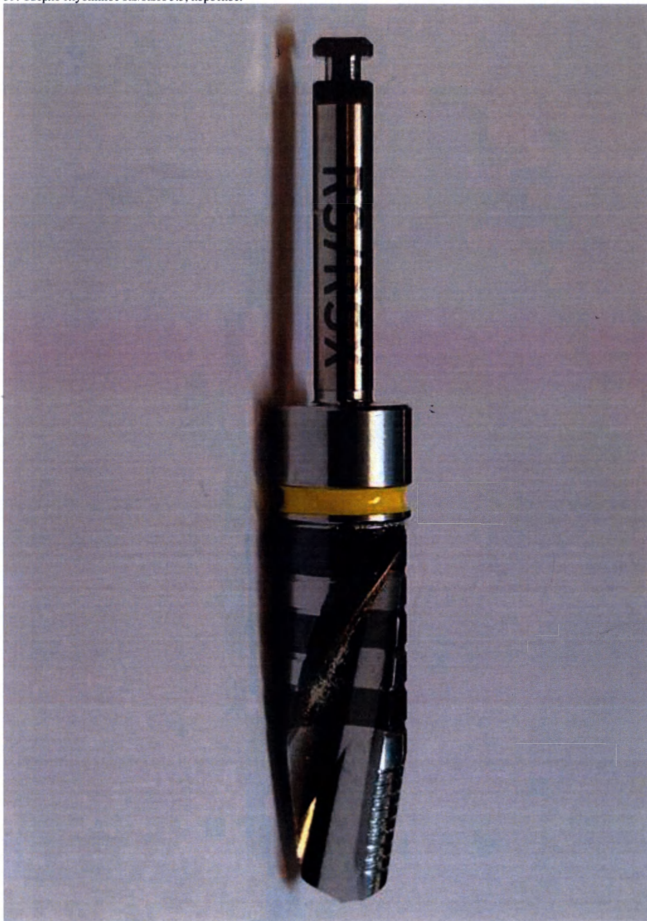
59. Сверло глубинное RS/RX 5.5, короткое.
