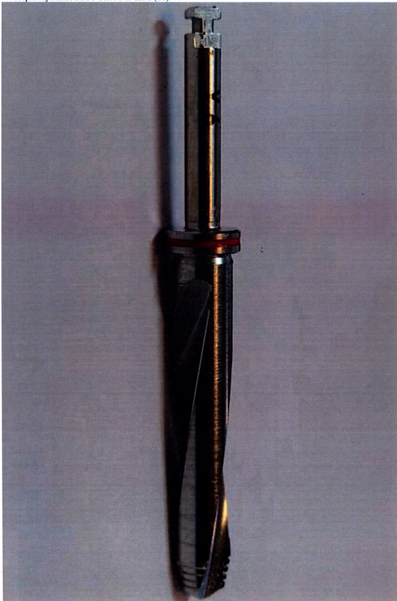
77. Сверло глубинное BEGO Guide S4.5 L23.5 (Y6).
