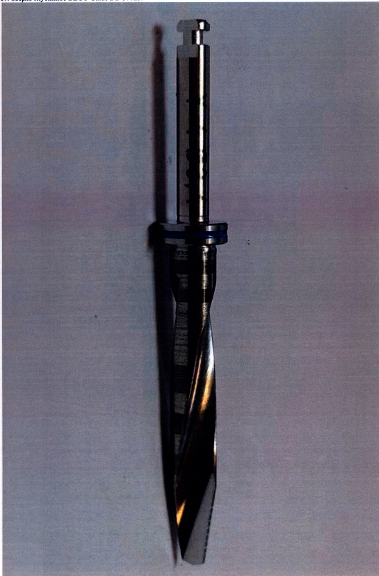
87. Сверло глубинное BEGO Guide DD 57725.
