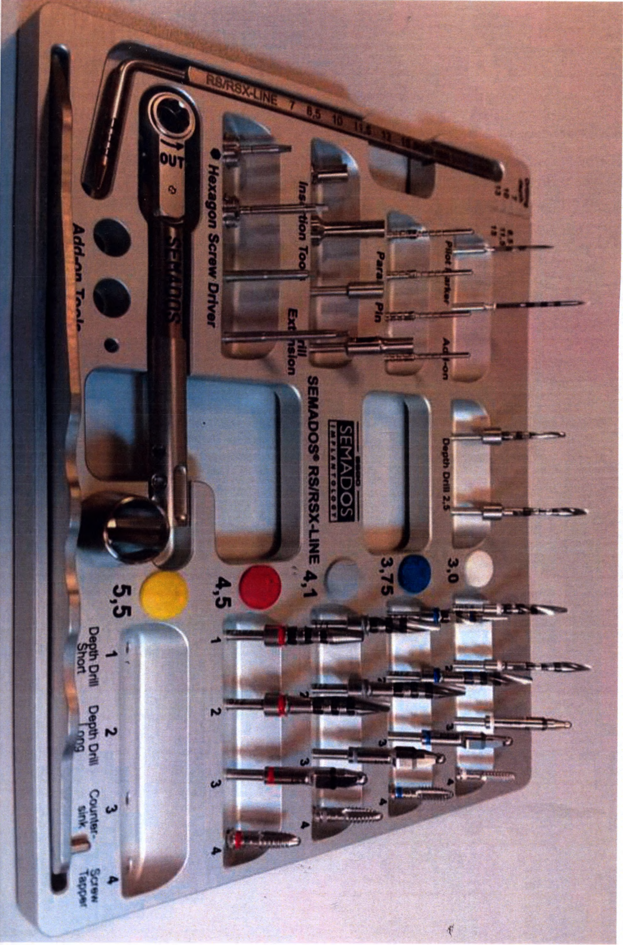
7. Набор BEGO Semados® RS/R SX-LineTray PLUS за исключением набора инструментов RS/R SX 5.5, в контейнере:
