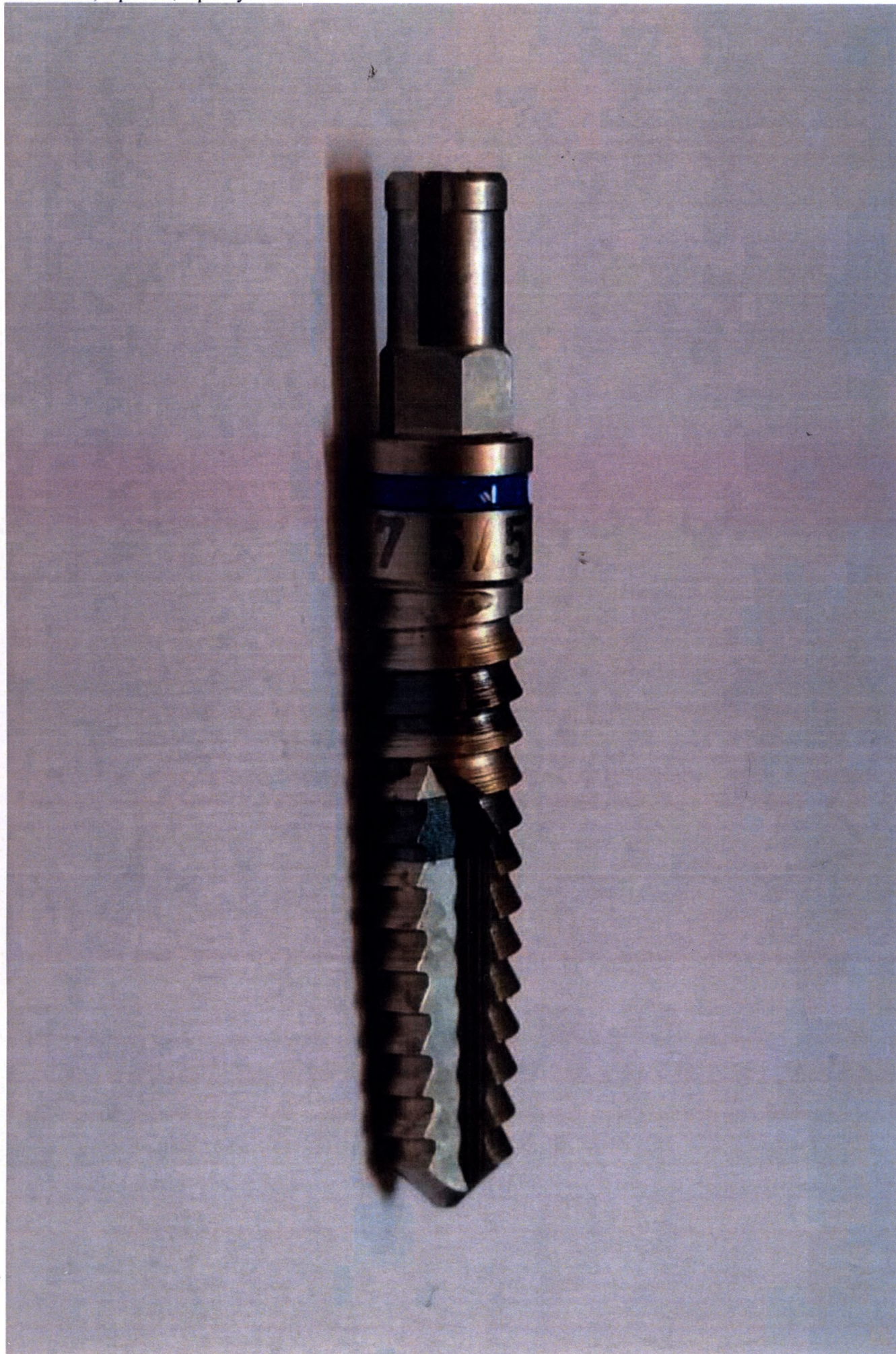
134. Метчик, нарезающий резьбу RI 3.75.
