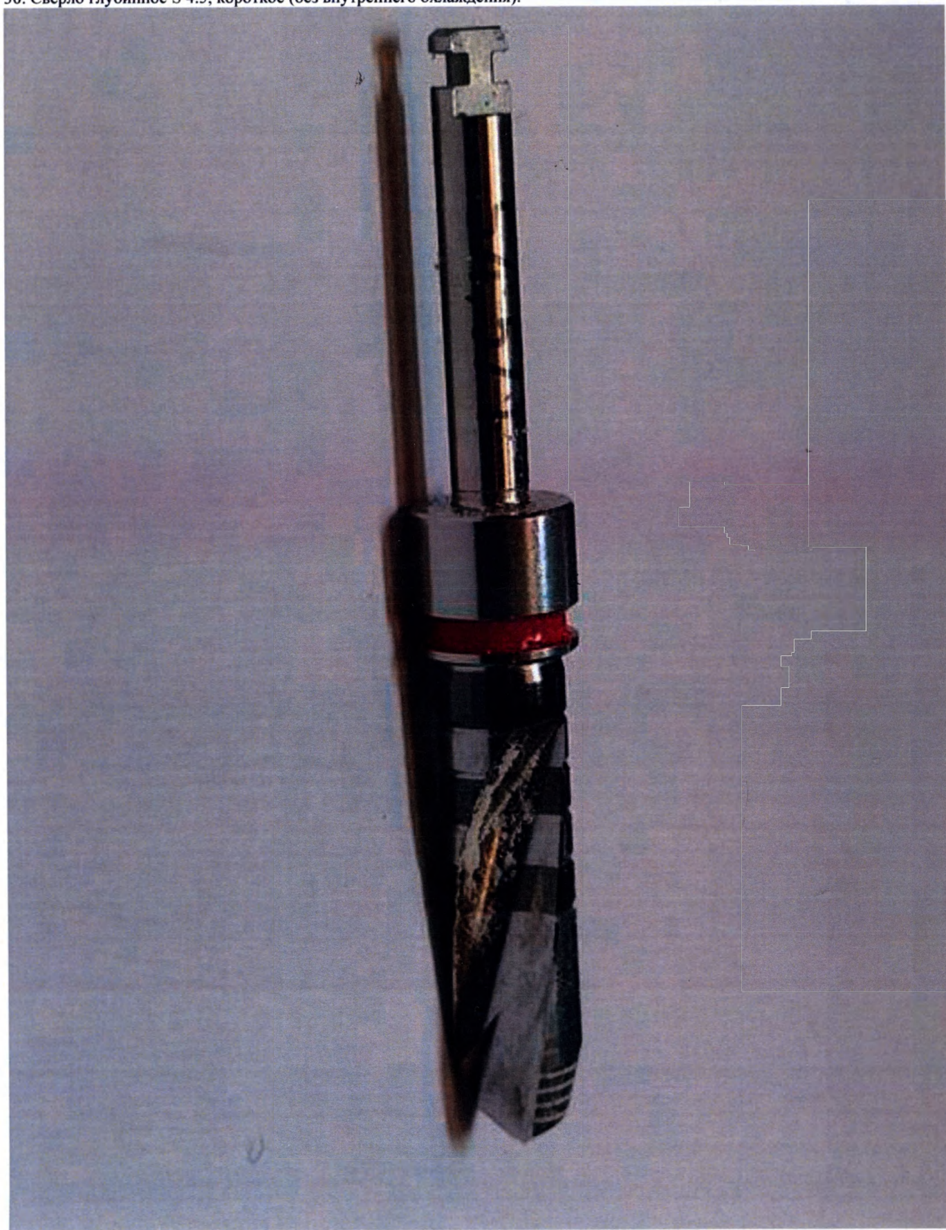
36. Сверло глубинное S 4.5, короткое (без внутреннего охлаждения).
