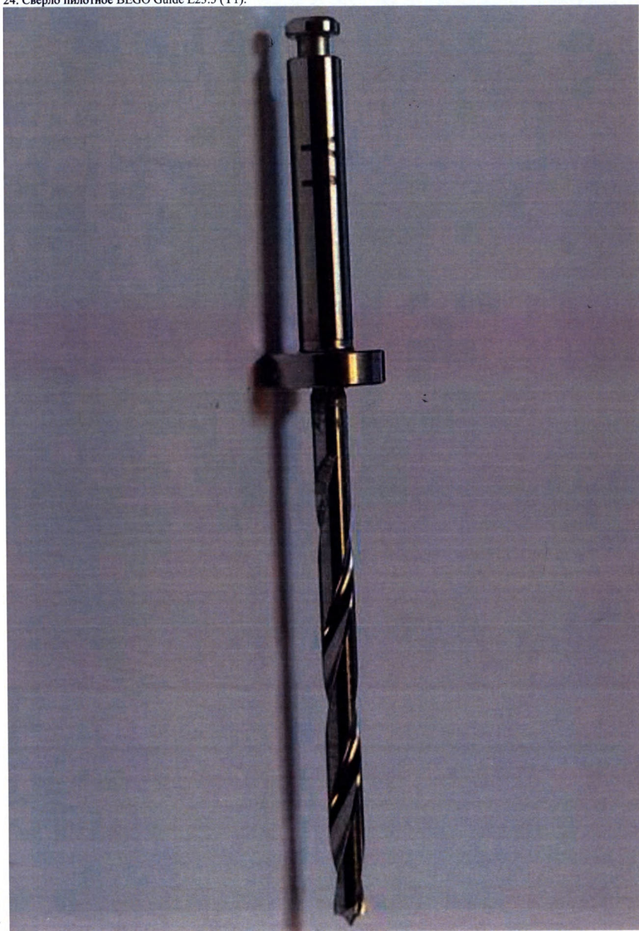
24. Сверло пилотное BEGO Guide L23.5 (Y1).
