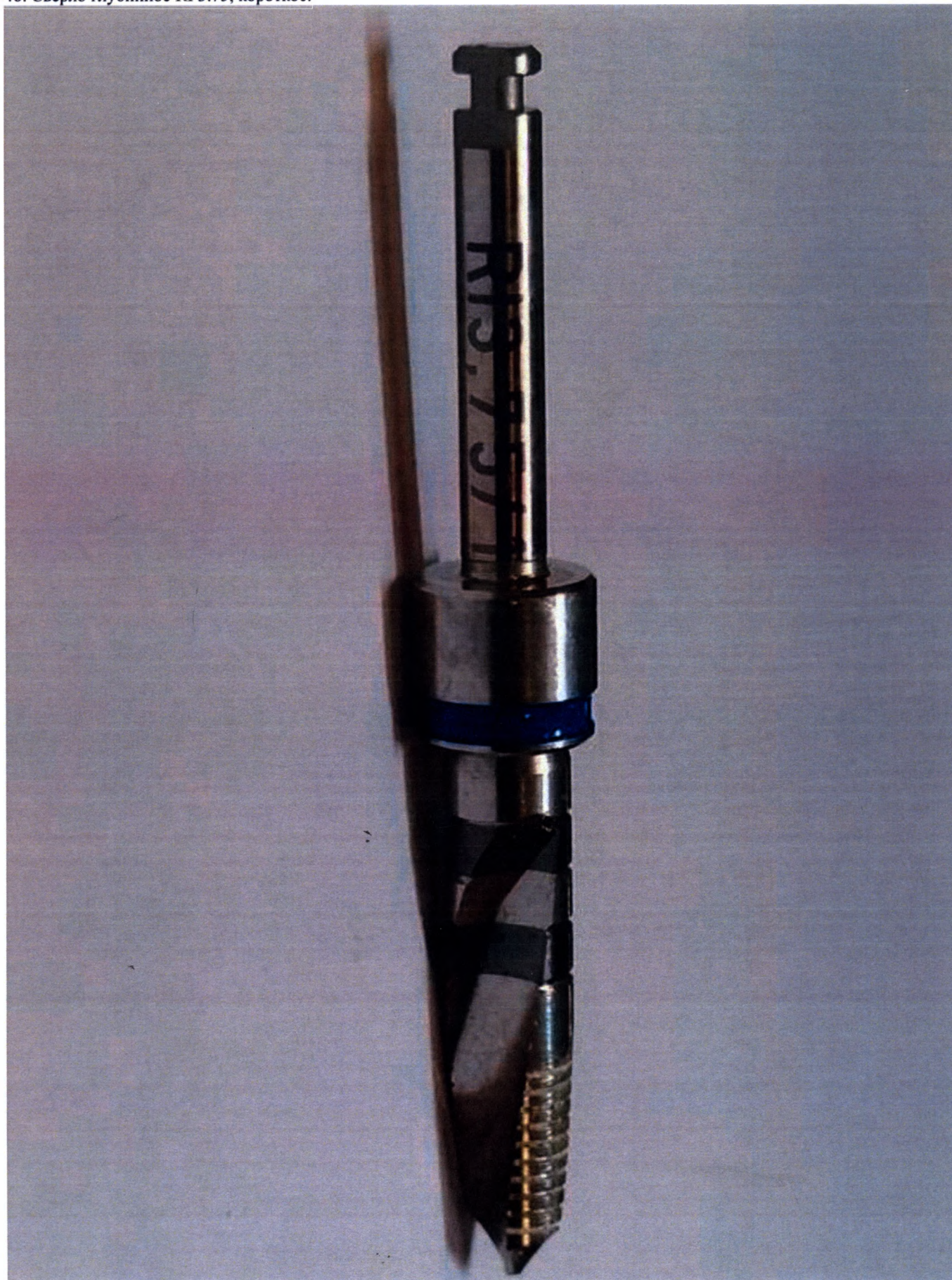
46. Сверло глубинное RI 3.75, короткое.
