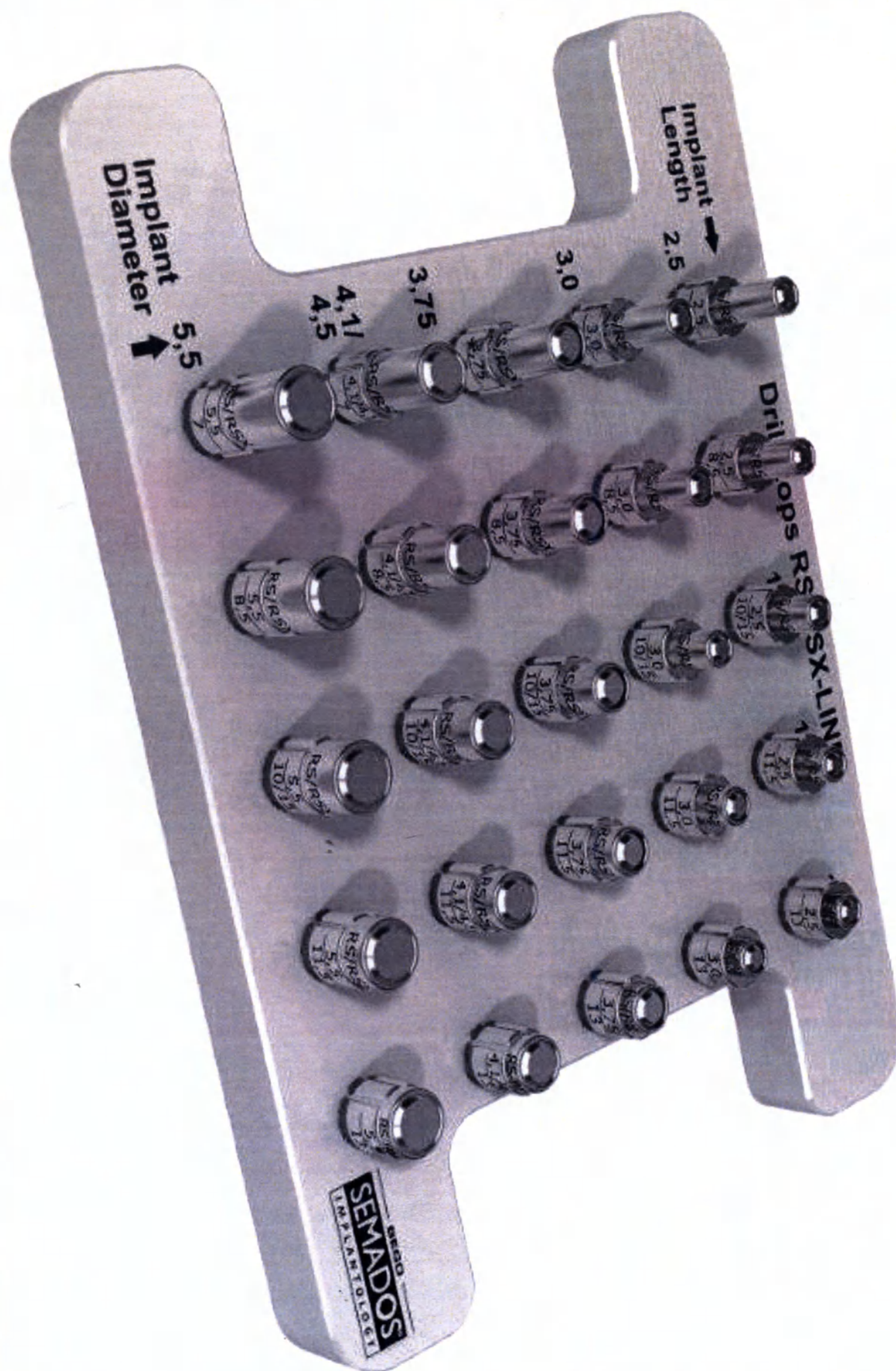
27. Набор ограничителей глубины сверления RS/R SX-LineTray PLUS , в контейнере:
