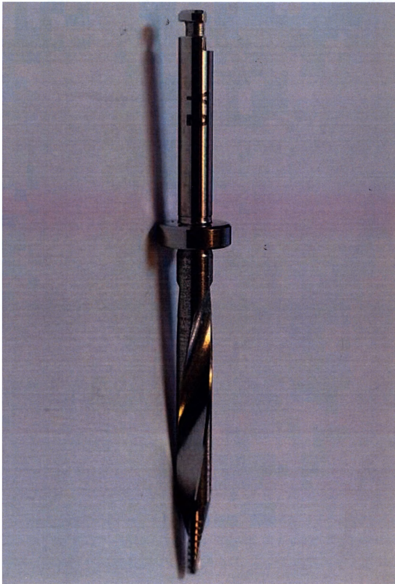
65. Сверло глубинное BEGO Guide 2.5 L23.5 (Y2).
