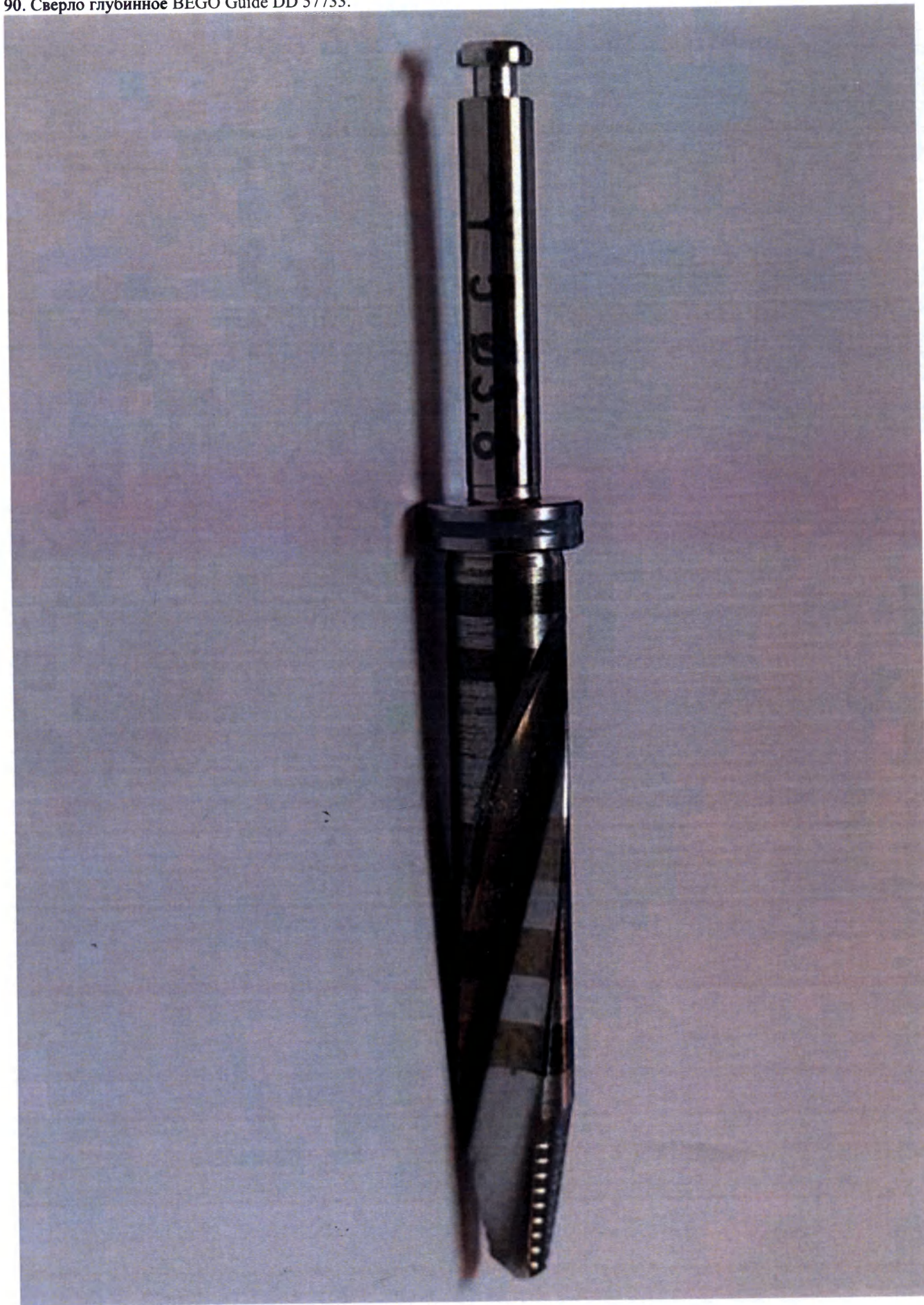
90. Сверло глубинное BEGO Guide DD 57733.
