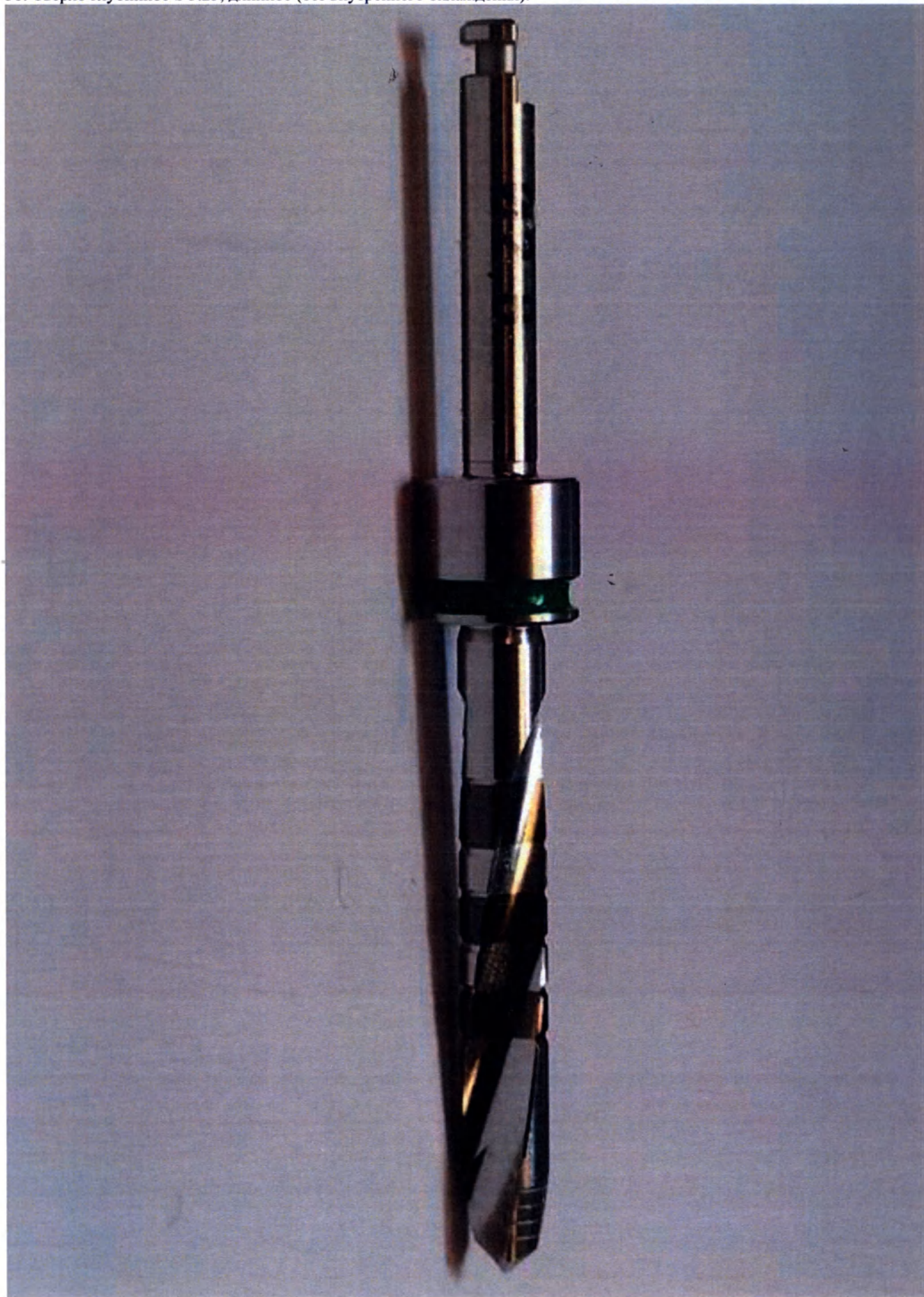
38. Сверло глубинное S 3.25, длинное (без внутреннего охлаждения).
