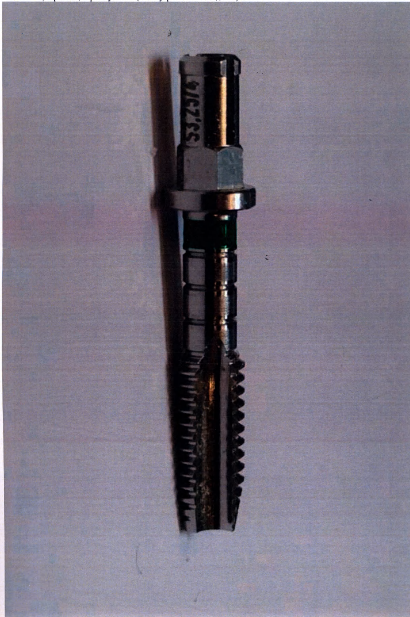
124. Метчик, нарезающий резьбу S 3.25 (без внутреннего охлаждения).
