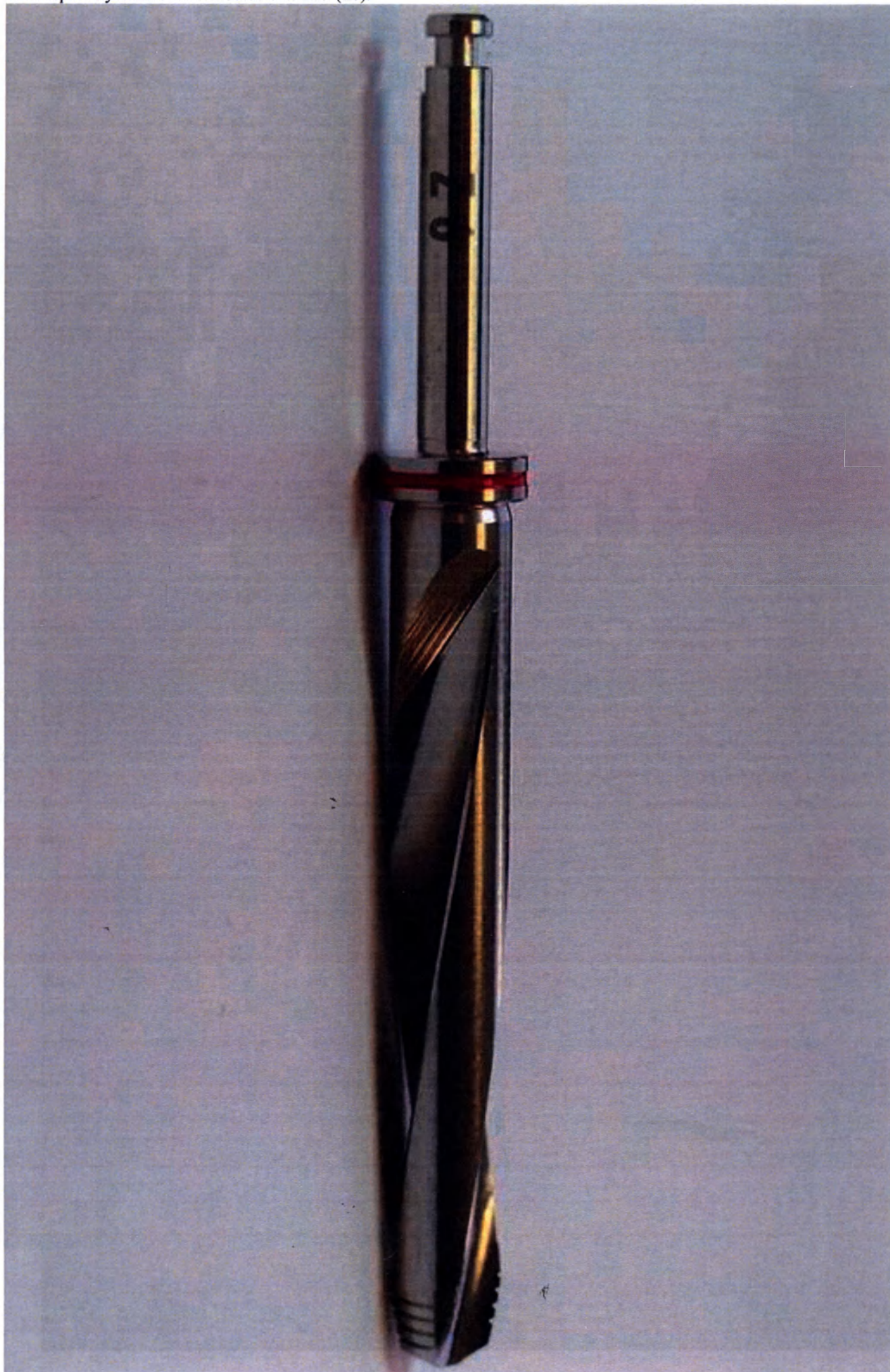
78. Сверло глубинное BEGO Guide S4.5 L29 (Z6).
