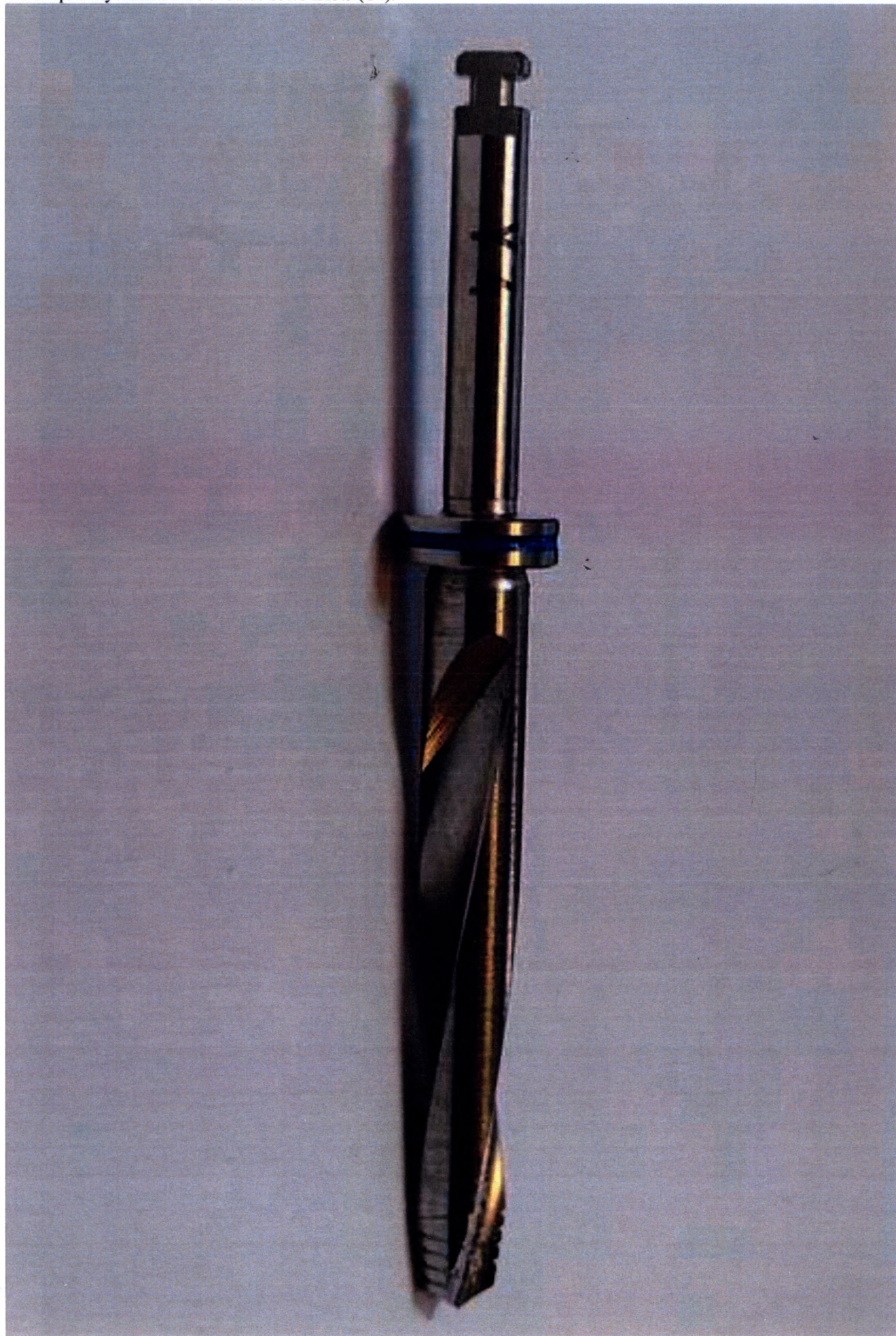
71. Сверло глубинное BEGO Guide S3.75 L23.5 (Y4).
