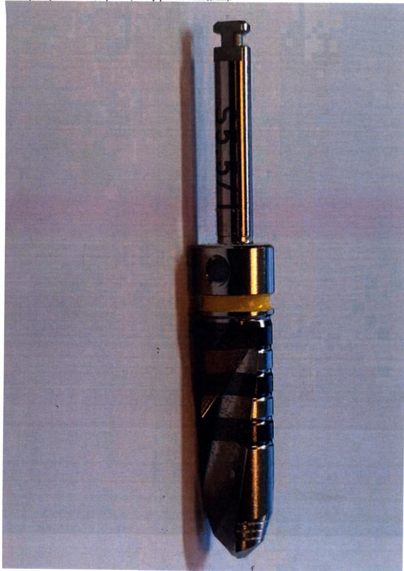
37. Сверло глубинное S 5.5, короткое (без внутреннего охлаждения).
