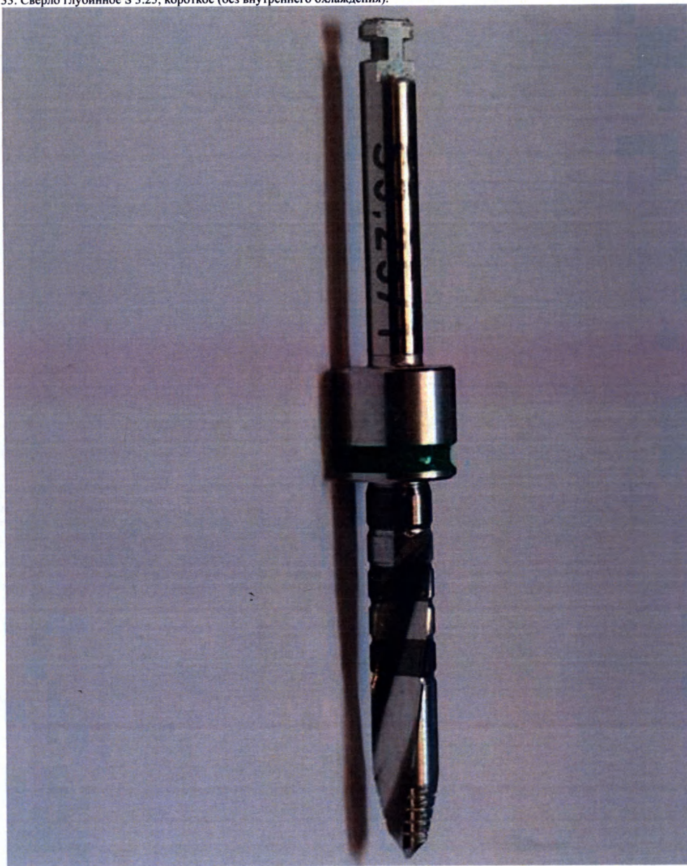
33. Сверло глубинное S 3.25, короткое (без внутреннего охлаждения).
