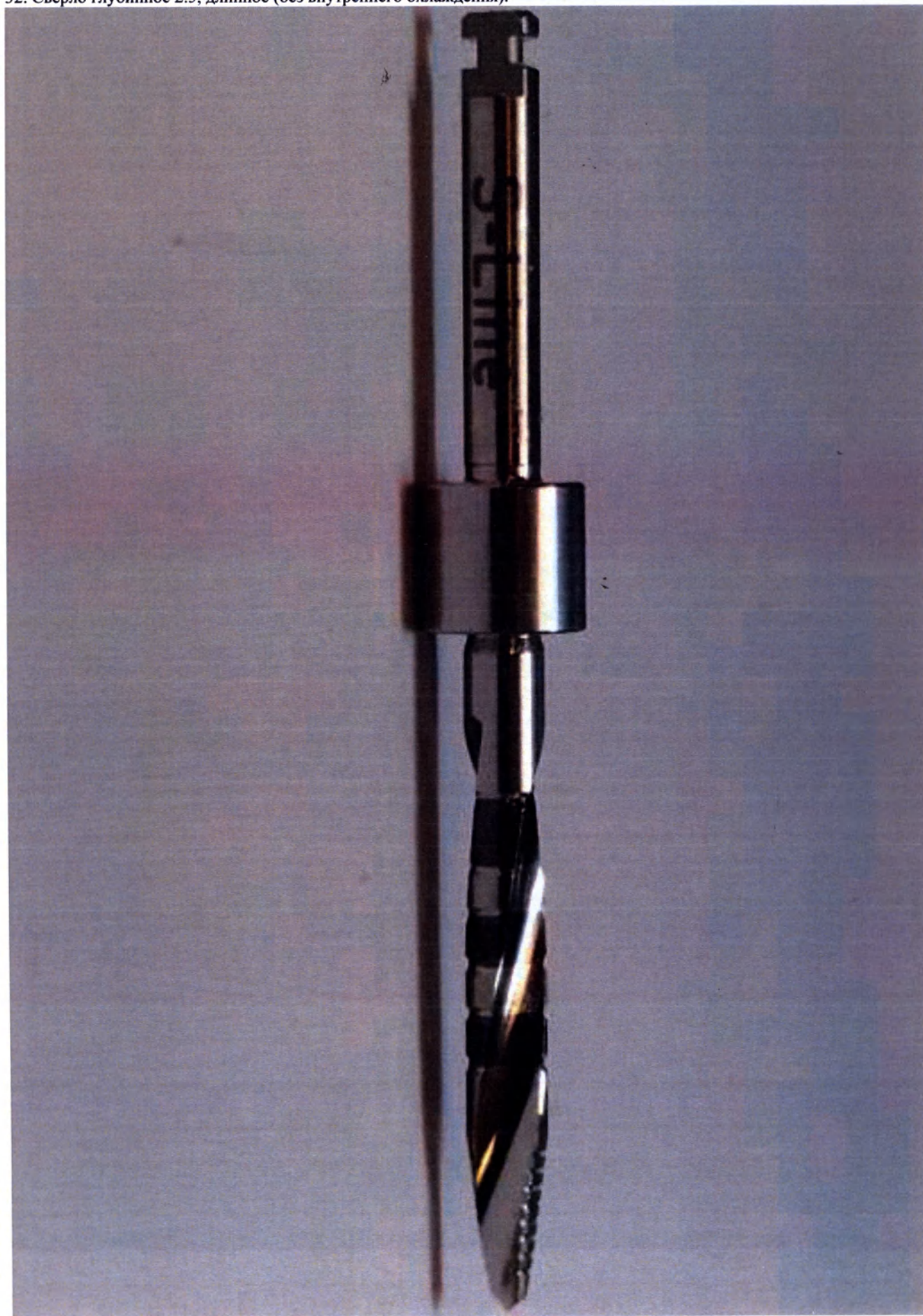
32. Сверло глубинное 2.5, длинное (без внутреннего охлаждения).
