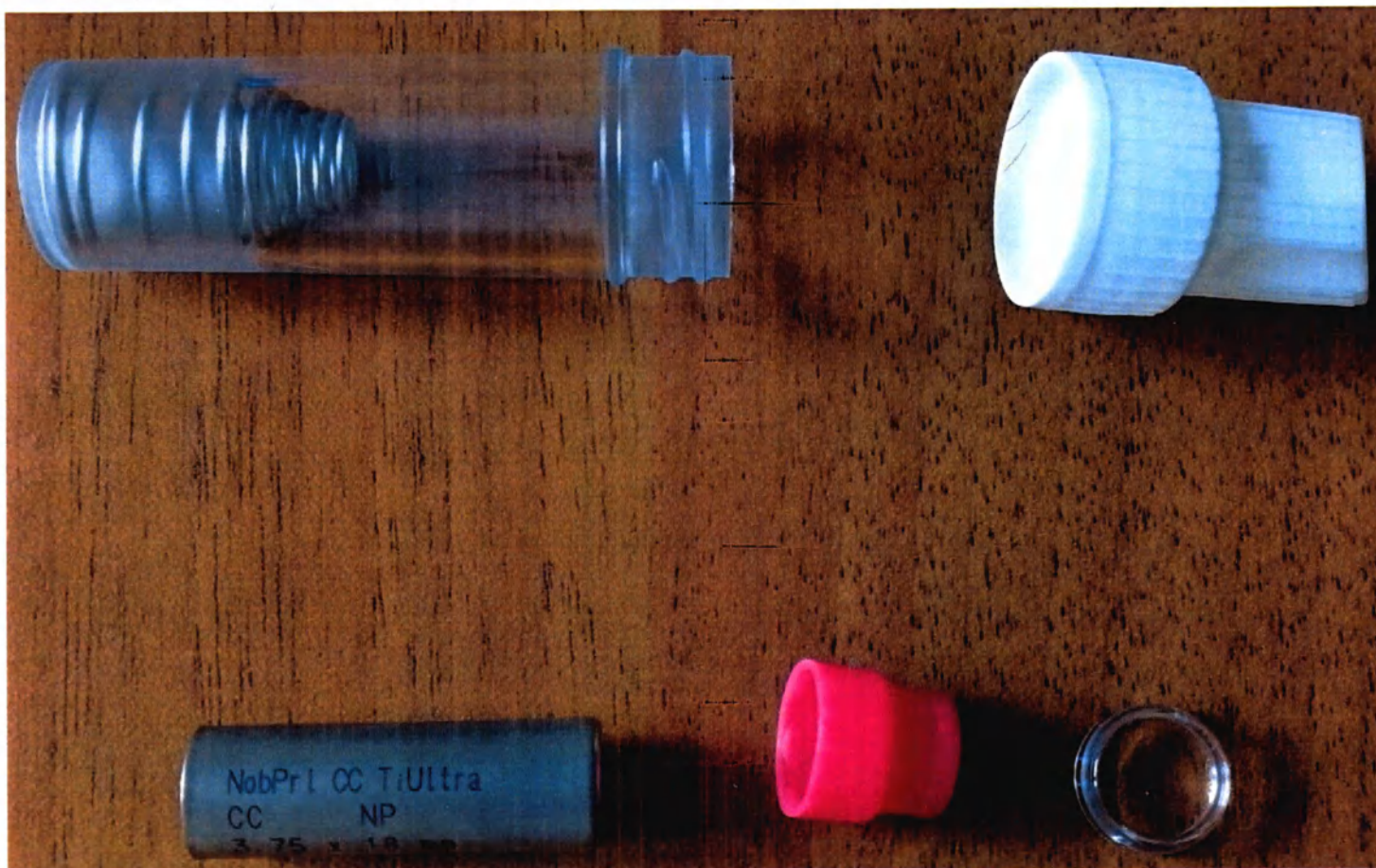
12. Имплантат NobelParallel Conical Connection (CC) TiUltra NP 3.75x18mm. Компоненты упаковки.
