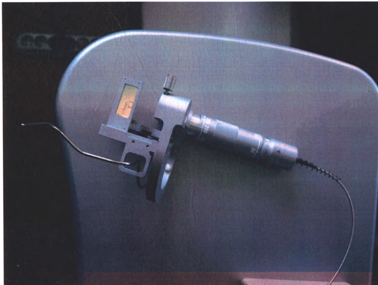
Рисунок 12 – Адаптер.
