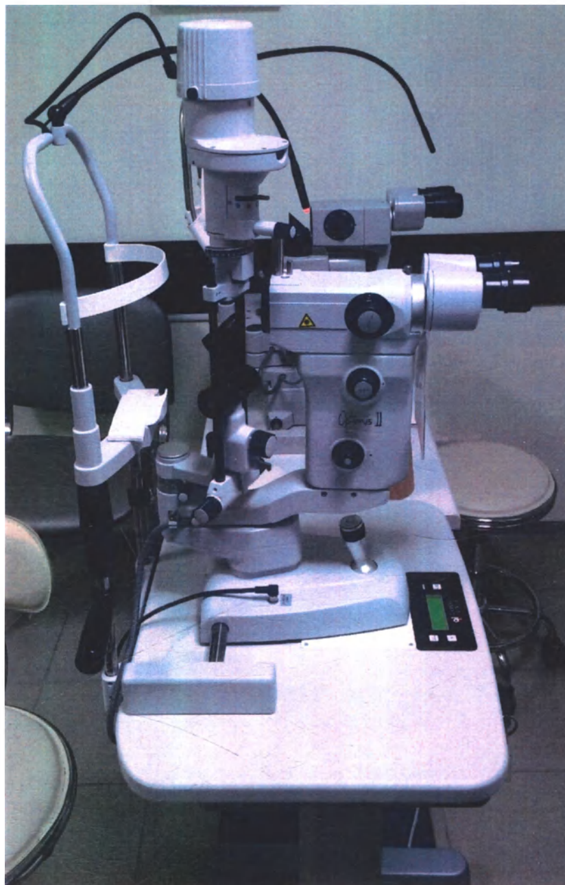
Рисунок 1 – Система офтальмологическая лазерная OPTIMIS II с лампой щелевой модели SL 9900.
