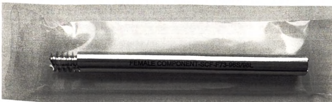
Рисунок 8 – Компонент с внутренней резьбой 96/98 мм Ø7,3 мм, SCF-F73-96S/98L
