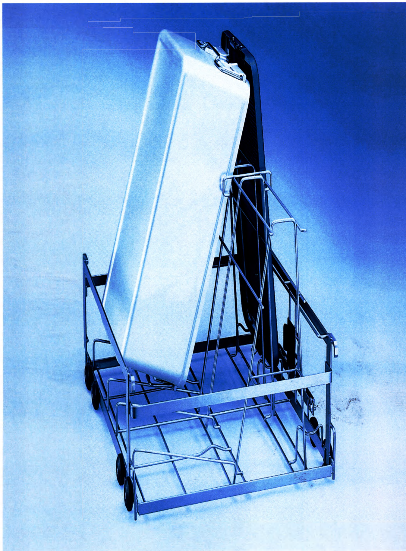
Тележка Е 711/1 для размещения вставок и контейнеров, а также медицинских инструментов и лабораторного стекла для автоматов для мойки и дезинфекции G 7825, G 7826
