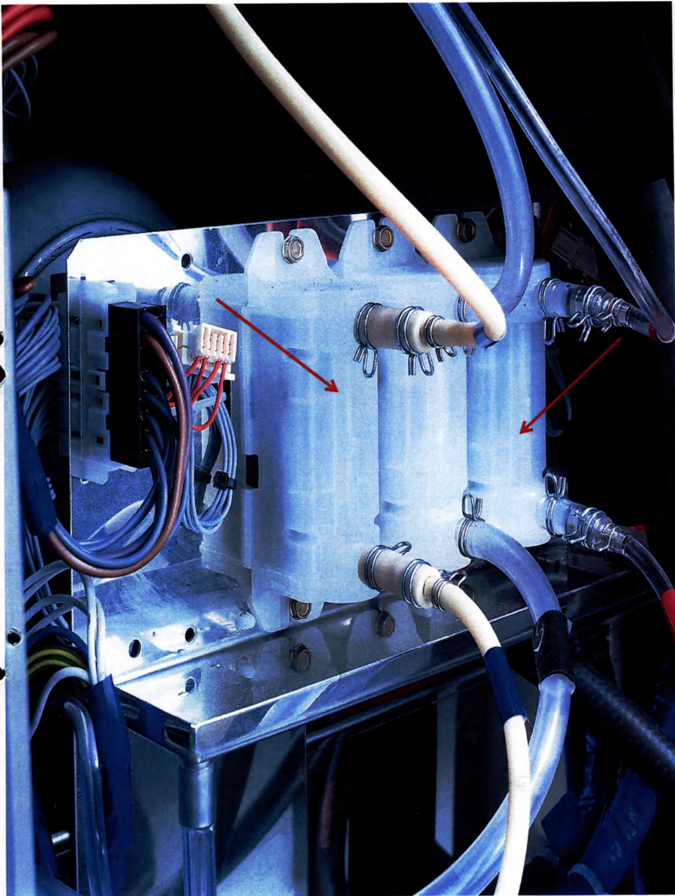
Системы дозирования жидких сред DOS 10/30 и DOS 60/30 для автоматов для мойки и дезинфекции G 7823, G 7824, G 7825, G 7826
