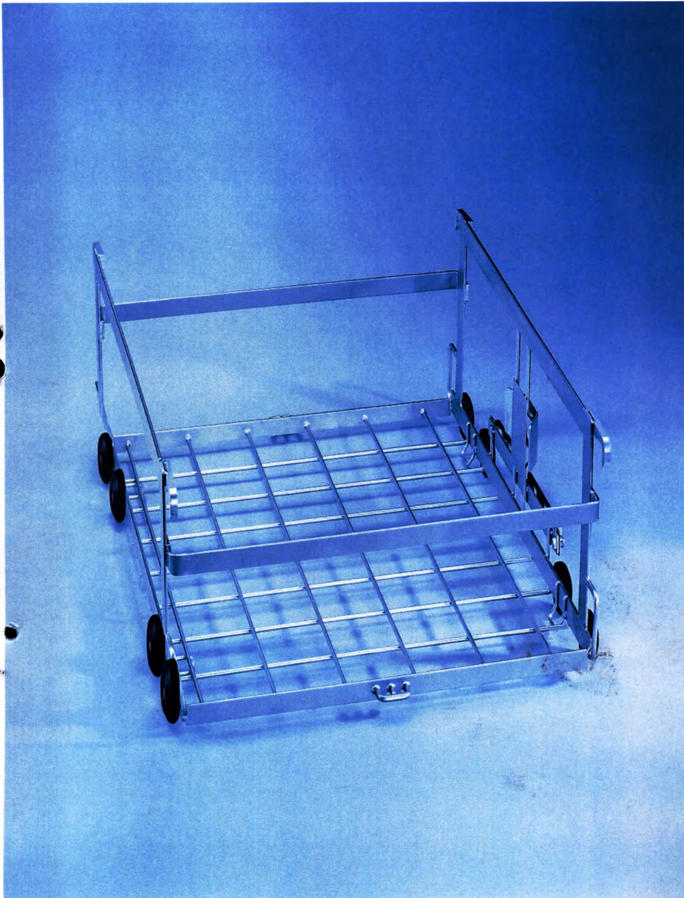
Вставка Е 550 для размещения медицинского инструмента для автоматов для мойки и дезинфекции G 7823, G 7824
