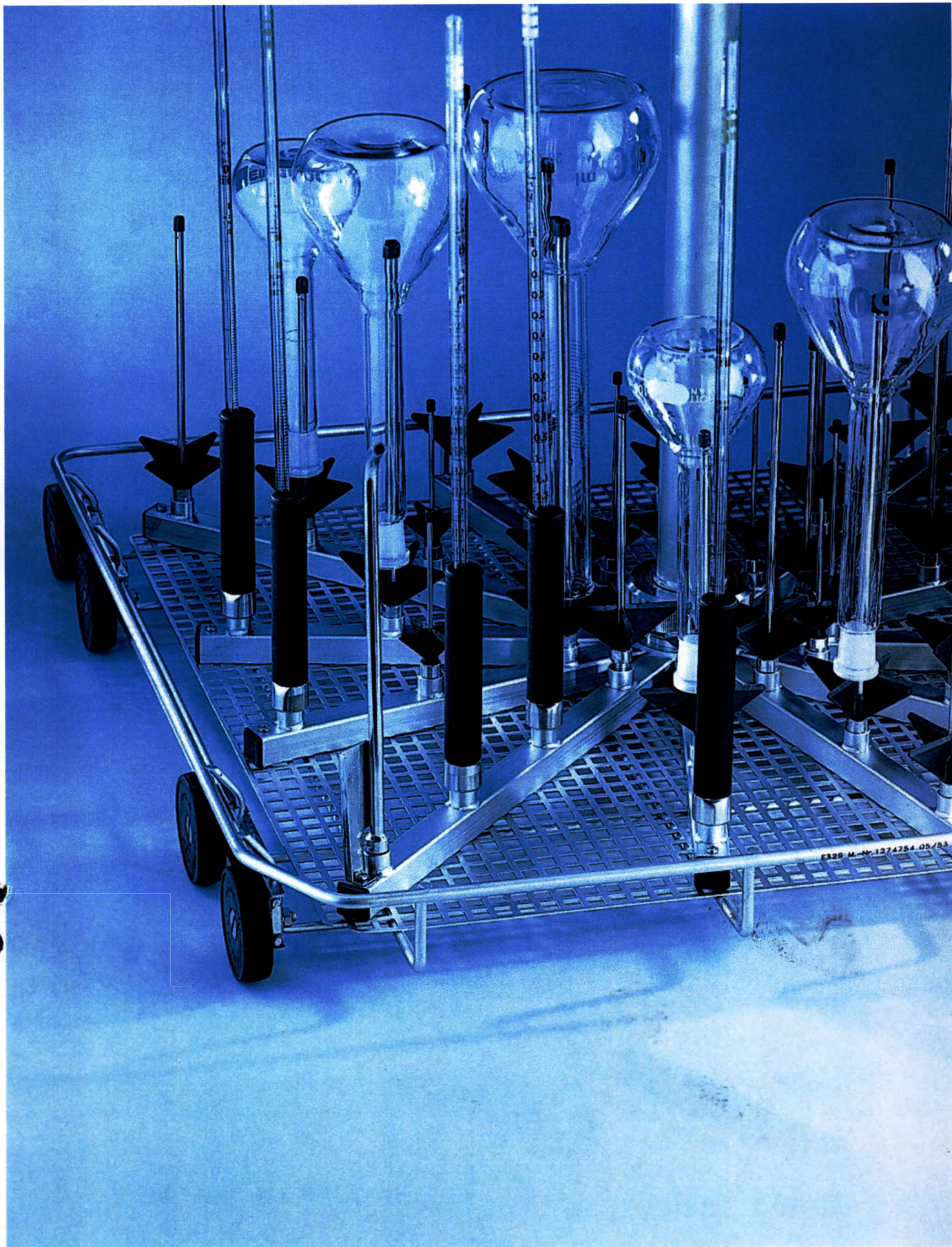
Вставка Е 336 для размещения медицинского инструмента и лабораторного стекла для автоматов для мойки и дезинфекции G 7823, G 7824, G 7825, G 7826, G 7882, G 7882 CD, G 7883, G 7883 CD
