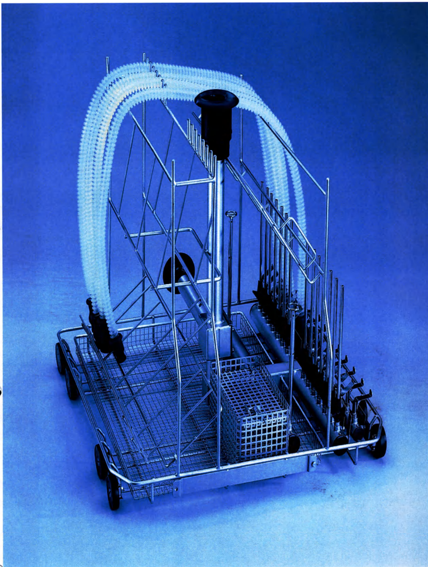
Тележка Е 368 для размещения вставок, контейнеров и специальных медицинских инструментов для автоматов для мойки и дезинфекции G 7882, G 7882 CD
