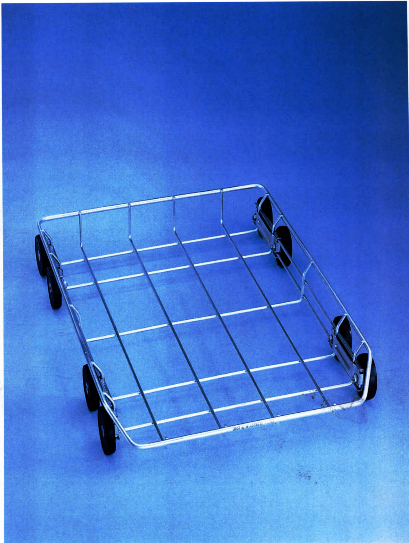
Корзина U 800 для размещения вставок, контейнеров и специальных медицинских и стоматологических инструментов для автоматов для мойки и дезинфекции G 7831, G 7881, G 7882, G 7882 CD
