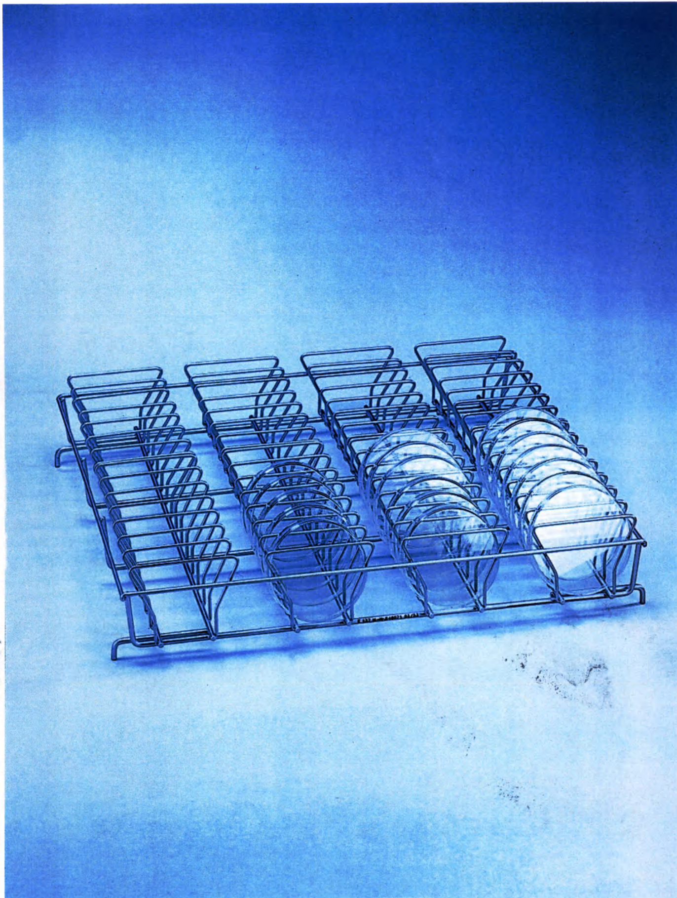
Вставка Е 137 для размещения медицинского инструмента и лабораторного стекла для автоматов для мойки и дезинфекции G 7825, G 7826, G 7883, G 7883 CD
