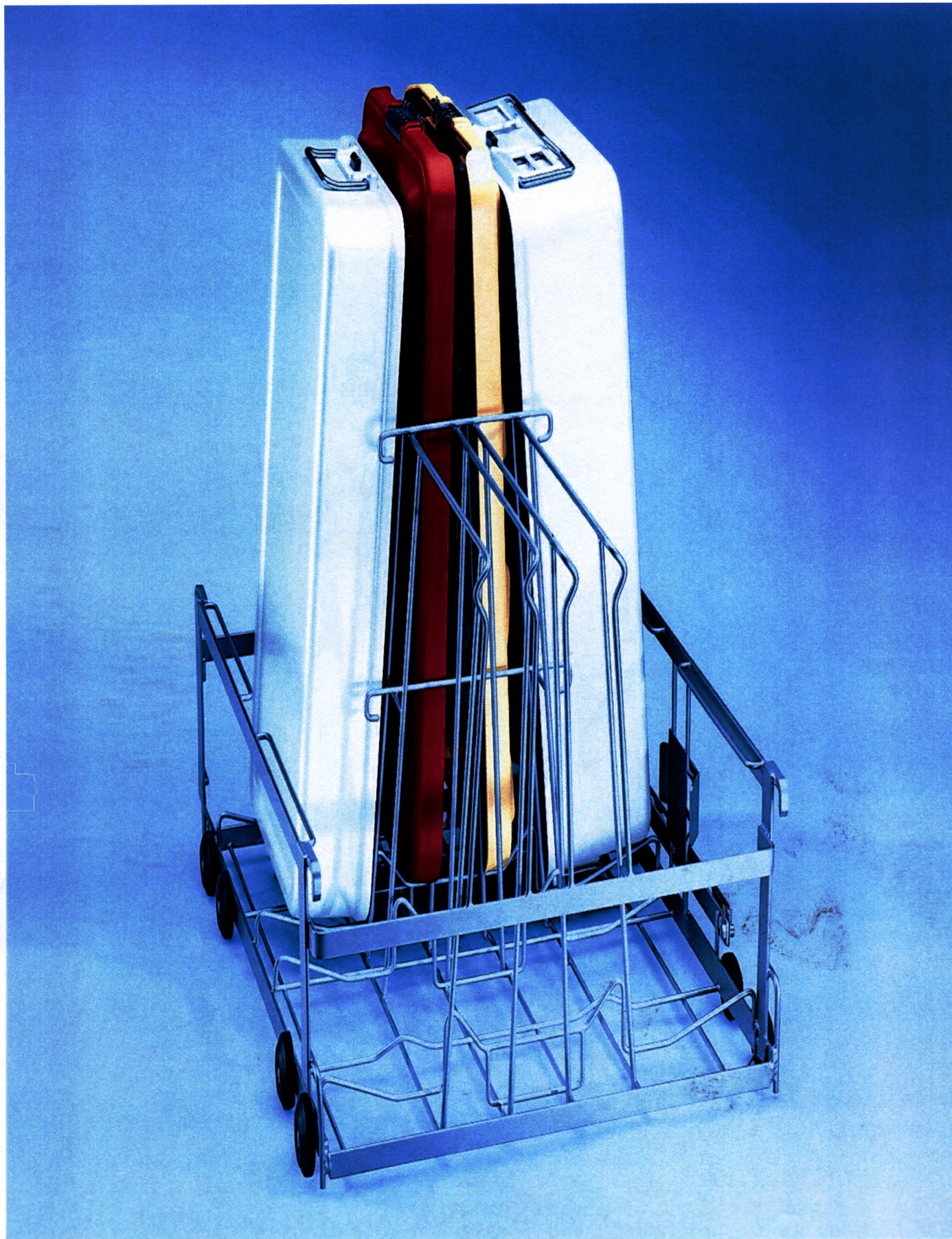
Тележка Е 710/1 для размещения вставок и контейнеров, а также медицинских инструментов и лабораторного стекла для автоматов для мойки и дезинфекции G 7825, G 7826
