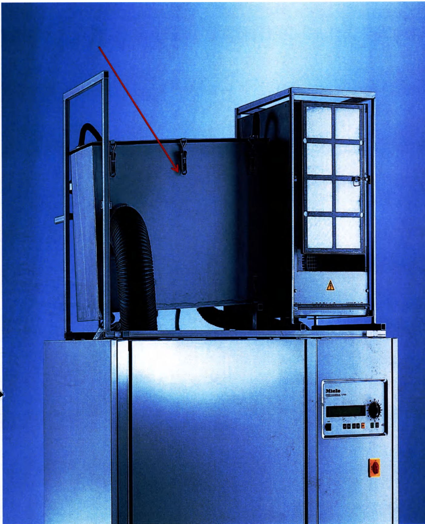
Системы конденсации пара DK 25/26 для автоматов для мойки и дезинфекции G 7825, G 7826
