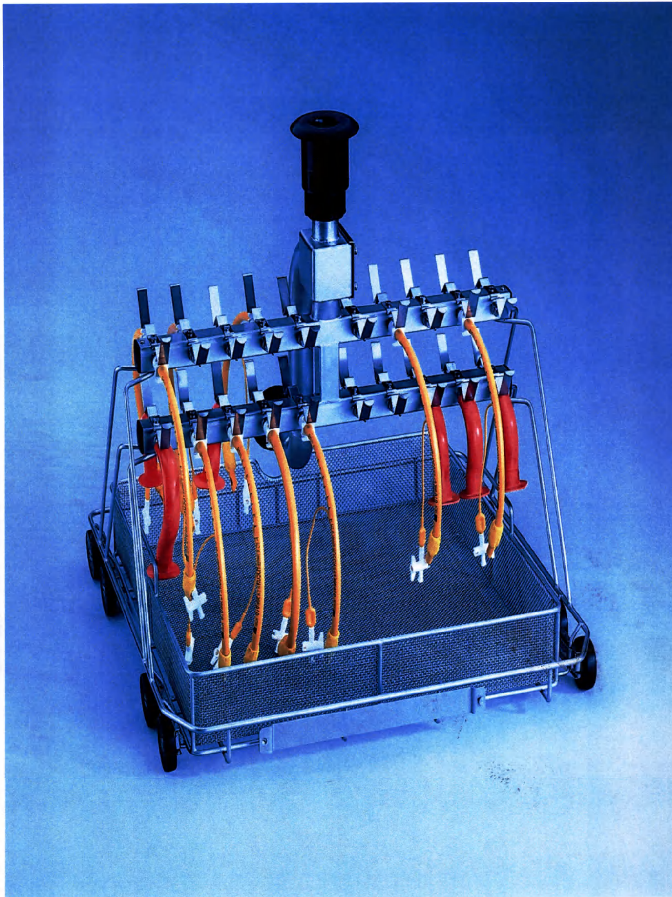
Тележка Е 367 для размещения вставок, контейнеров и специальных медицинских инструментов для автоматов для мойки и дезинфекции G 7882, G 7882 CD
