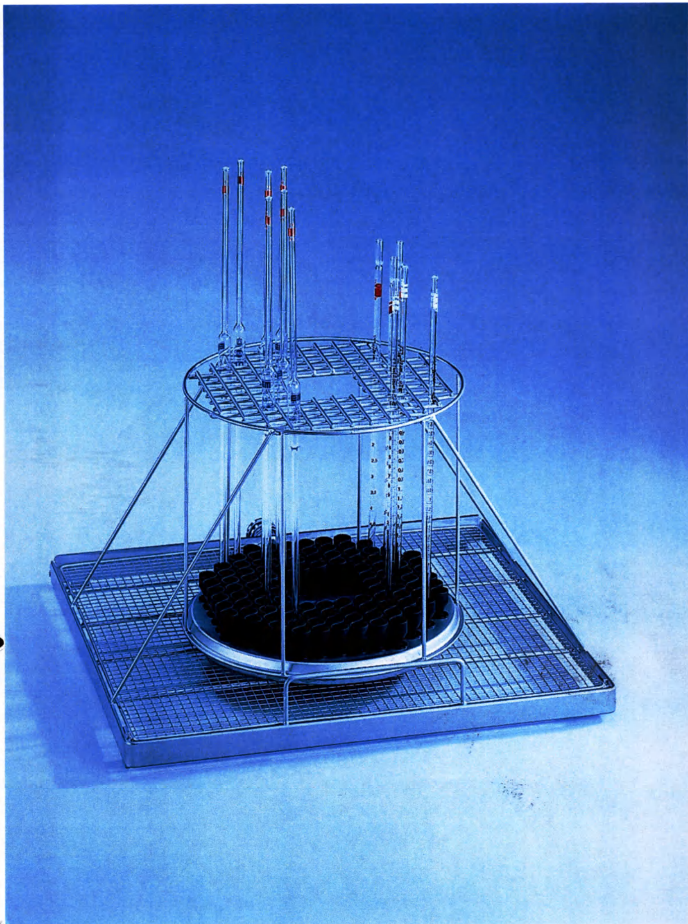
Модуль-вставка Е 745/1 для размещения медицинского инструмента и лабораторного стекла для автоматов для мойки и дезинфекции G 7825, G 7826
