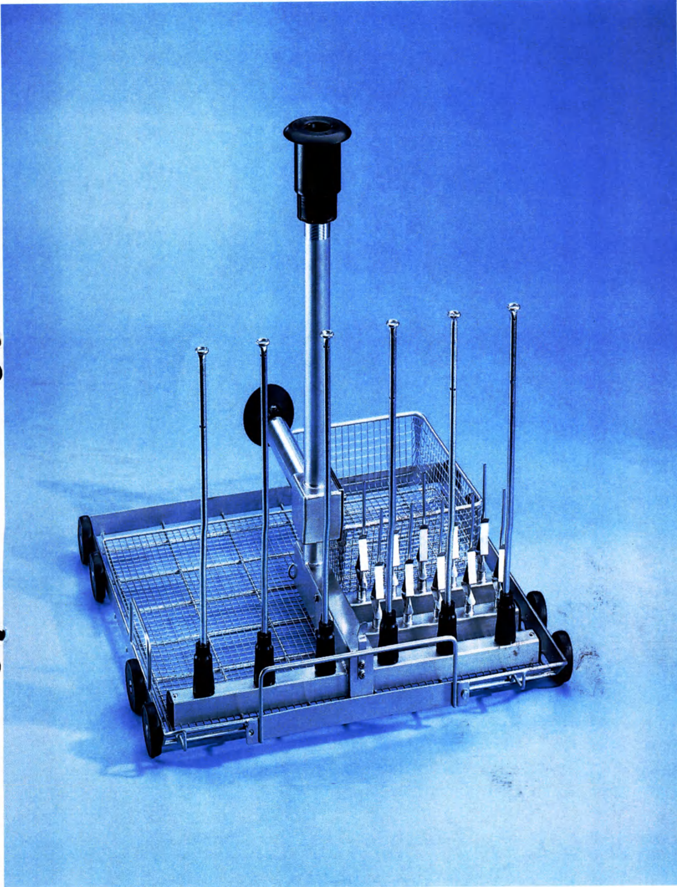
Тележка Е 501, Е 503 для размещения вставок, контейнеров и специальных медицинских инструментов для автоматов для мойки и дезинфекции G 7882, G 7882 CD
