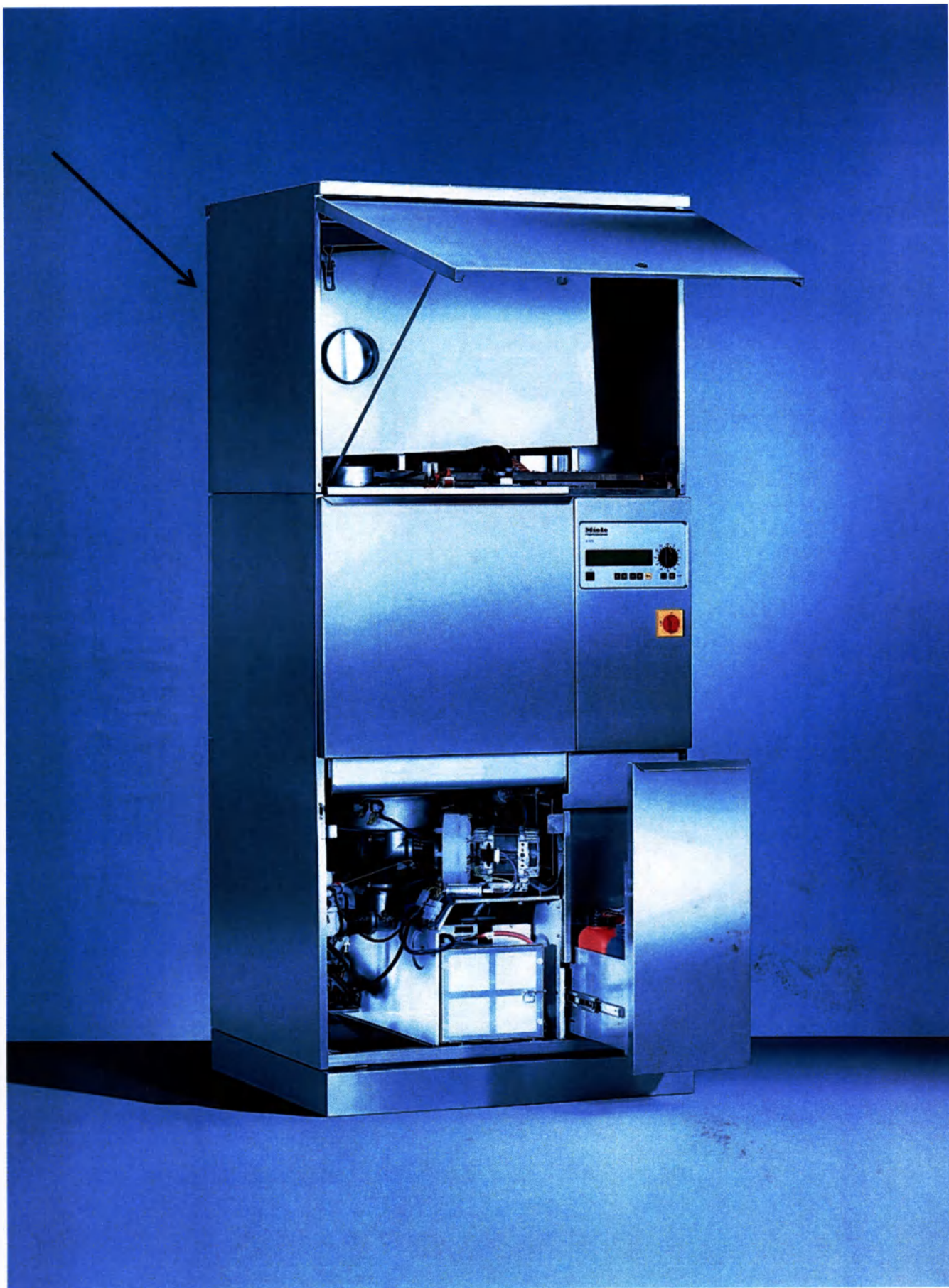
Монтажный комплект MAV 23/24 для автоматов для мойки и дезинфекции G 7823, G 7824
