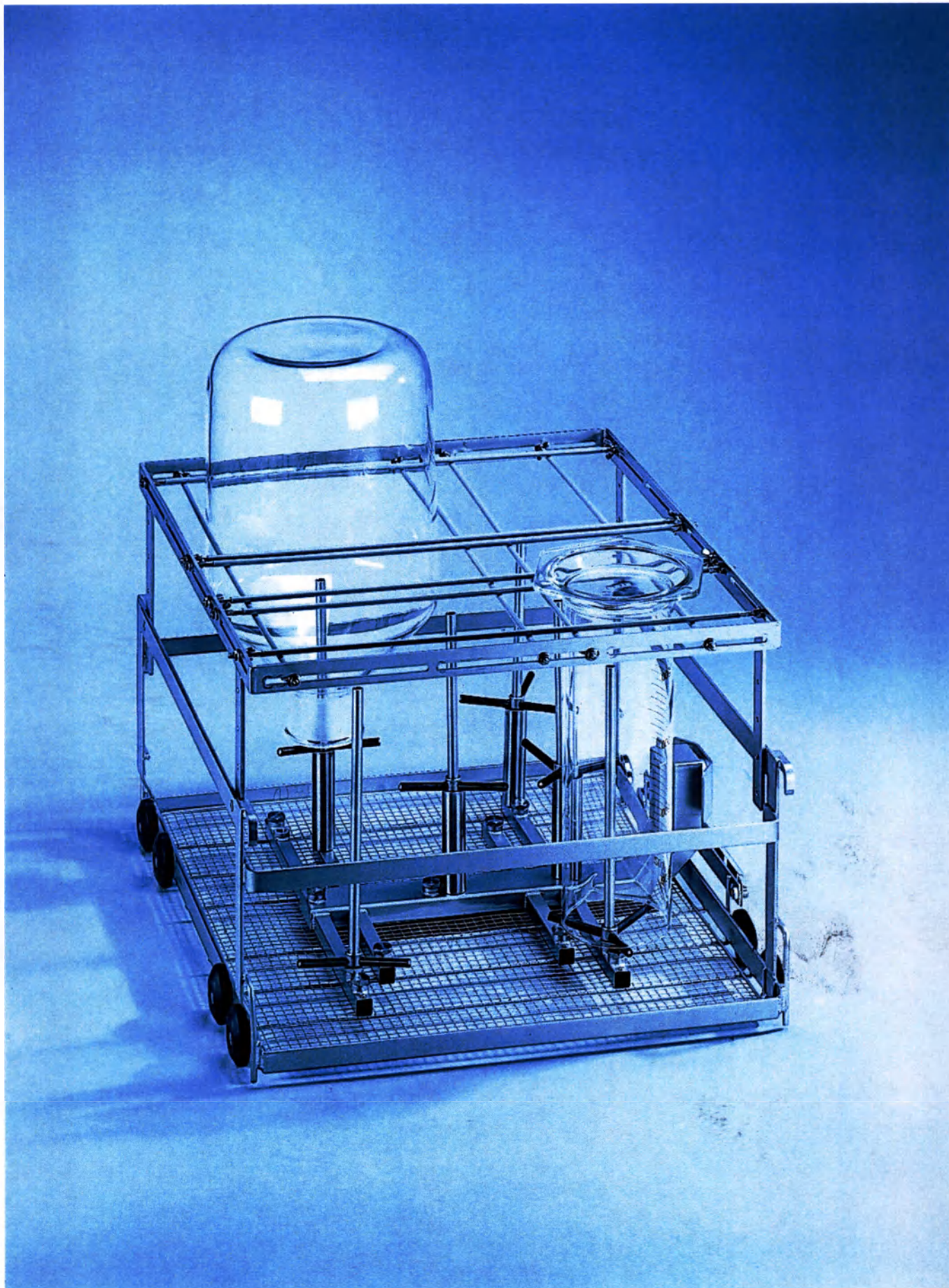
Тележка Е 757 для размещения вставок и контейнеров, а также медицинских инструментов и лабораторного стекла для автоматов для мойки и дезинфекции G 7825, G 7826
