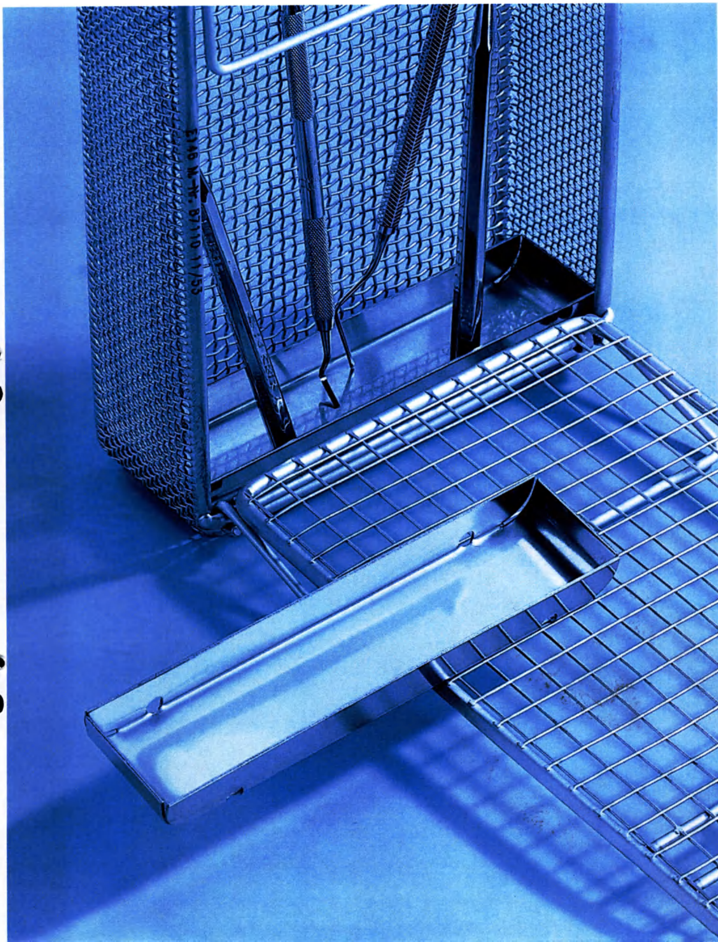
Вставка Е 328 для размещения медицинского и стоматологического инструмента, а также лабораторного стекла для автоматов для мойки и дезинфекции G 7831, G 7881, G 7882, G 7882 CD, G 7883, G 7883 CD
