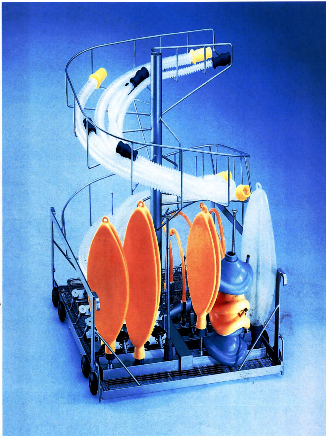
Тележка Е 715/1 для размещения вставок и контейнеров, а также медицинских инструментов и лабораторного стекла для автоматов для мойки и дезинфекции G 7825, G 7826
