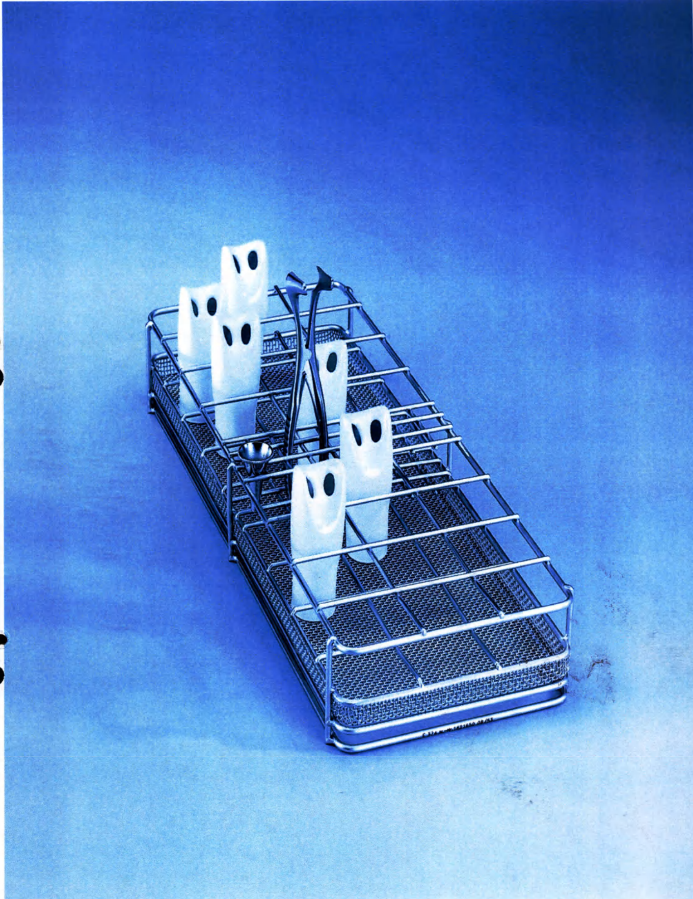
Вставка Е 374 для размещения медицинского инструмента и лабораторного стекла для автоматов для мойки и дезинфекции G 7825, G 7826, G 7882, G 7882 CD, G 7883, G 7883 CD
