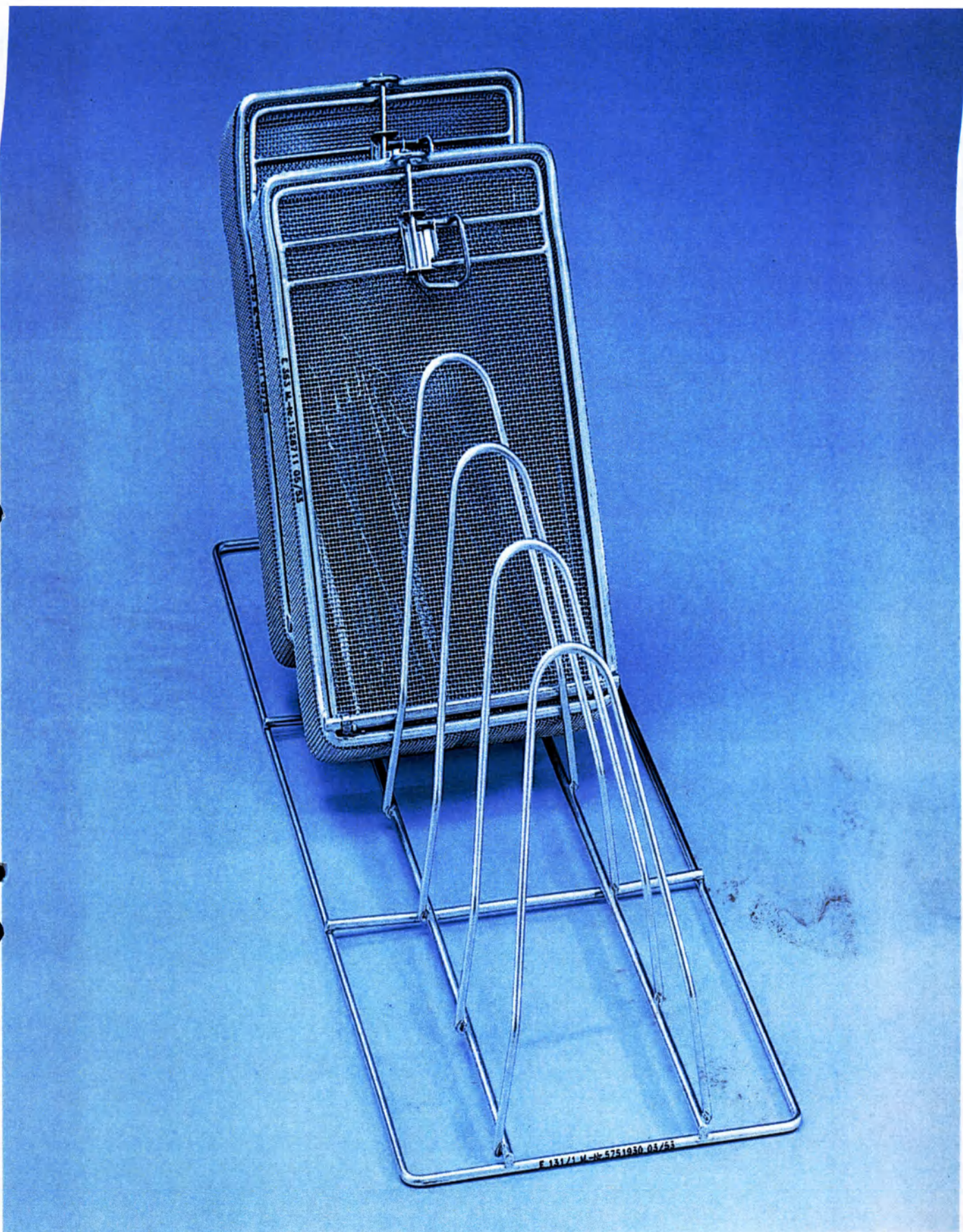
Вставка Е 131/1 для размещения медицинского инструмента и лабораторного стекла для автоматов для мойки и дезинфекции G 7823, G 7824, G 7825, G 7826, G 7831, G 7881, G 7882, G 7882 CD, G 7883, G 7883 CD
