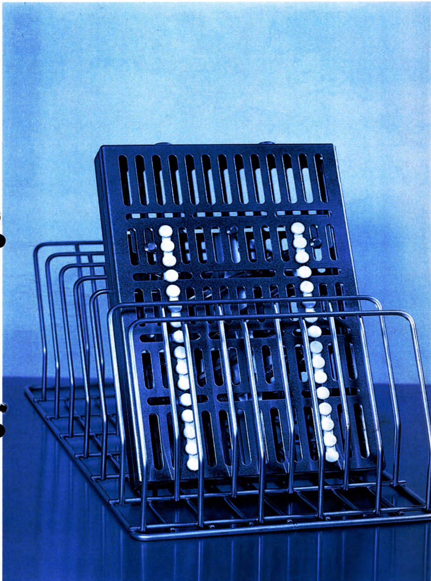
Вставка Е 523 для размещения медицинского и стоматологического инструмента для автоматов для мойки и дезинфекции G 7823, G 7824, G 7825, G 7826, G 7831, G 7881, G 7882, G 7882 CD
