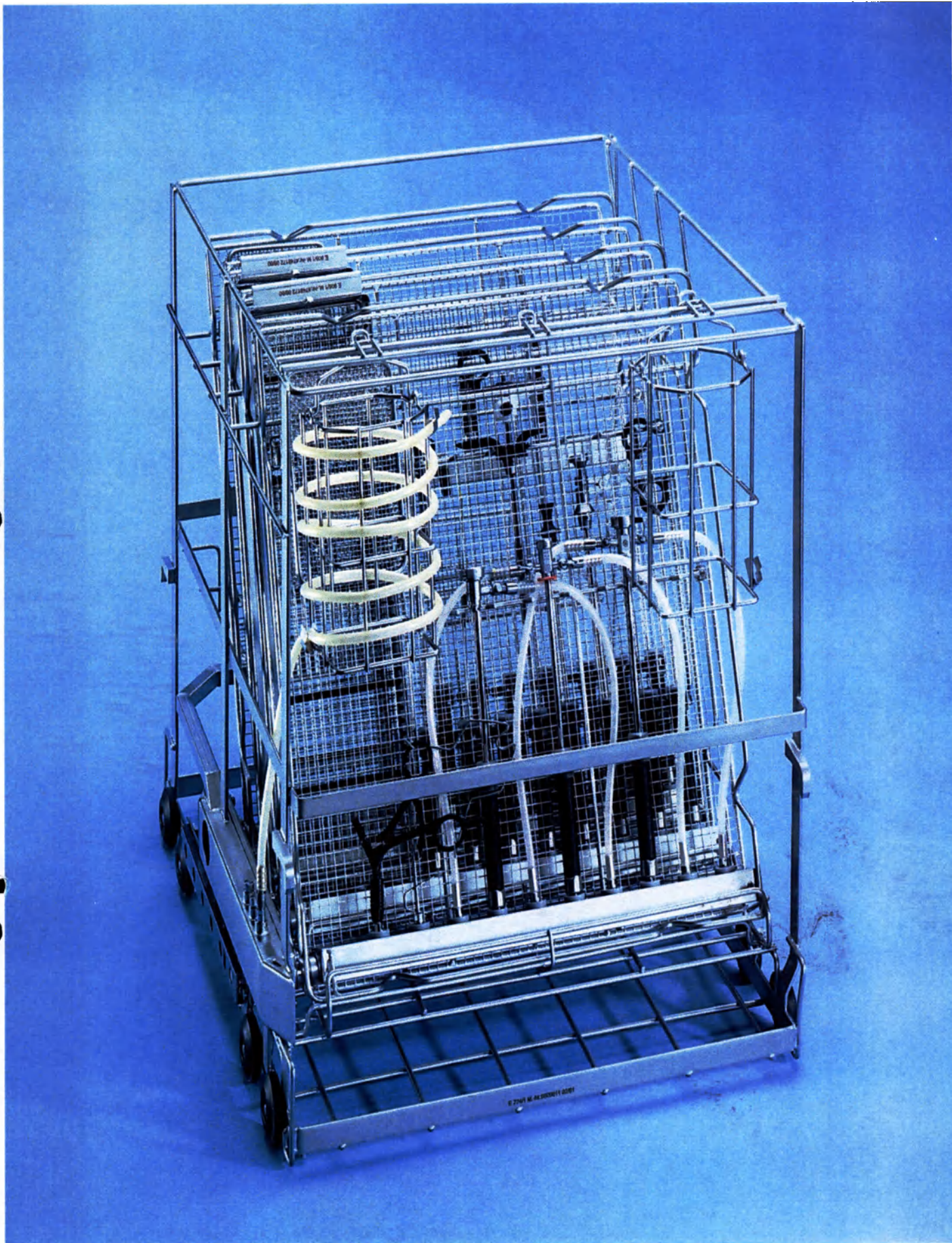
Тележка Е 774/1 для размещения вставок и контейнеров, а также медицинских инструментов и лабораторного стекла для автоматов для мойки и дезинфекции G 7825, G 7826
