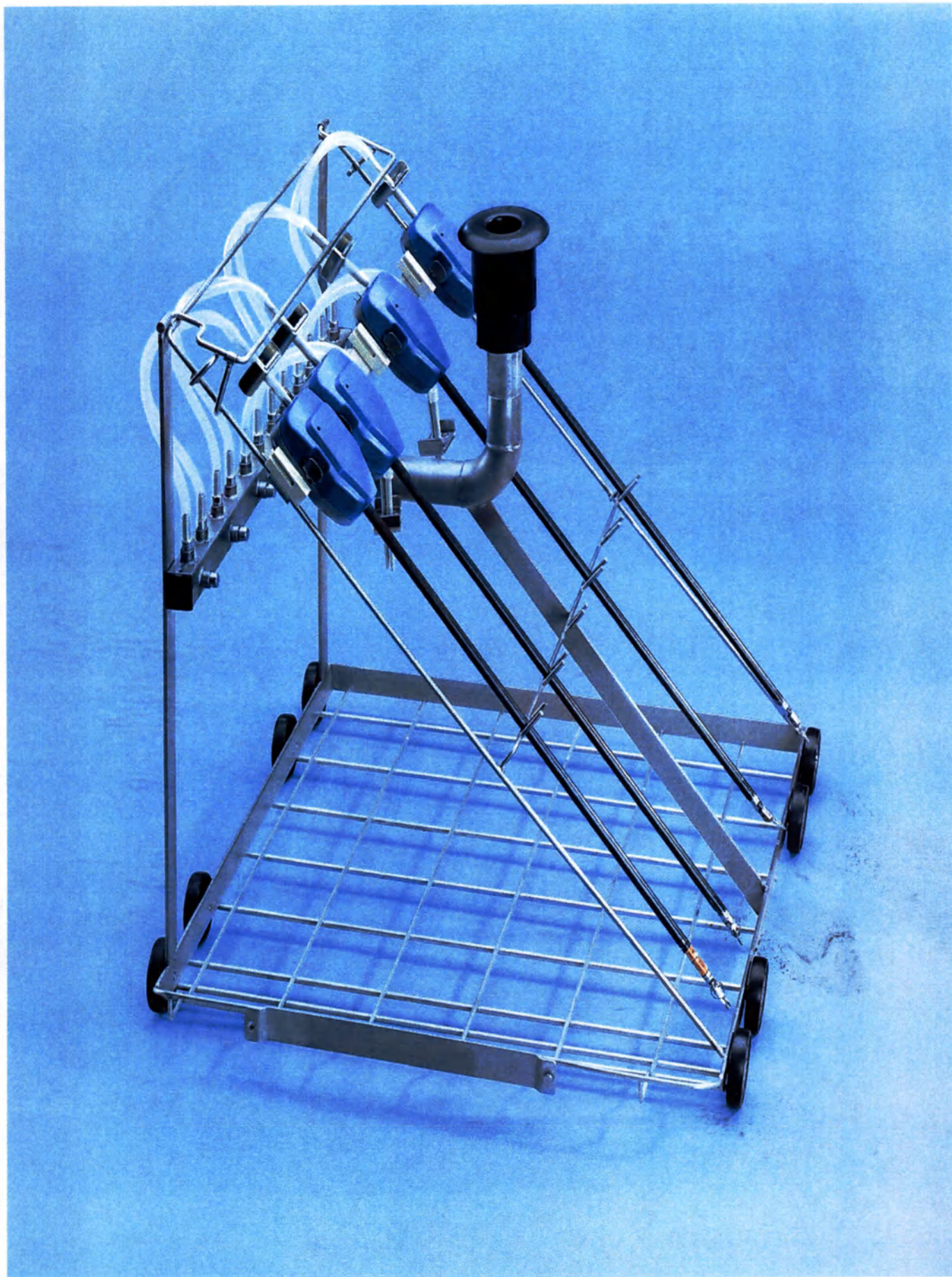
Тележка Е 428 для размещения вставок, контейнеров и специальных медицинских инструментов, а также лабораторного стекла для автоматов для мойки и дезинфекции G 7882, G 7882 CD
