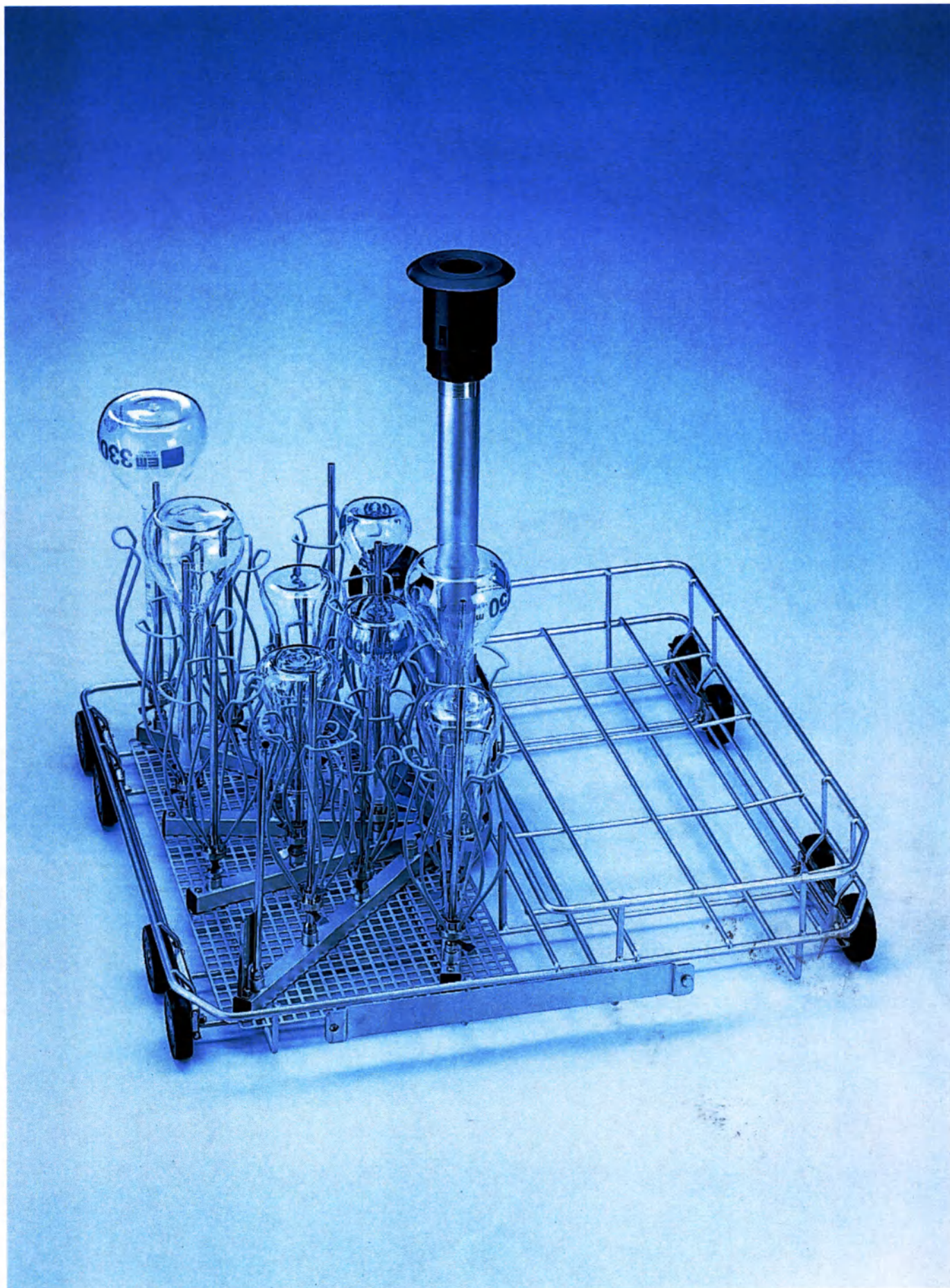
Тележка Е 385 для размещения лабораторного стекла для автоматов для мойки и дезинфекции G 7883, G 7883 CD
