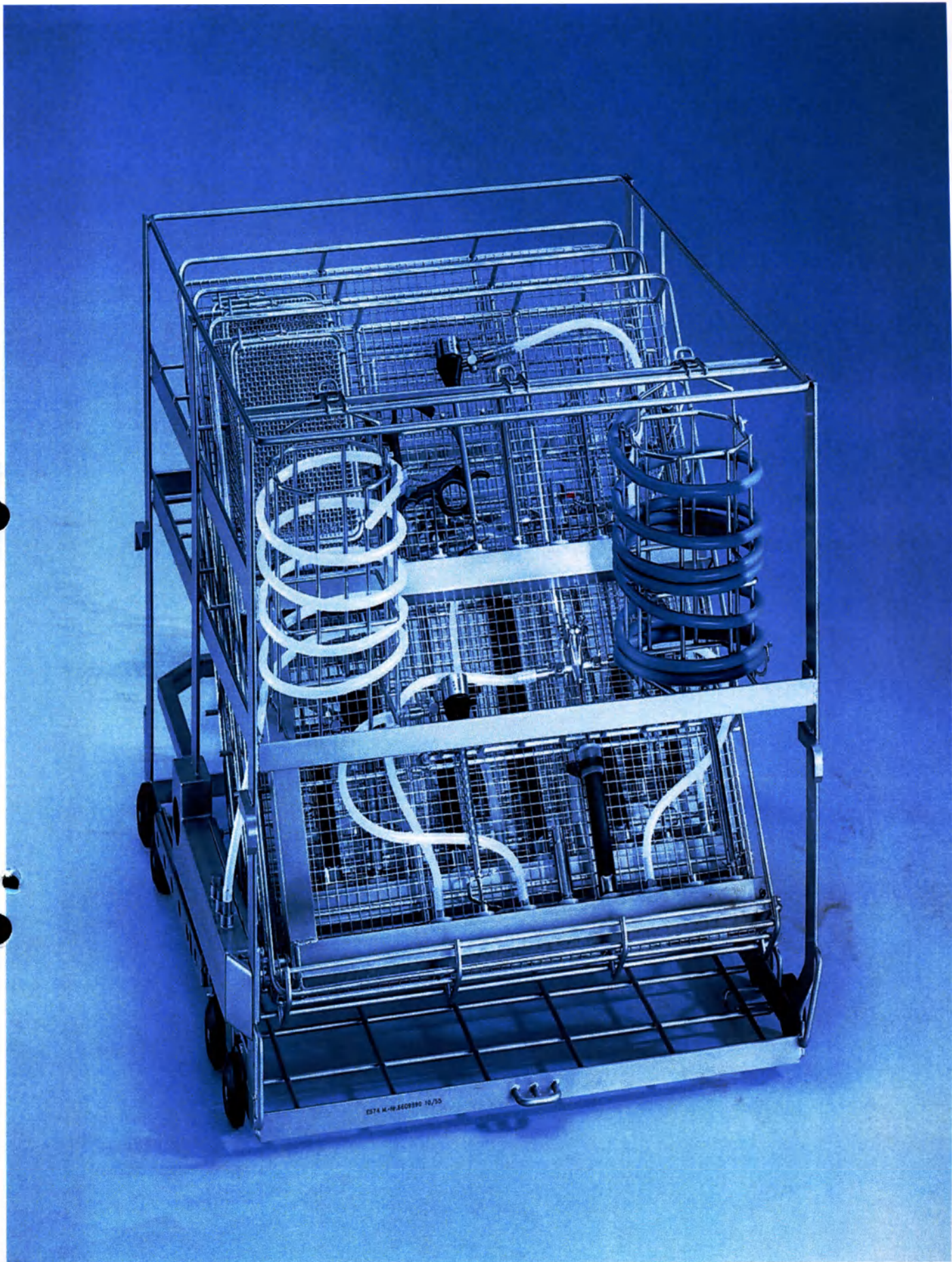
Тележка Е 574 для размещения вставок и специальных медицинских инструментов для автоматов для мойки и дезинфекции G 7823, G 7824
