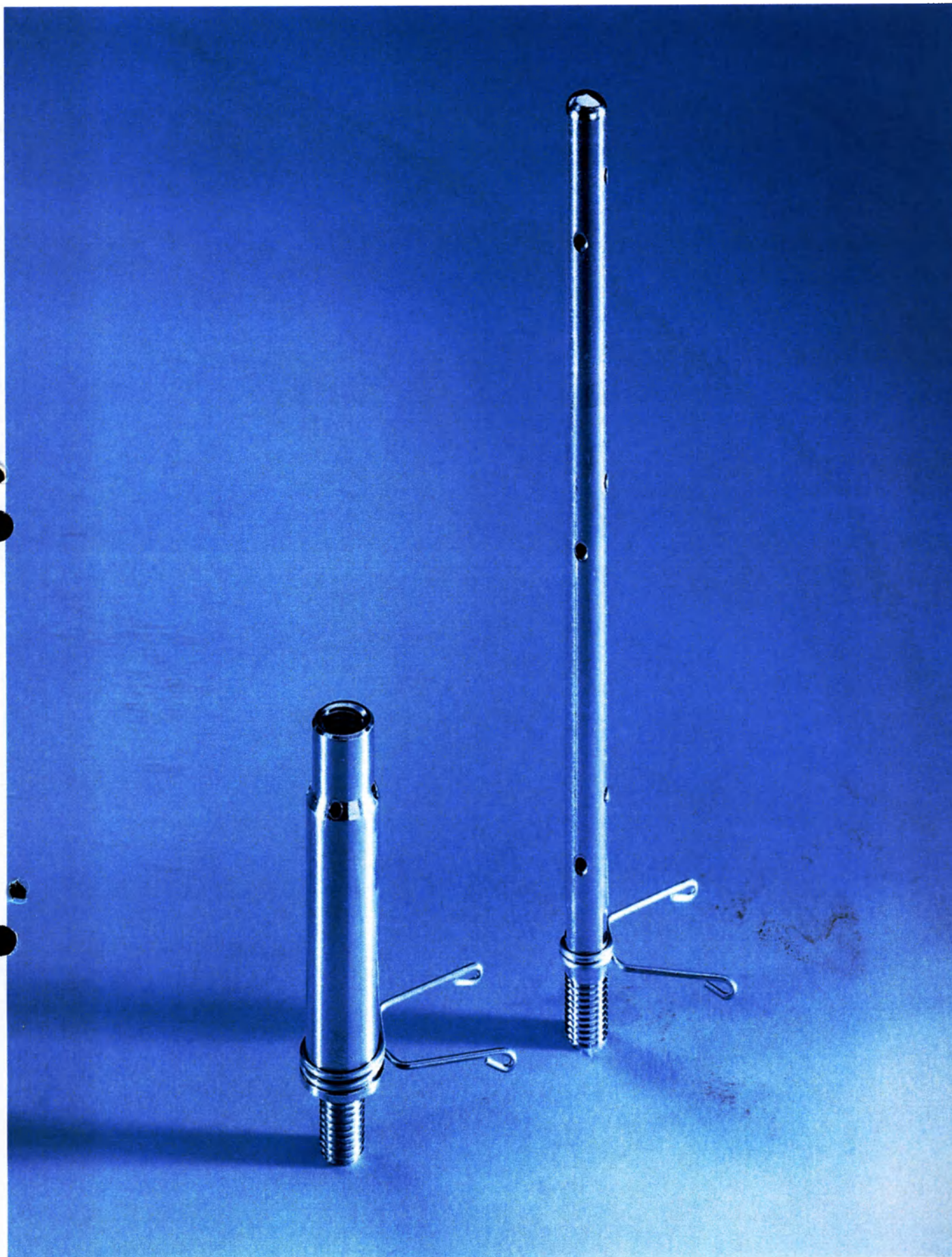
Промывочная втулка Е 464 и инжекторное сопло Е 454 для размещения микроинструмента и лабораторного стекла для автоматов для мойки и дезинфекции G 7823, G 7824, G 7825, G 7826, G 7882, G 7882 CD, G 7883, G 7883 CD
