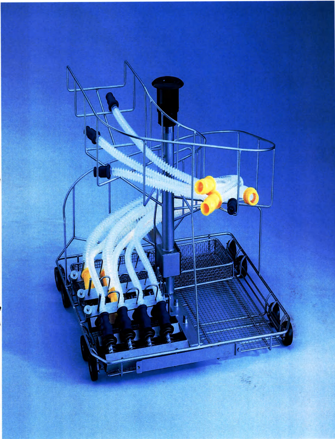
Тележка Е 461/2 для размещения вставок, контейнеров и специальных медицинских инструментов для автоматов для мойки и дезинфекции G 7882, G 7882 CD
