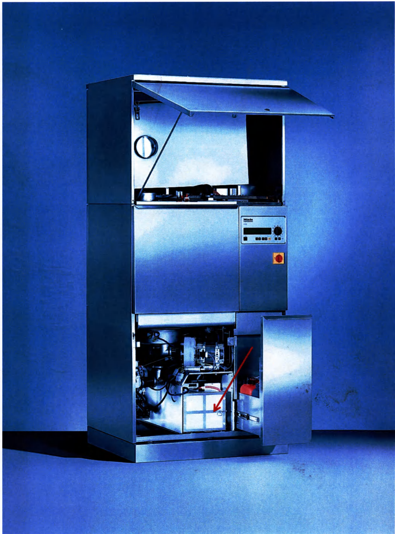
Системы сушки горячим воздухом TA-S1 для автоматов для мойки и дезинфекции G 7823, G 7824
