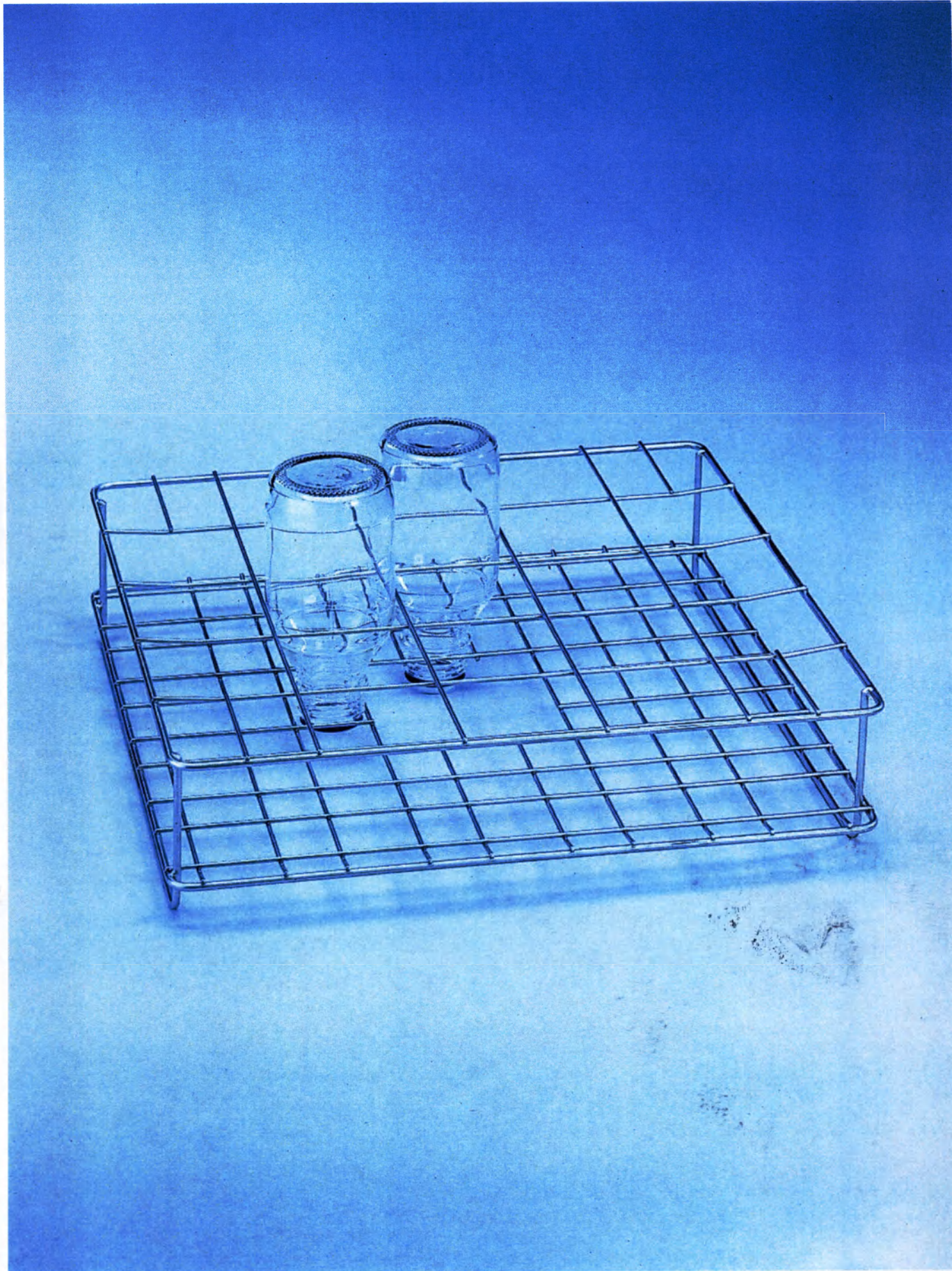
Вставка Е 129 для размещения медицинского инструмента и лабораторного стекла для автоматов для мойки и дезинфекции G 7825, G 7826, G 7883, G 7883 CD
