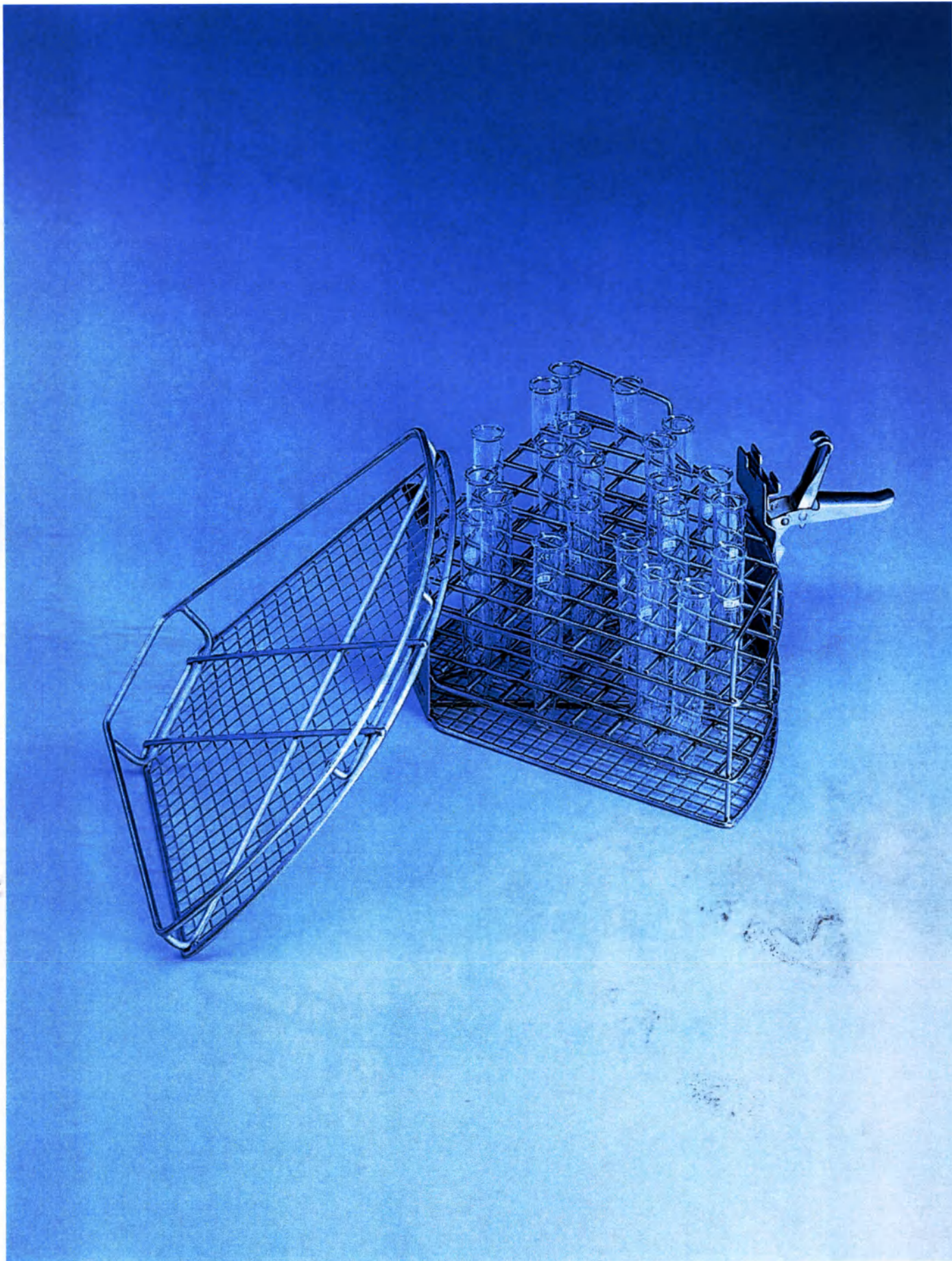
Вставка Е 149 для размещения медицинского инструмента и лабораторного стекла для автоматов для мойки и дезинфекции G 7825, G 7826
