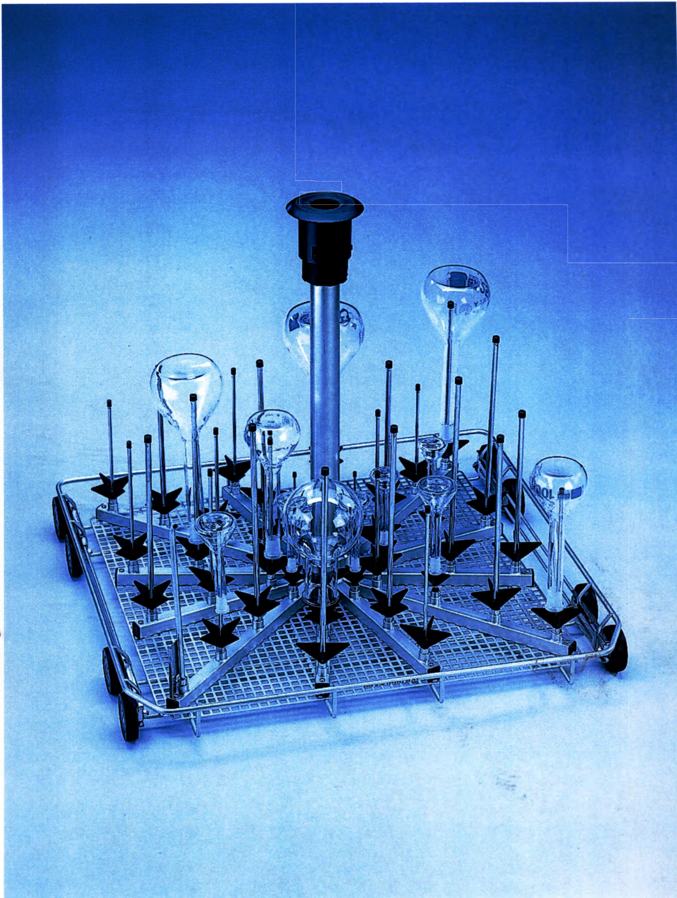
Тележка Е 329 для размещения лабораторного стекла для автоматов для мойки и дезинфекции G 7883, G 7883 CD
