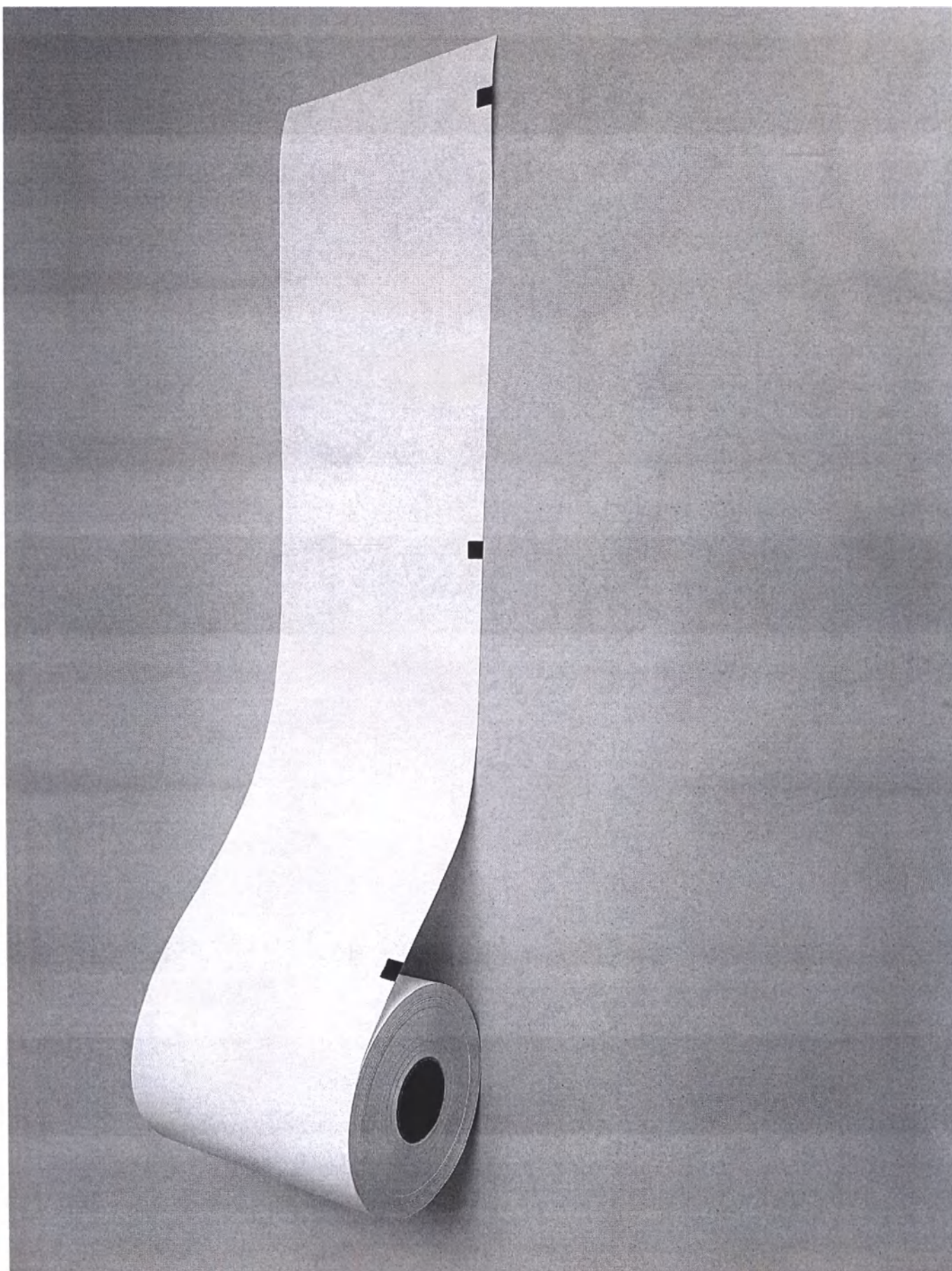
Общий вид бумаги (ленты) для электроэнцефалографической регистрации в рулонах без диаграммной сетки, с фотометками, с намоткой термослоем наружу ЭЭГ-Р-Ч-М-Н
