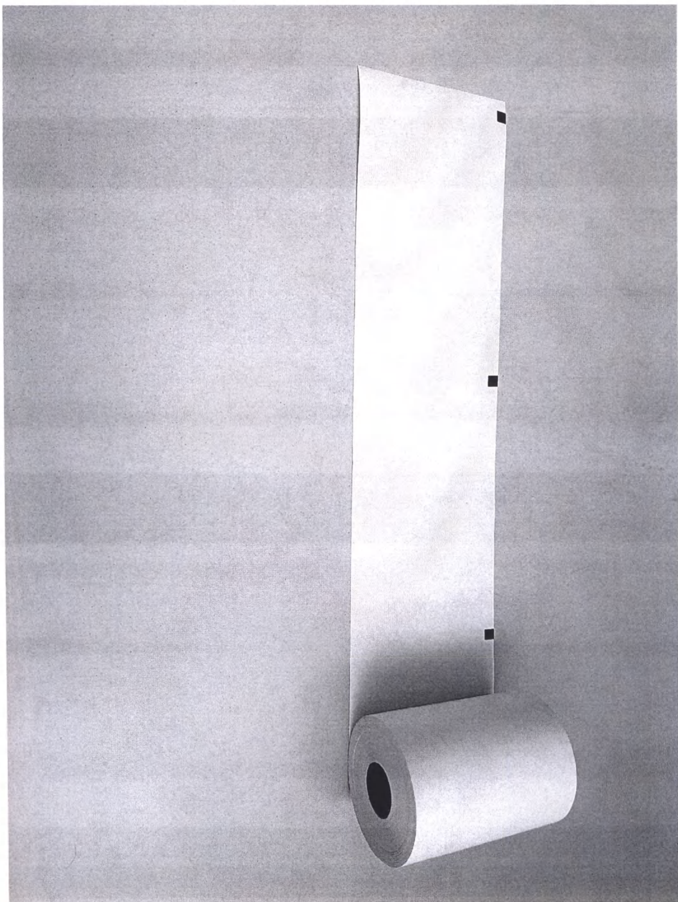
Общий вид бумаги (ленты) для электроэнцефалографической регистрации в рулонах без диаграммной сетки, с фотометками, с намоткой термослоем внутри ЭЭГ-Р-Ч-М-В
