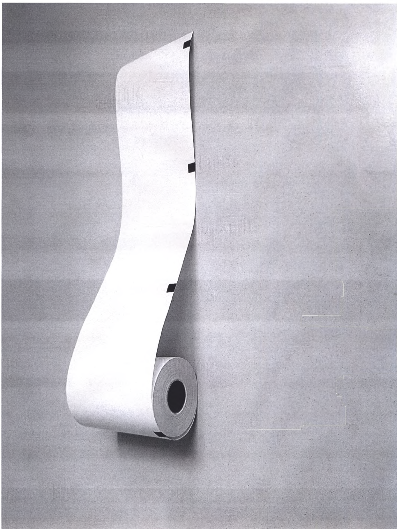
Общий вид бумаги (ленты) для эхокардиографического самописца в рулонах без диаграммной сетки, с фотометками, с намоткой термослоем наружу ЭХО-Р-Ч-М-Н
