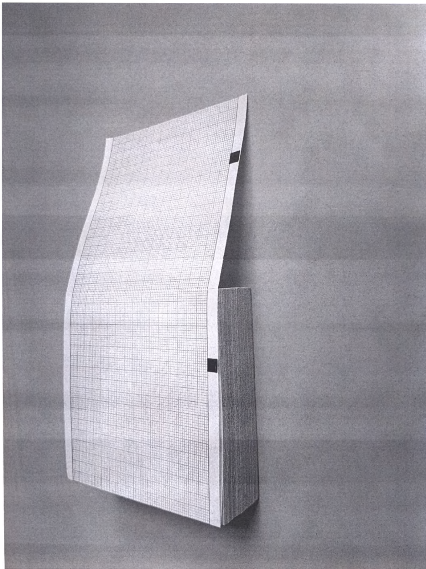
Общий вид бумаги (ленты) принтера для лабораторного прибора в пачке с диаграммной сеткой, с фотометками ПЛП-П-С-М
