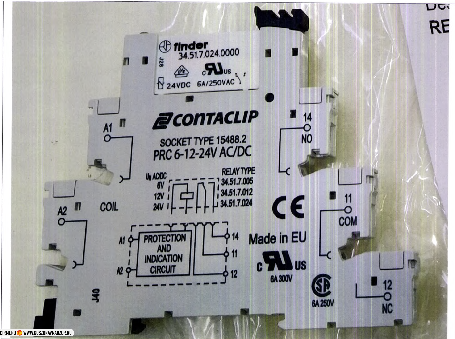
137. Реле электромагнитные с держателем - 2шт. (Не более (при необходимости))
