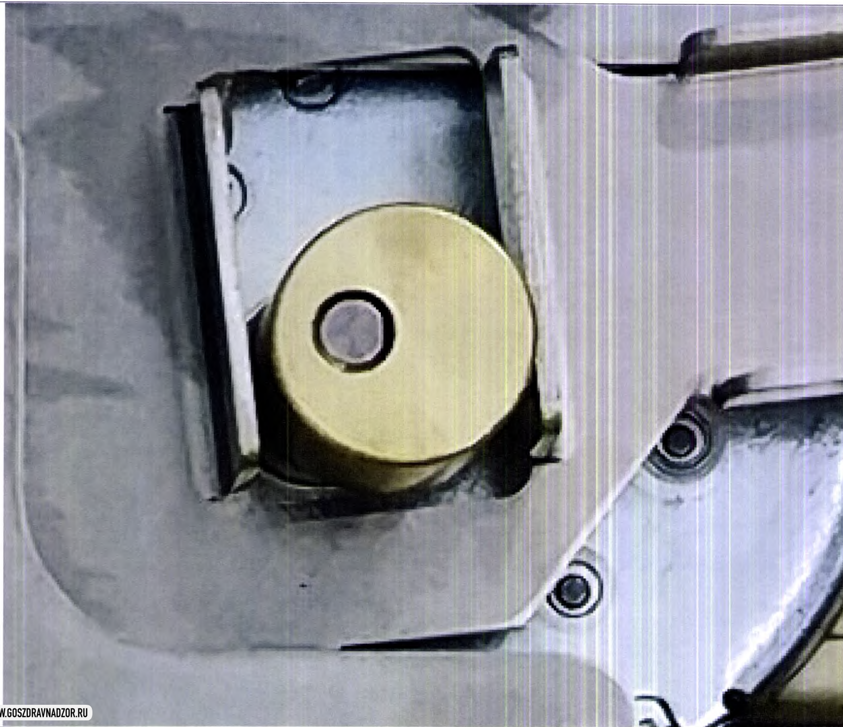
166. Эксцентрик электродвигателя механизма блокировки двери - 1шт.
