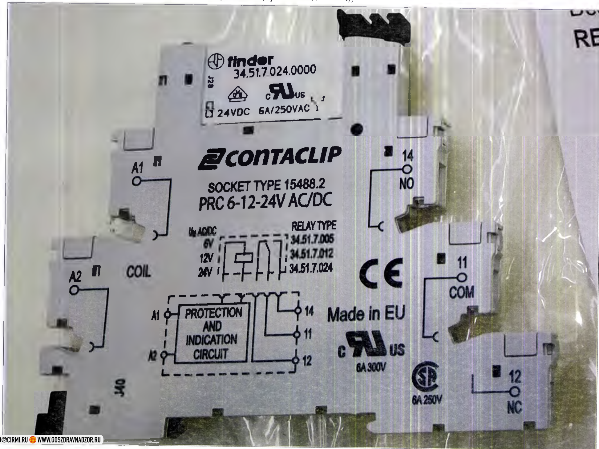
163. Реле электромагнитные с держателем - 5шт. (Не более (при необходимости))
