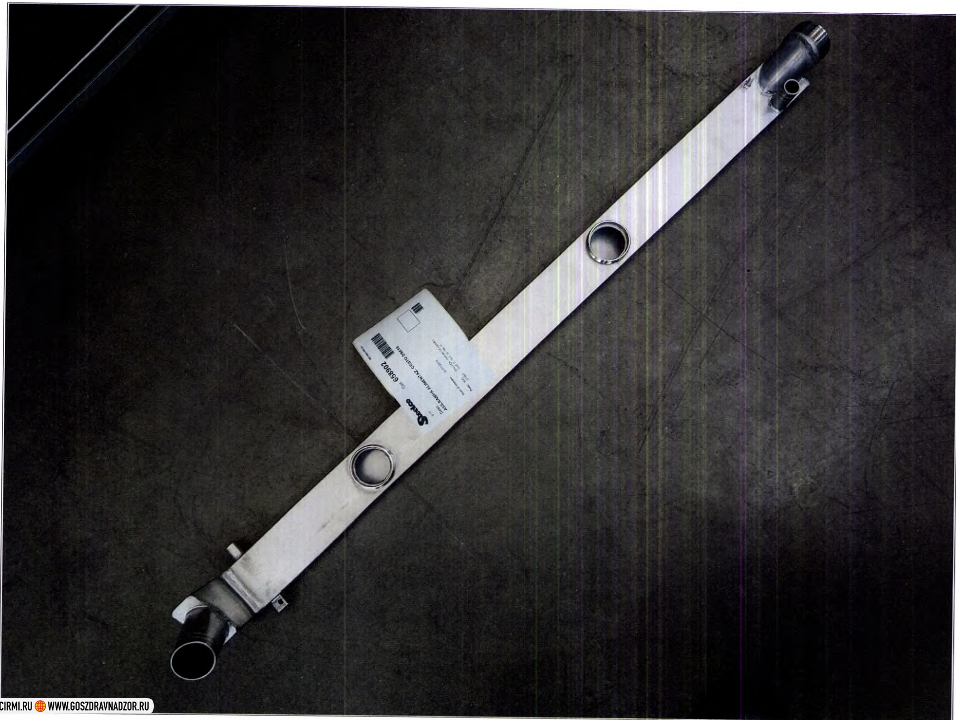
157. Рампа подачи воды в камеру - 1 шт.
