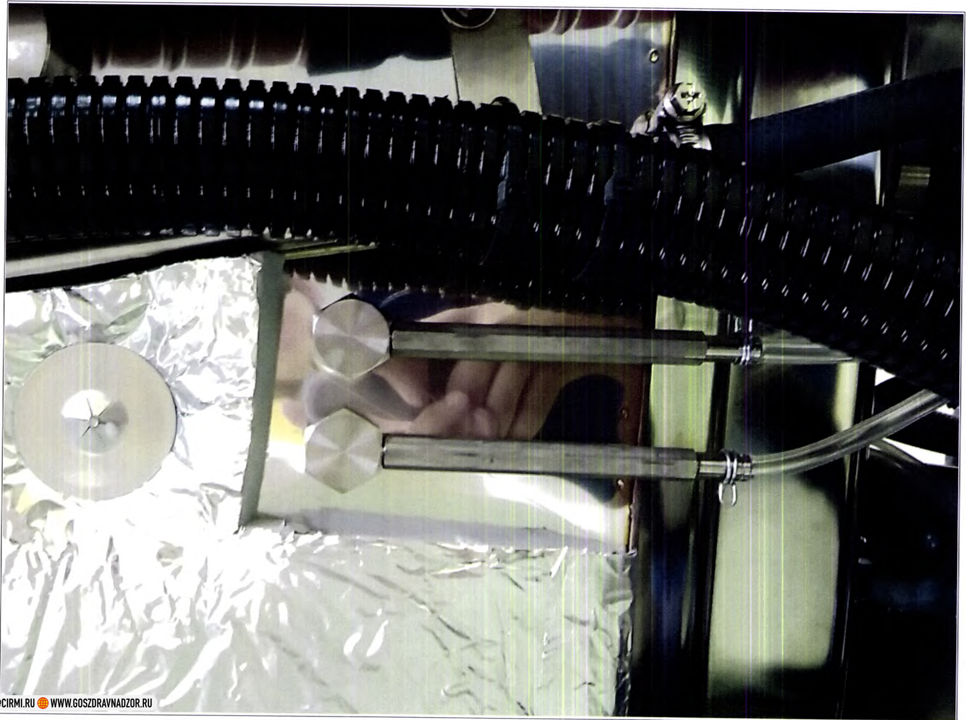
184. Трубки подачи детергента в камеру - 2шт.
