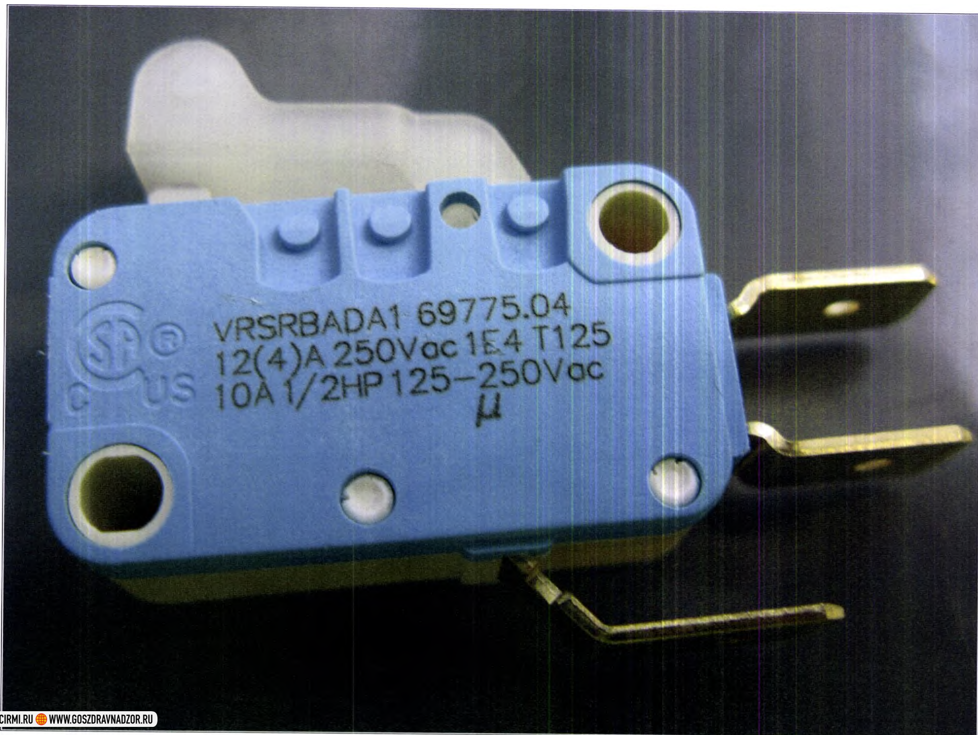
100. Микровыключатель - 2шт.
