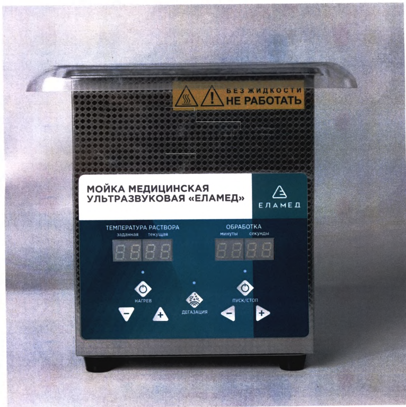
Фотографическое изображение Общий вид Мойка медицинская ультразвуковая «ЕЛАМЕД», исполнение 12.
