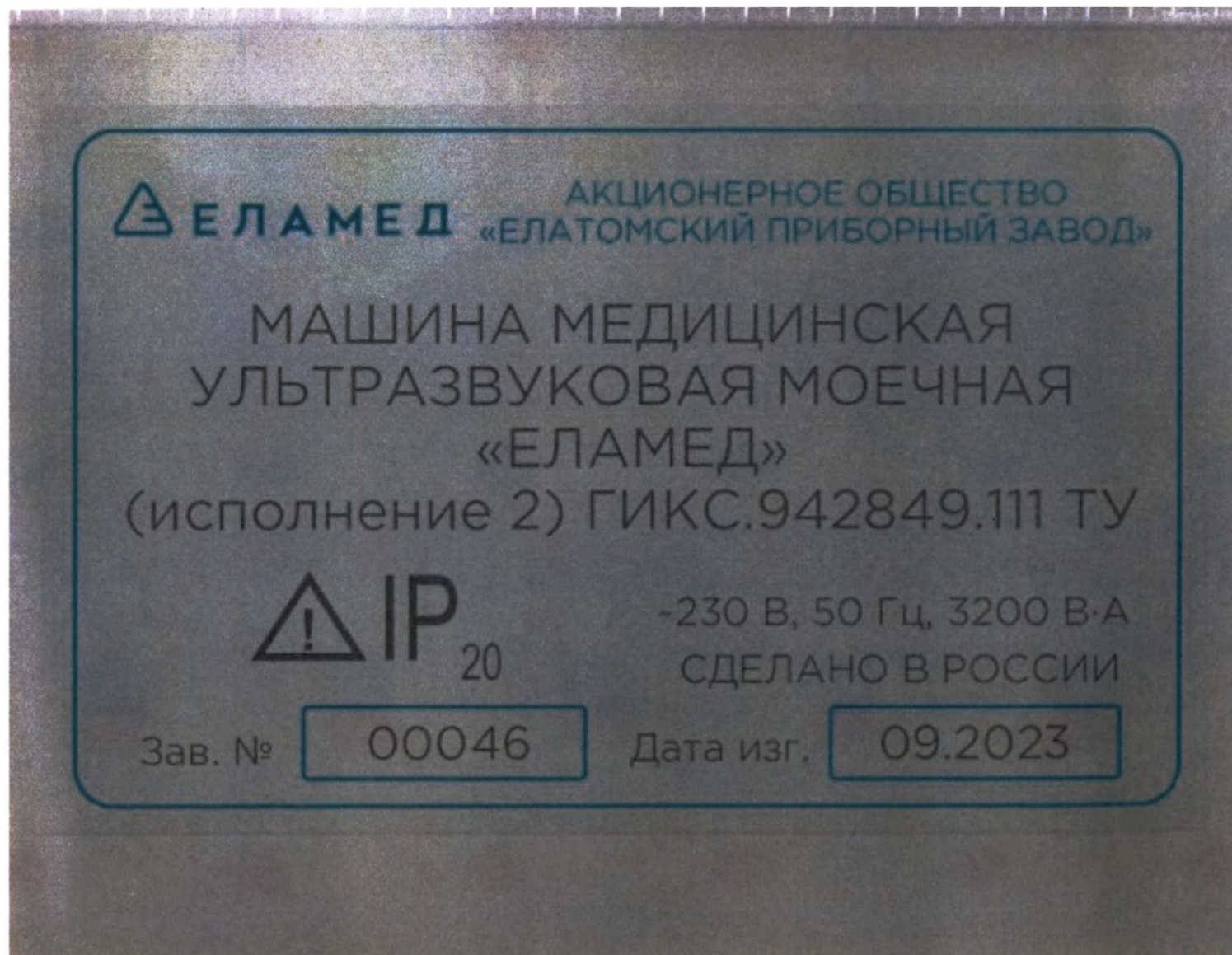
Фотографическое изображение Маркировка - шильдик Машина медицинская ультразвуковая моечная «ЕЛАМЕД», исполнение 2.
