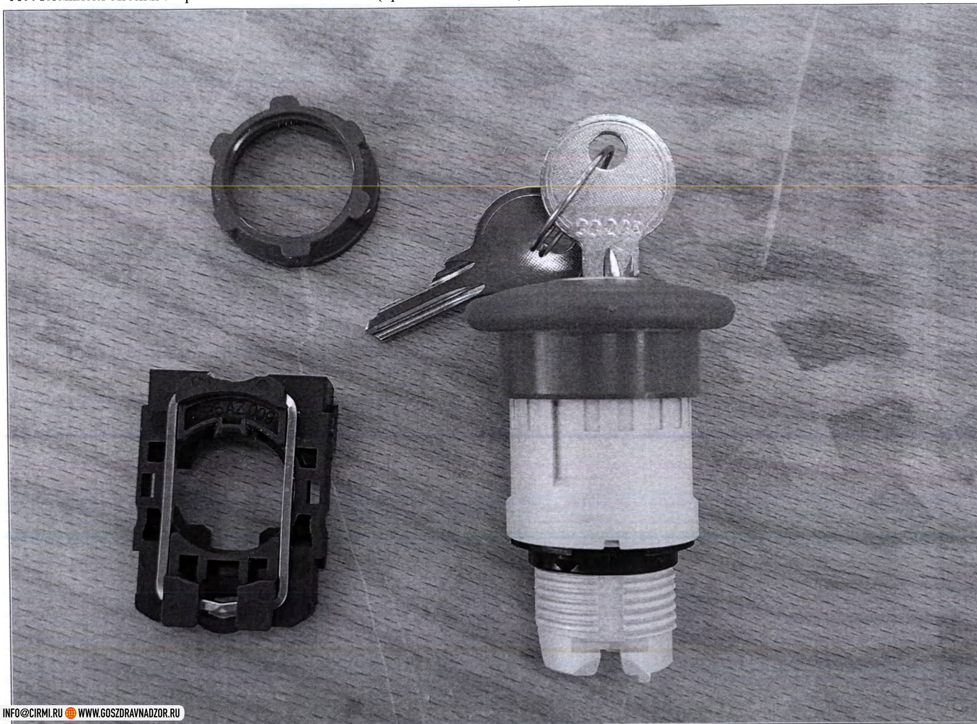
119. Комплект кнопки аварийного отключения - 1 шт. (при необходимости)
