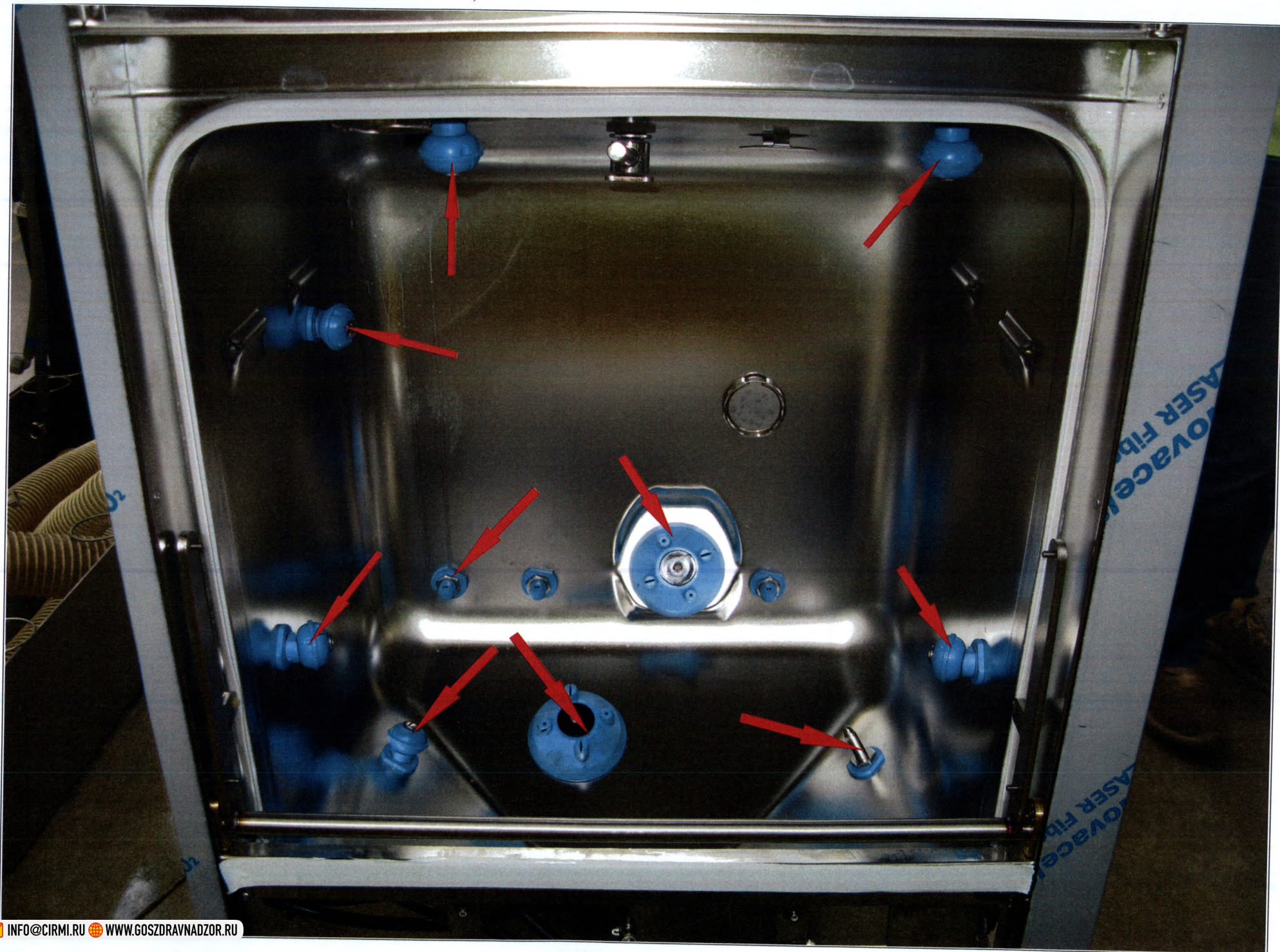
34. Комплект форсунок - 1 шт. (при необходимости)
