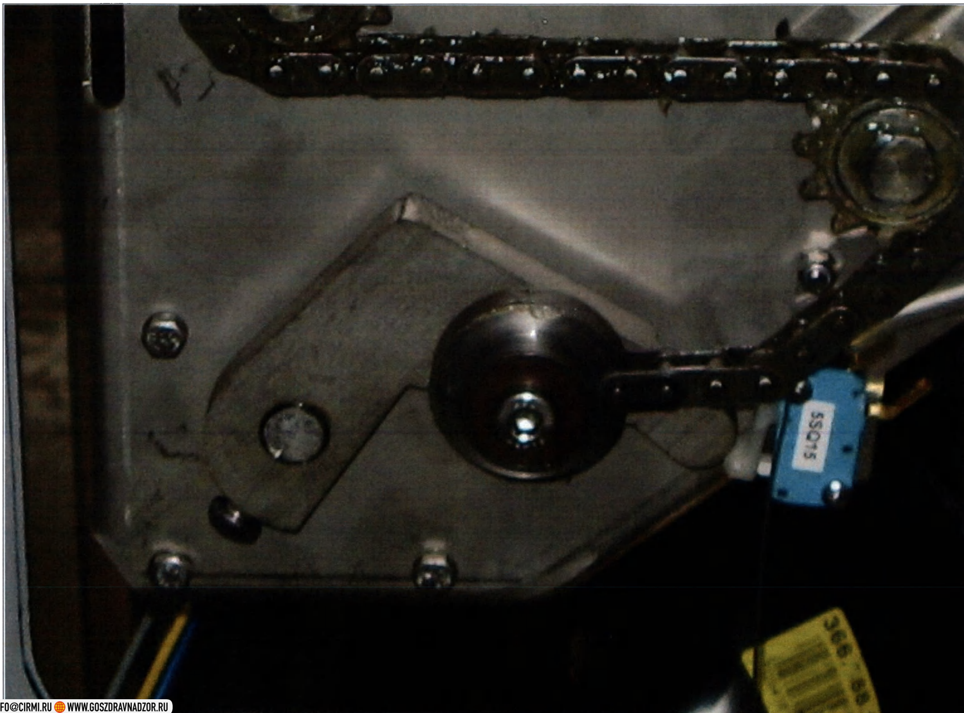
103. Эксцентрик привода двери камеры - 1шт. (при необходимости)
