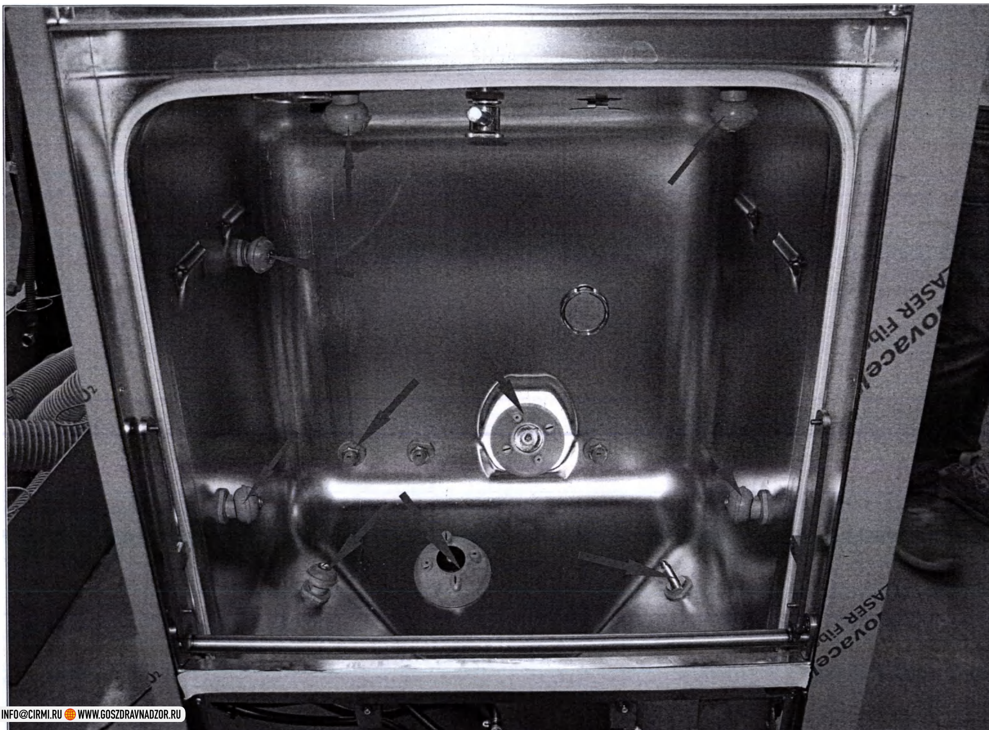
39. Комплект форсунок - 1 шт.
