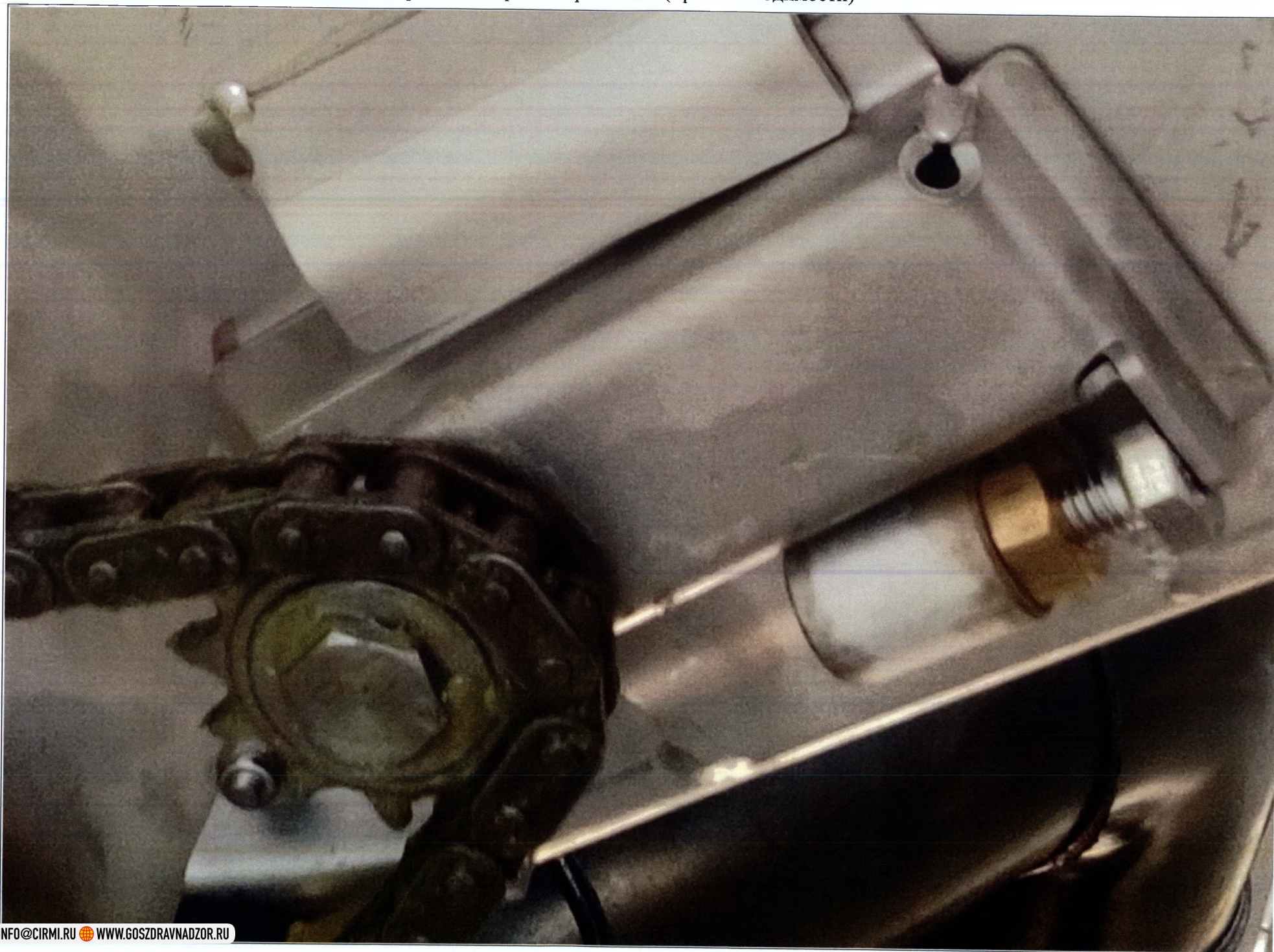
58. Кронштейн звездочки натяжения цепи привода двери камеры - 1 шт. (при необходимости)
