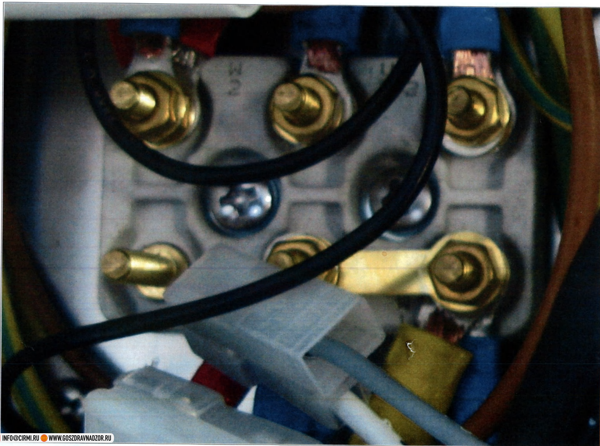
1. Блок клеммных колодок - 1шт.
