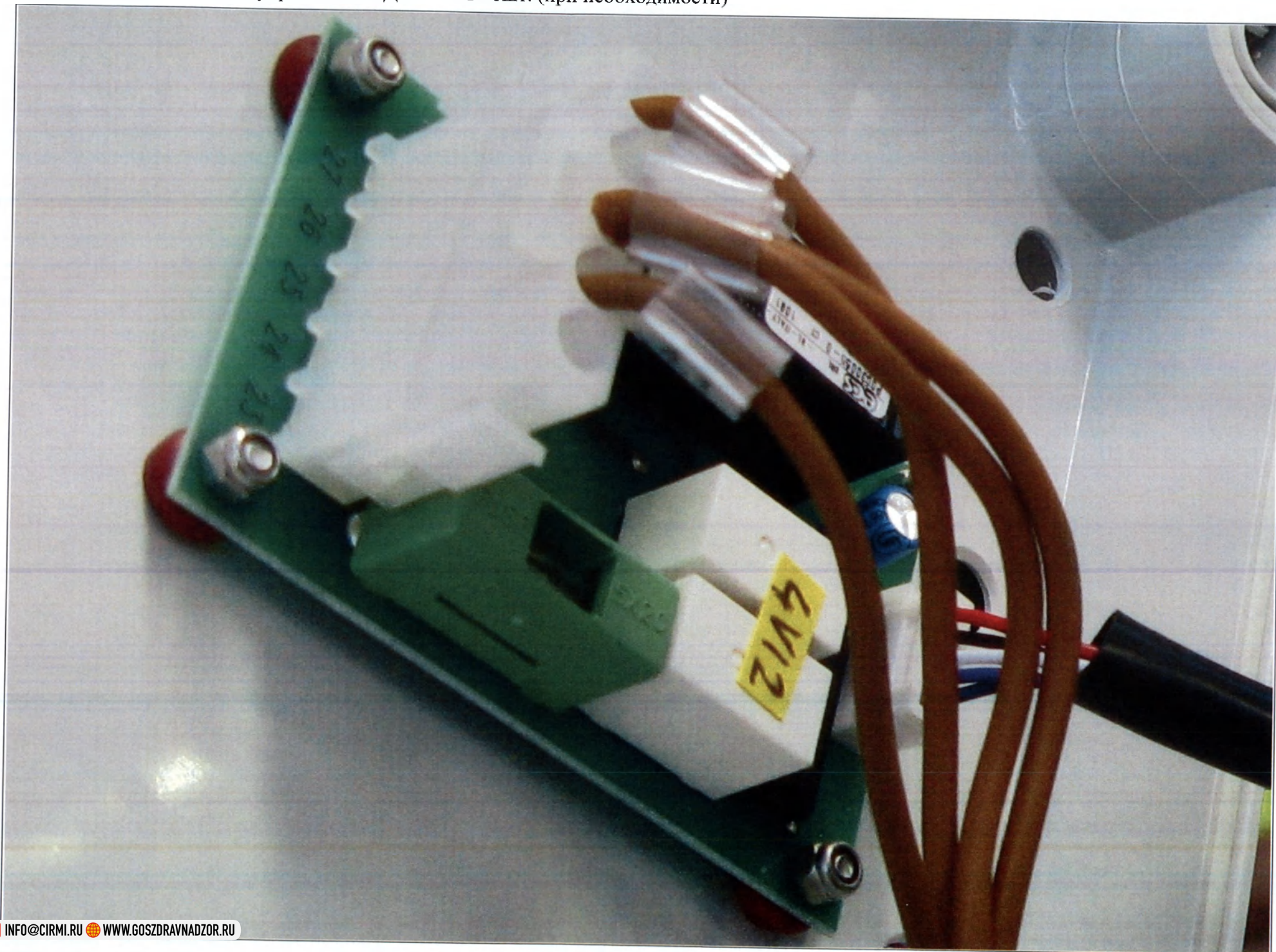
23. Дополнительная плата управления МДМ-П 1М - 1шт. (при необходимости)
