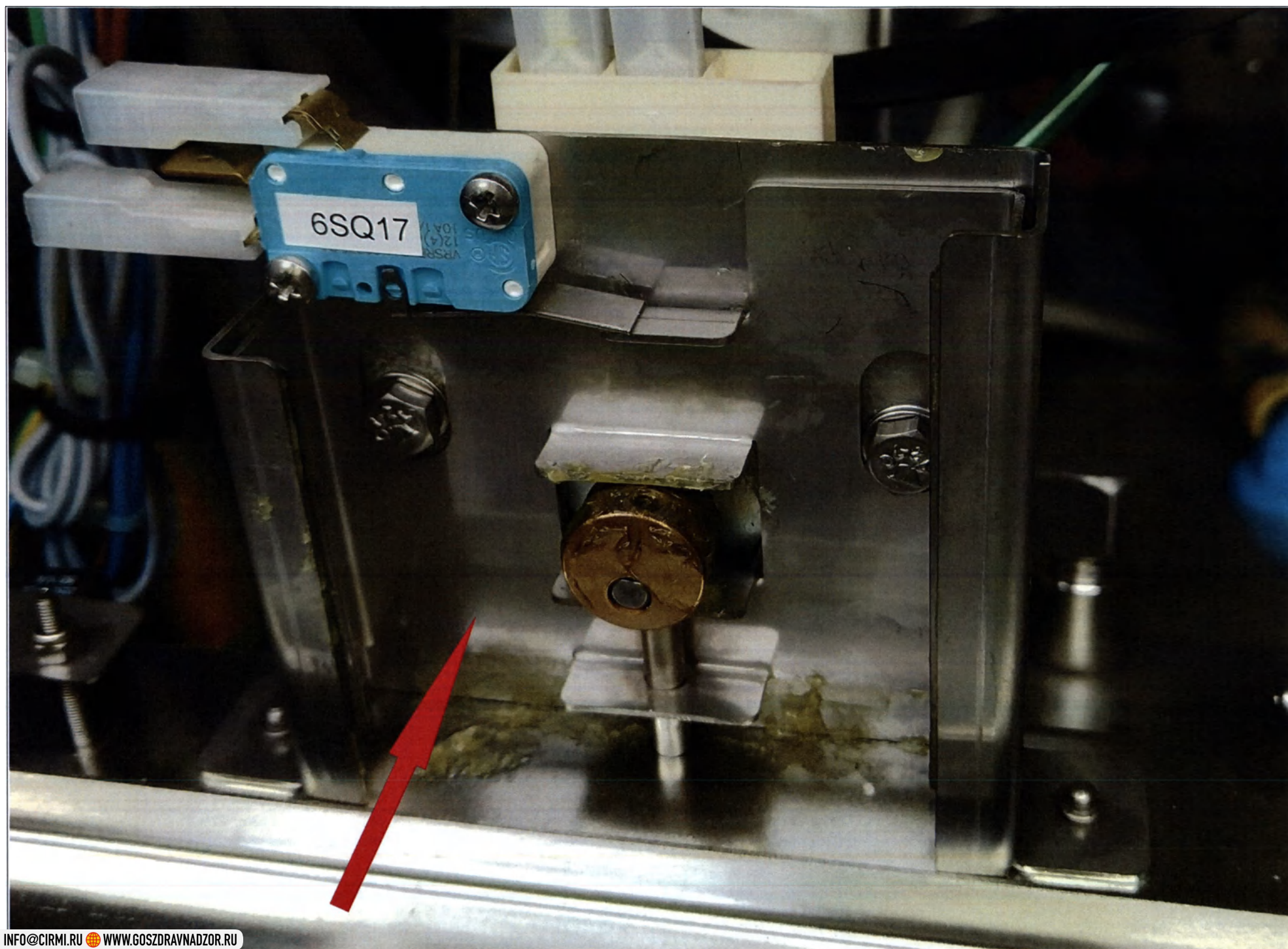
78. Пластина со штоком блокировки двери камеры - 1шт. (при необходимости)
