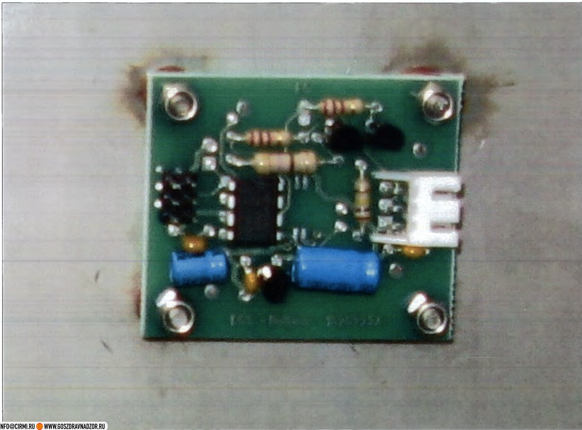
79. Плата сенсора включения привода двери - 1 шт. (при необходимости)
