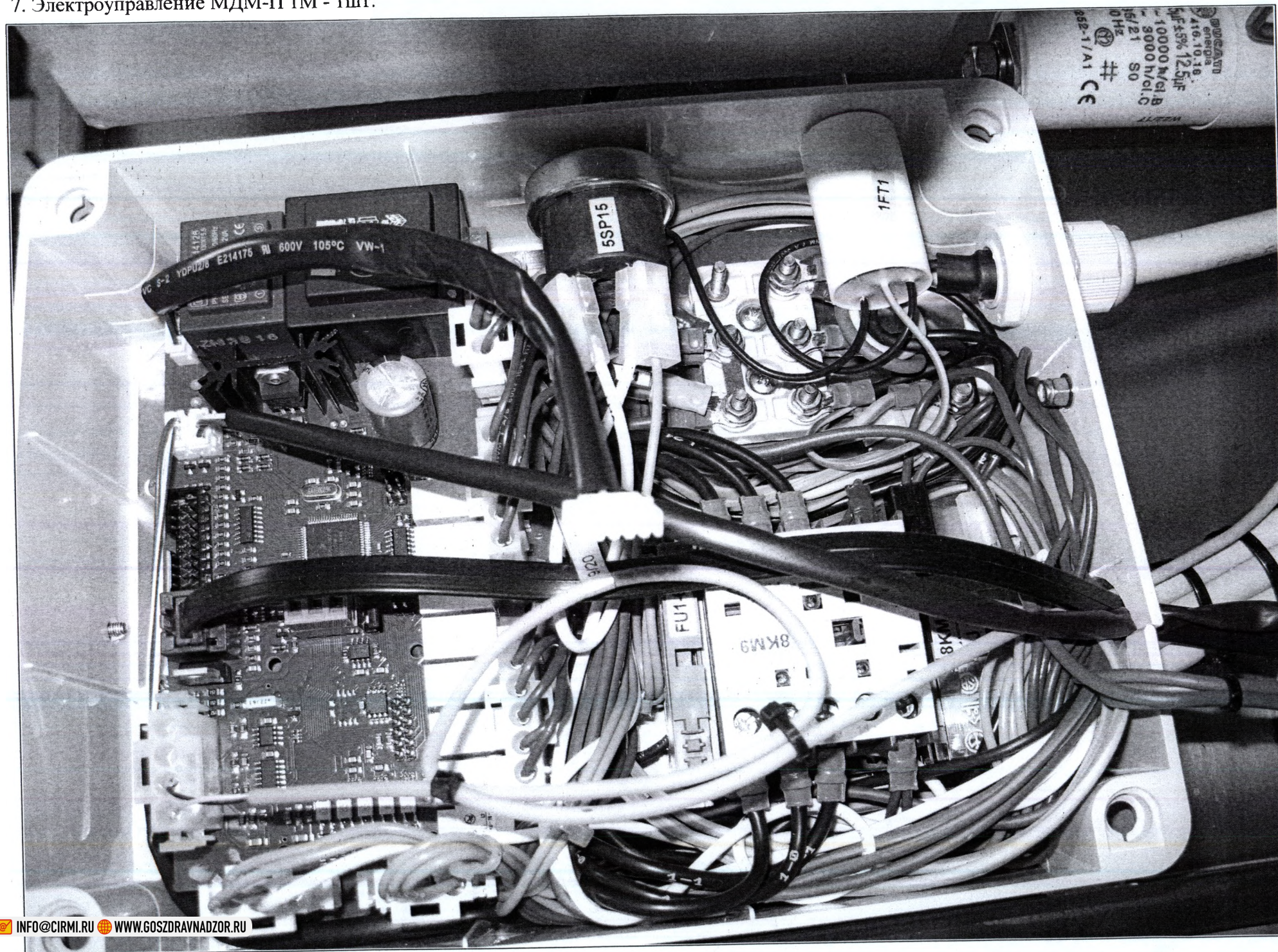
7. Электроуправление МДМ-П 1М - 1 шт.
