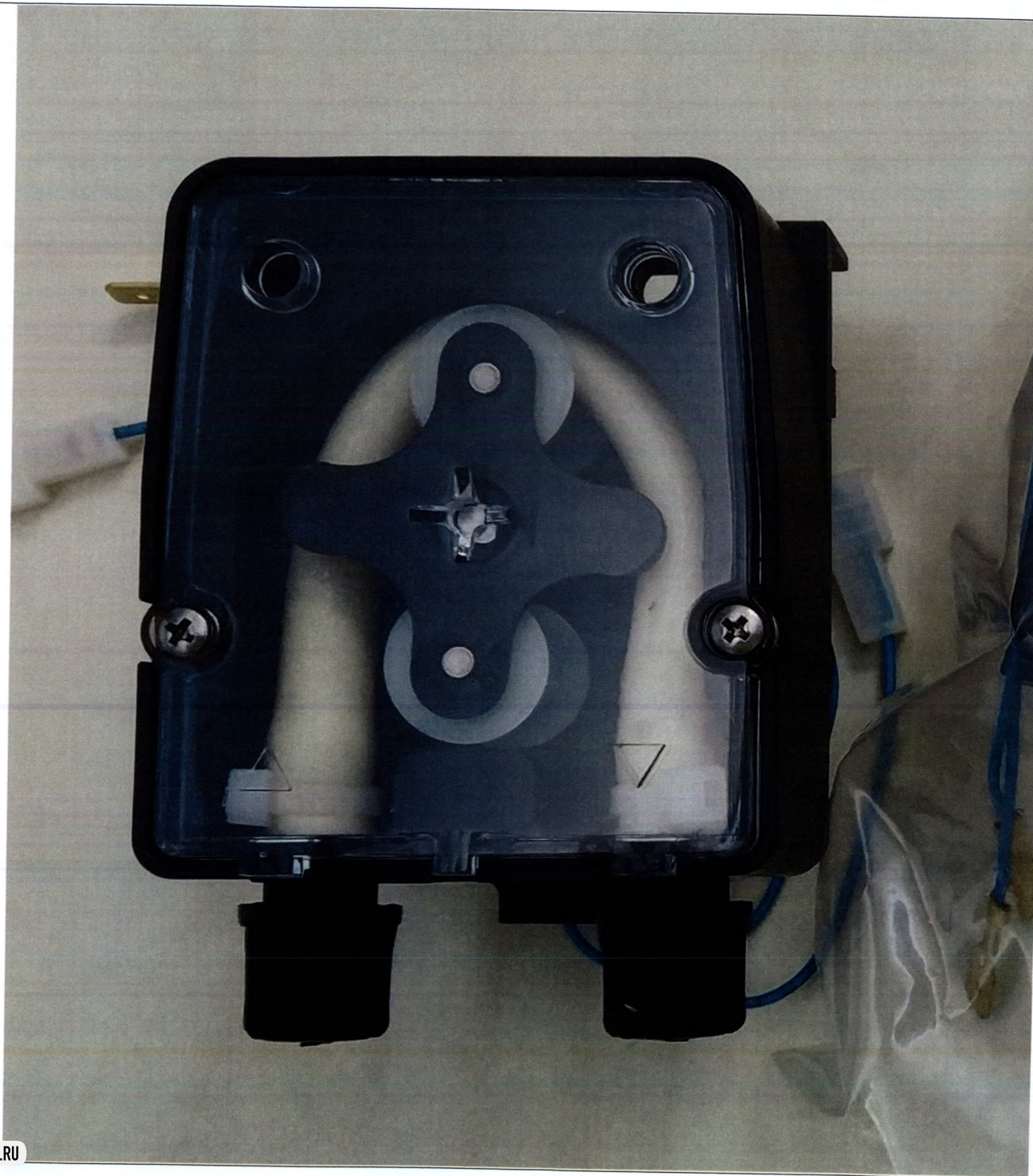
21. Дозирующий насос для детергента - 2шт. (при необходимости)
