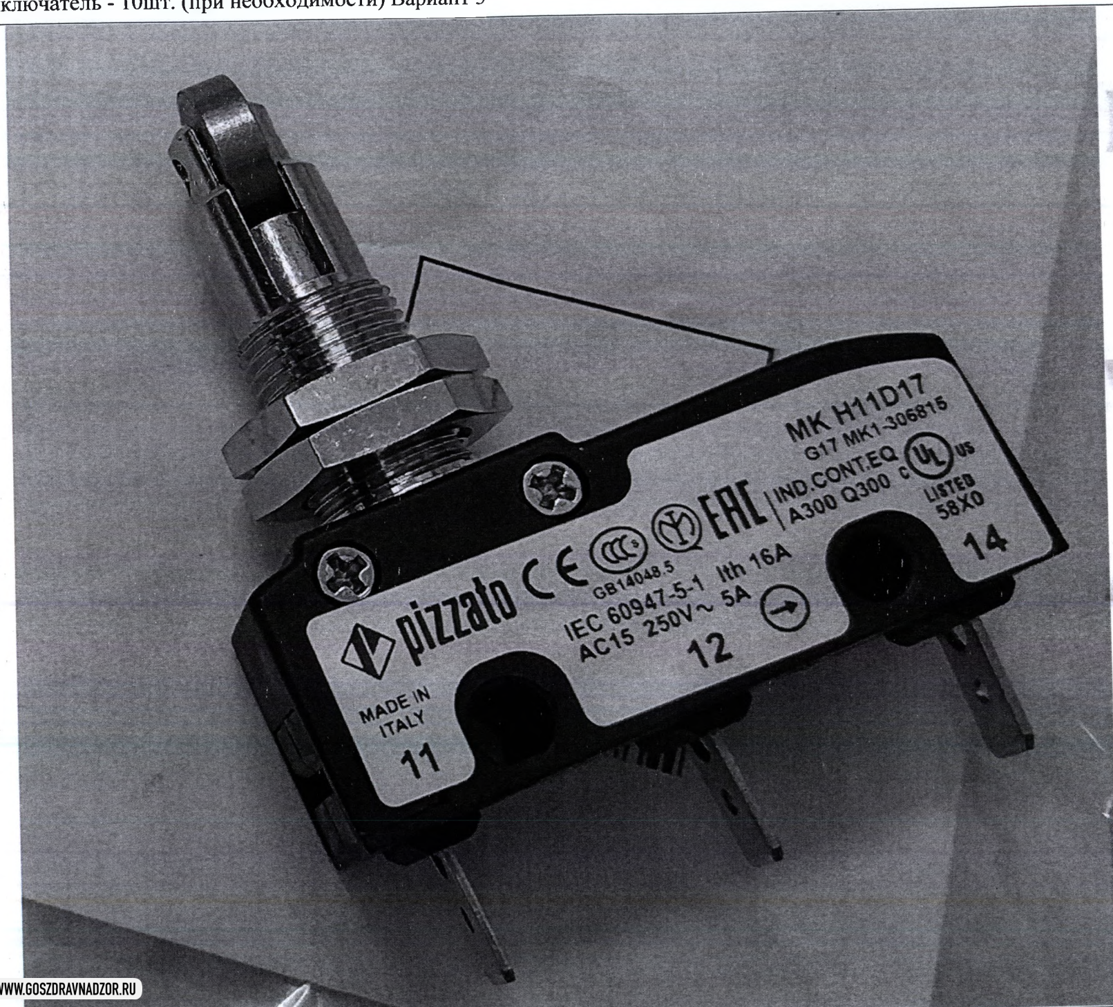
71. Микровыключатель - 10шт. (при необходимости) Вариант 3
