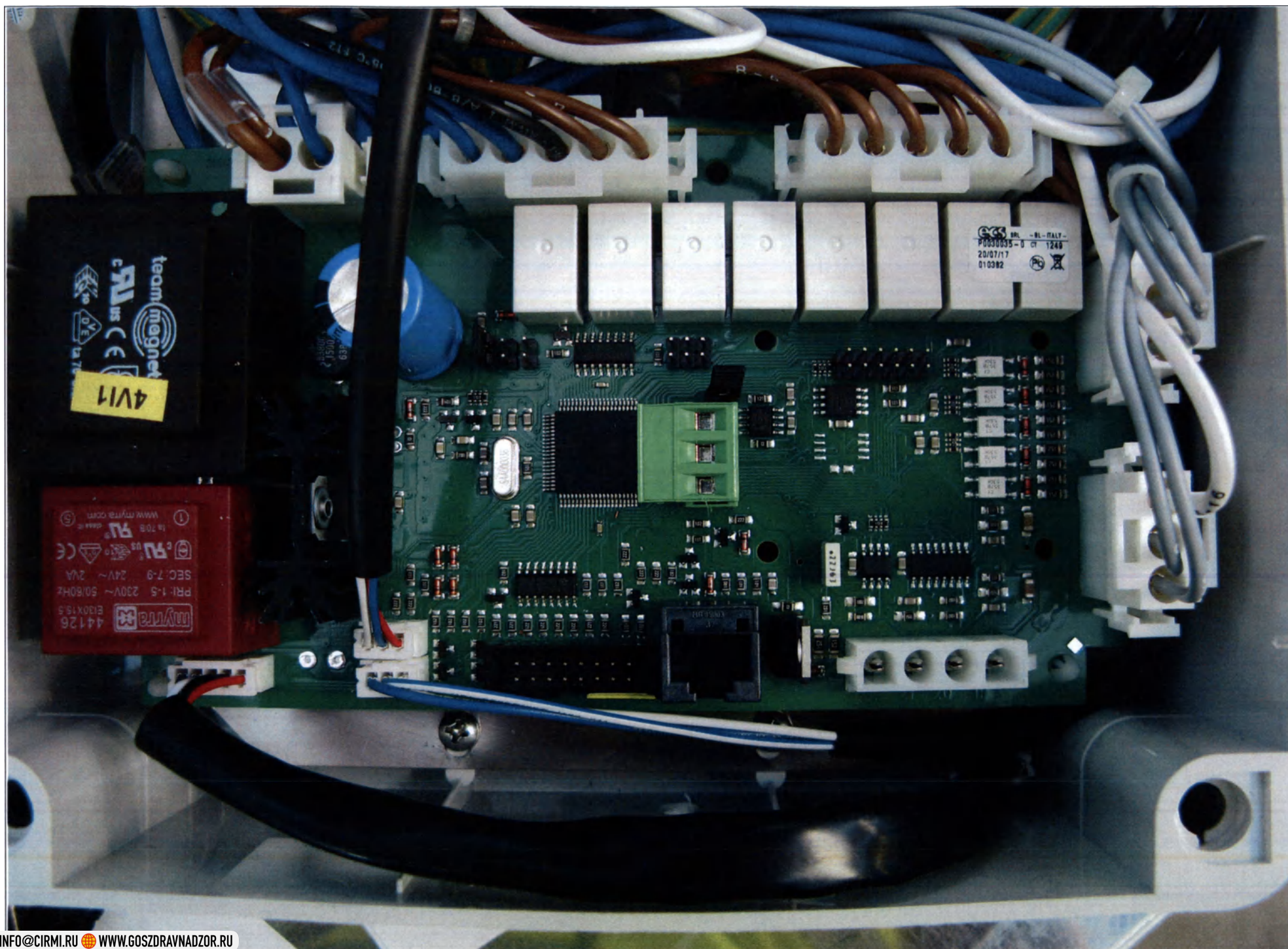
80. Плата управления МДМ-П 1М - 1шт.
