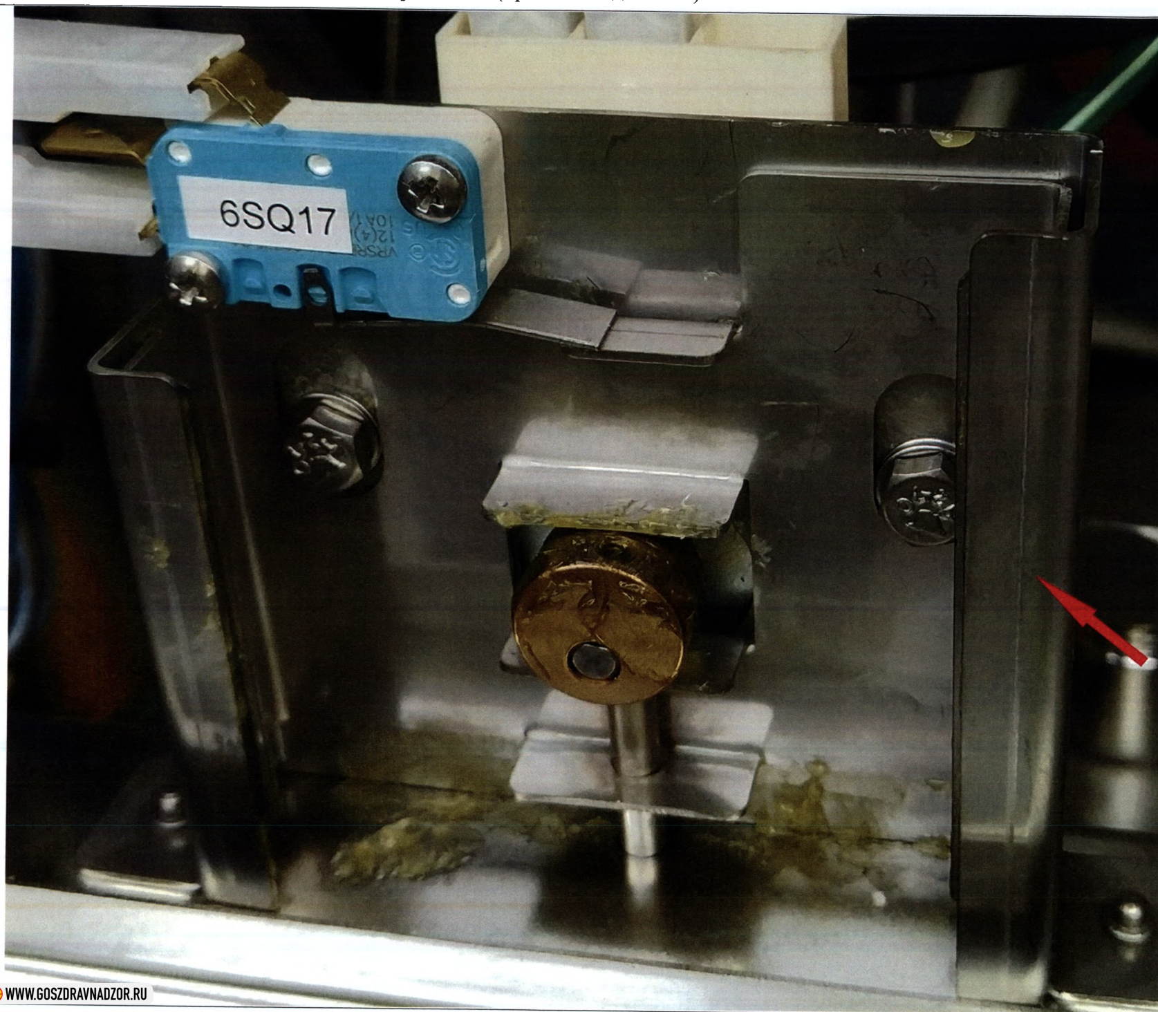
64. Кронштейн механизма блокировки двери камеры - 1 шт. (при необходимости)
