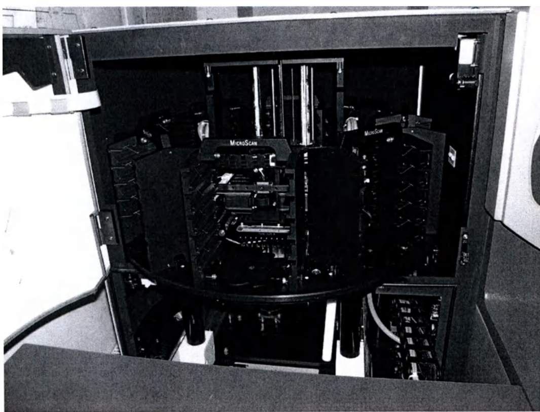
Отсек для установки панелей
