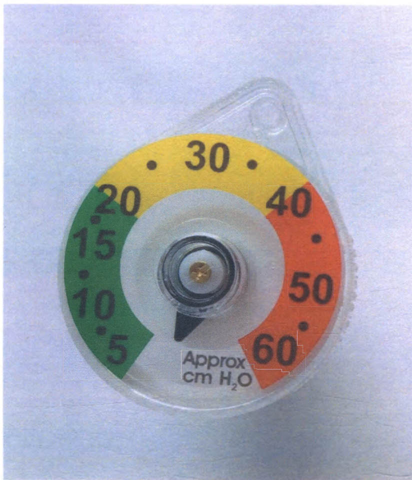
манометр от 0 до 60 см H 2 O
