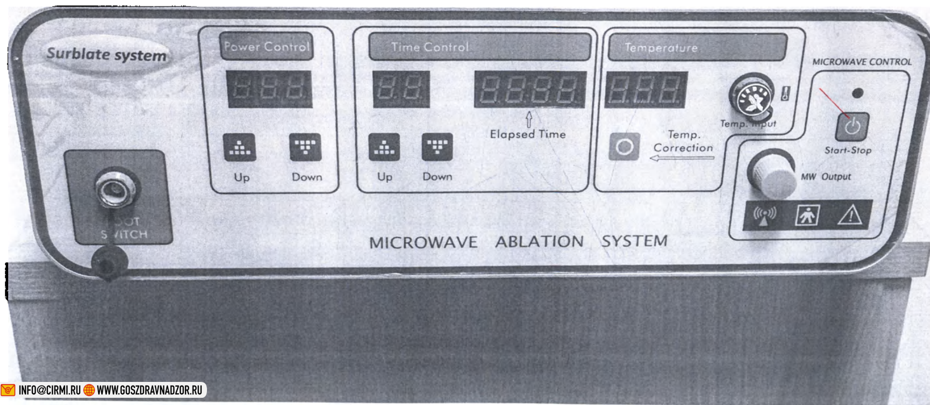
Рис. 1. Генератор (модель: МТС-3С). Вид спереди
