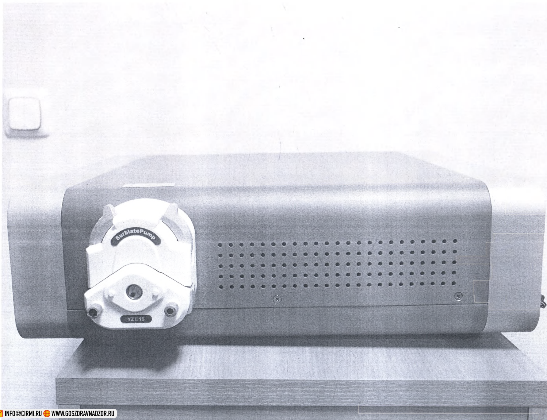
Рис. 2 Генератор (модель: МТС-3С). Вид сбоку
