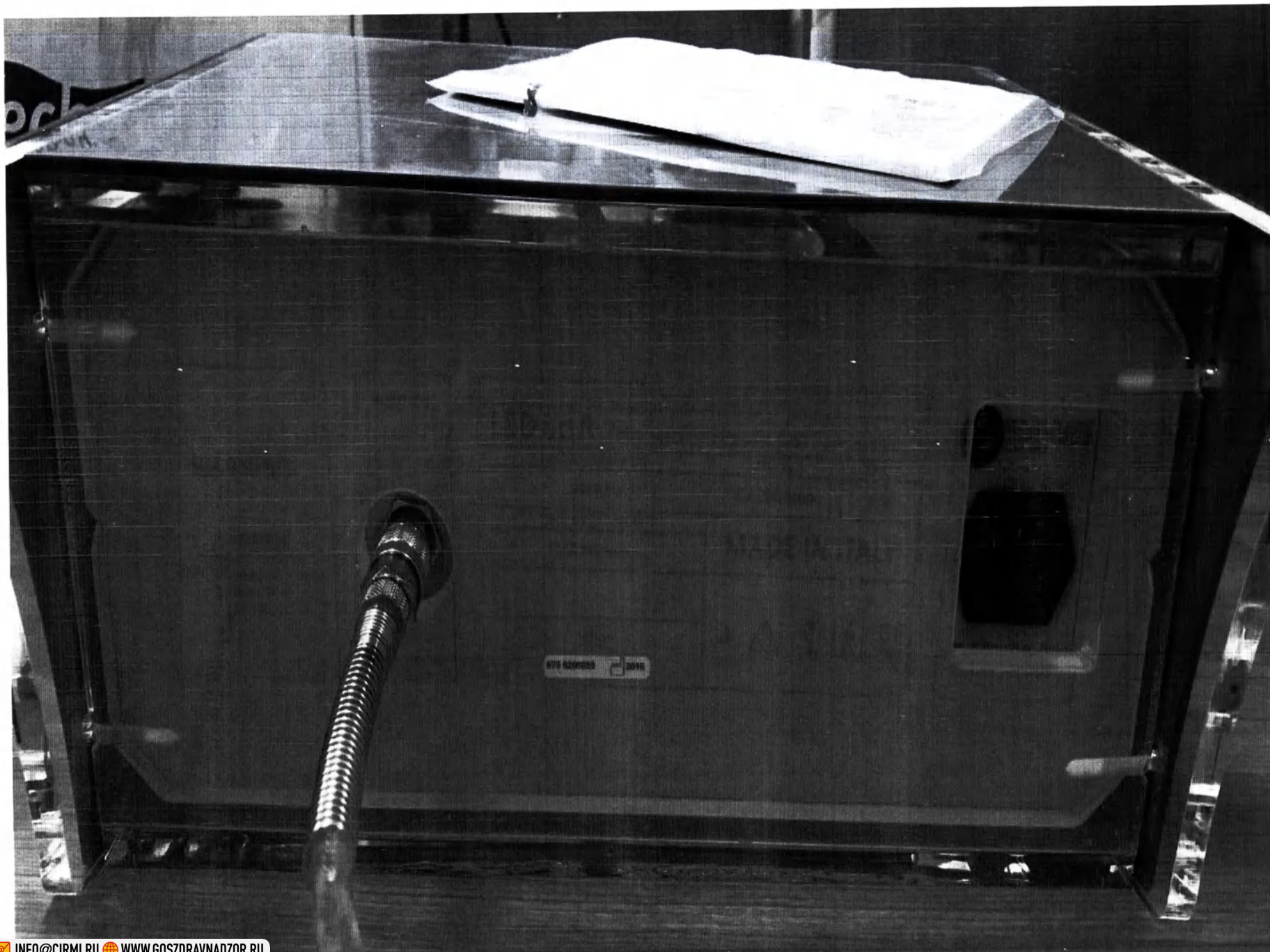
Рис.3. Аппарат для подкожных инъекций CO 2 CARBOMED. Фотографическое изображение задней части прибора.
