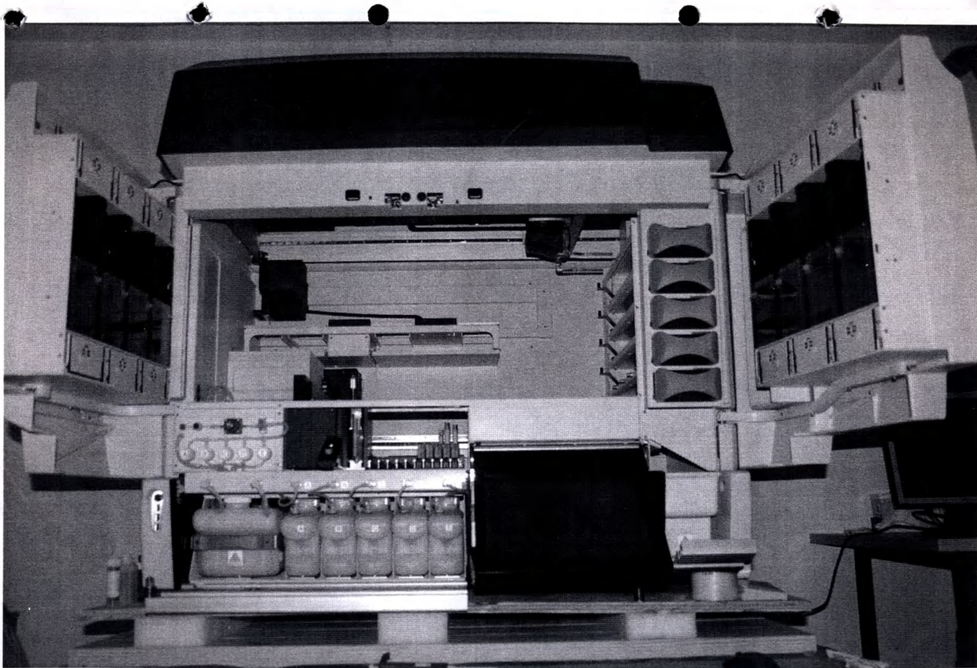
Фото 5. Сервисный режим: Открыты дверцы для доступа к органам управления и манипуляторам анализатора.
