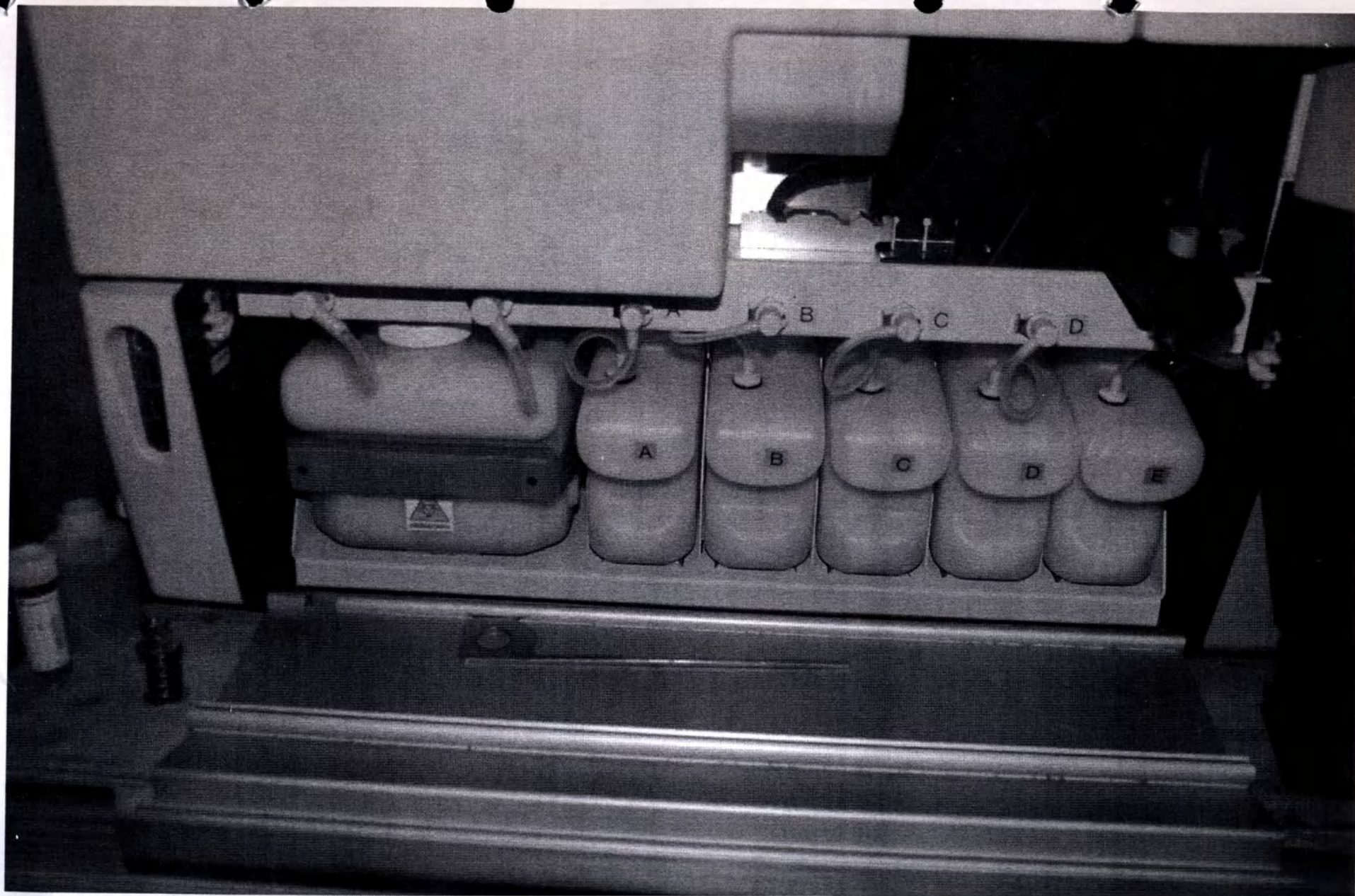
Фото 3. Отсек для размещения емкостей для промывочных растворов в открытом состоянии.
