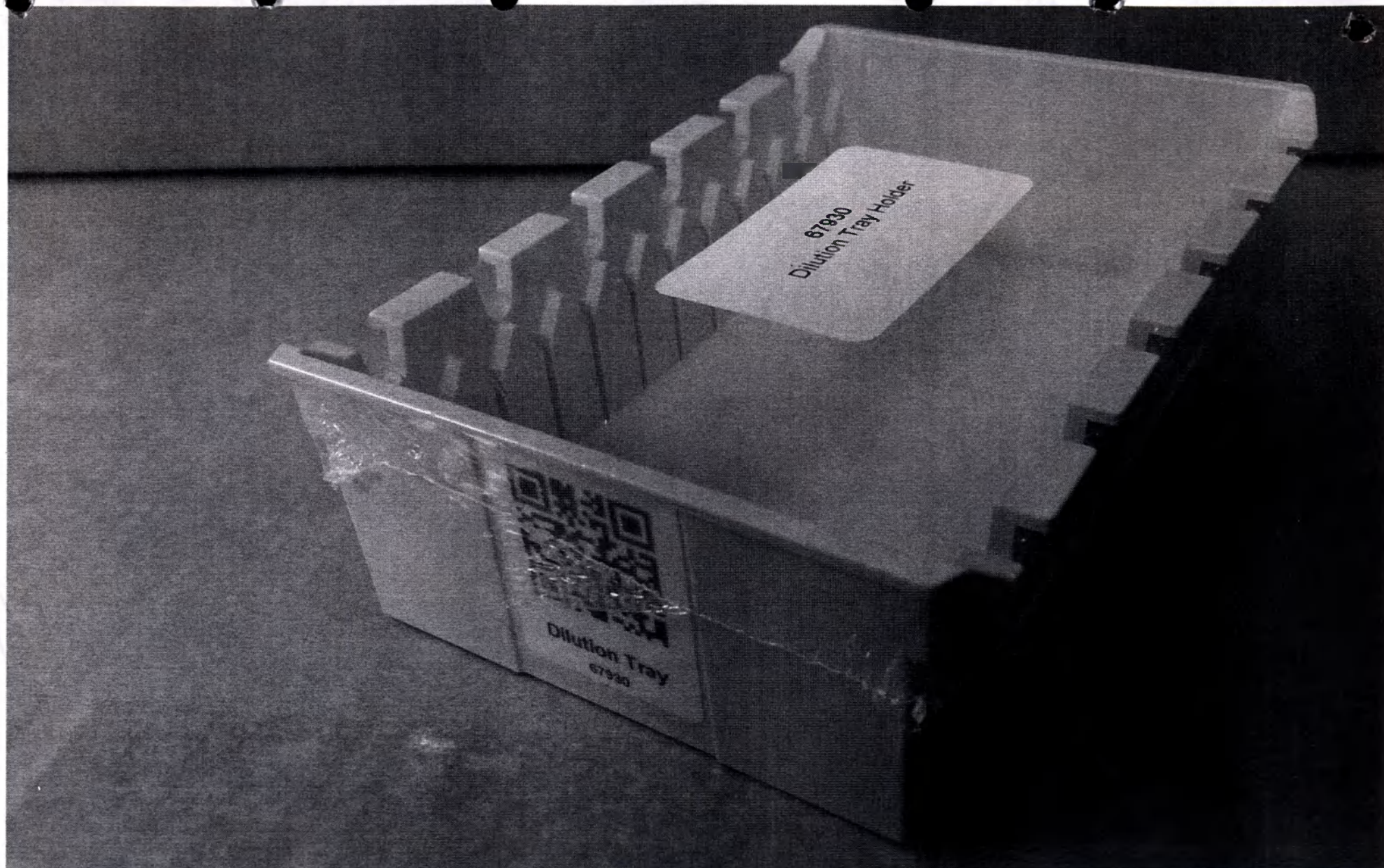
Фото 13. Картридж стрипов для разведения со штрих-кодом (Dilution Tray Holder With Barcode Label).
