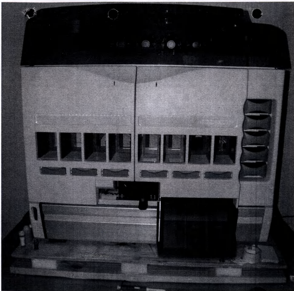
Фото 1. Общий вид анализатора иммуноферментного автоматического «Чаройт»
