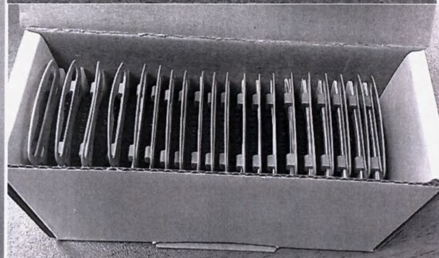
Фильтры для защиты от серы HF4 Pro со вспомогательным инструментом и кратким руководством правый (красный) – 10 шт./ левый (синий) – 10 шт. (HF4 Pro – Filter Red/ Blue 20) – 20 шт./уп.
