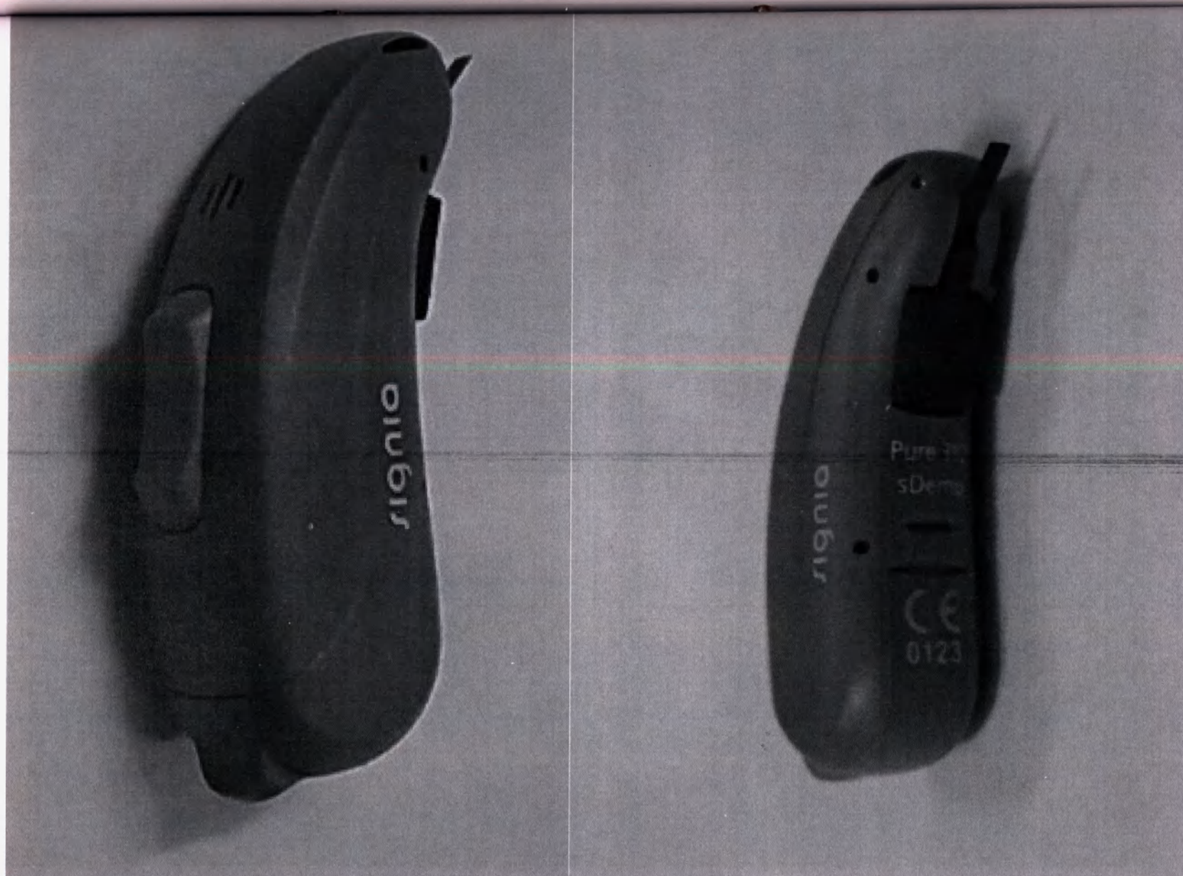
Аппарат слуховой цифровой Pure 312 sDemo DNx
