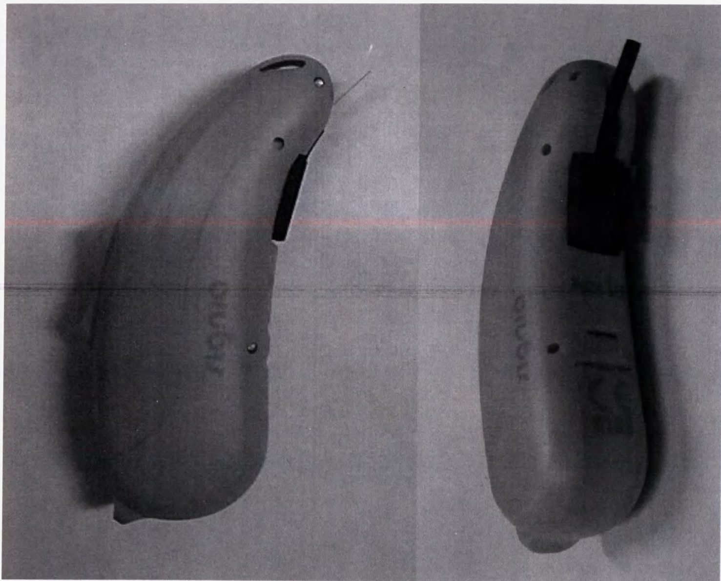
Аппарат слуховой цифровой Pure 312 5Nx.
