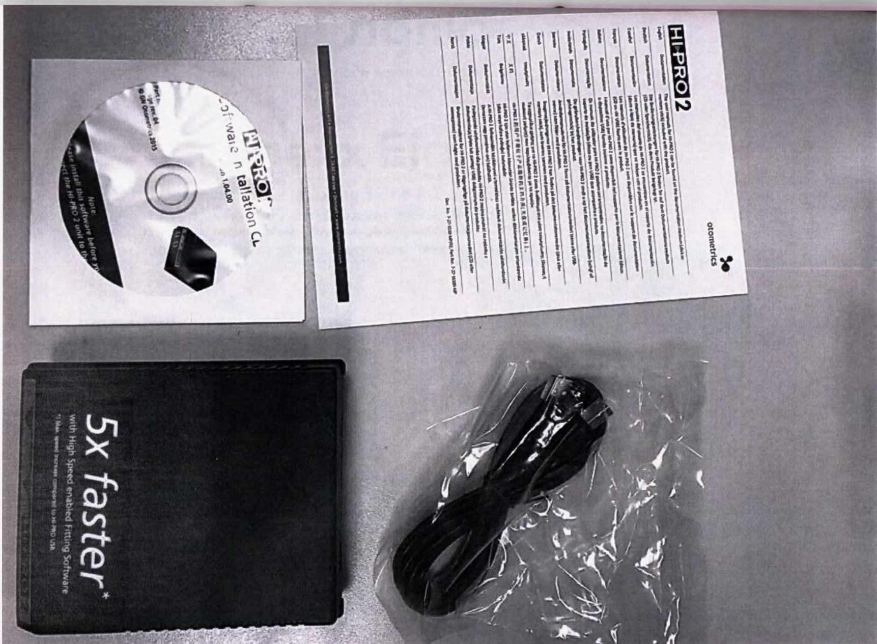
Программатор Hi-PRO 2 USB в комплекте: основное устройство Hi-PRO 2, USB-кабель, установочный компакт диск, руководство по установке
