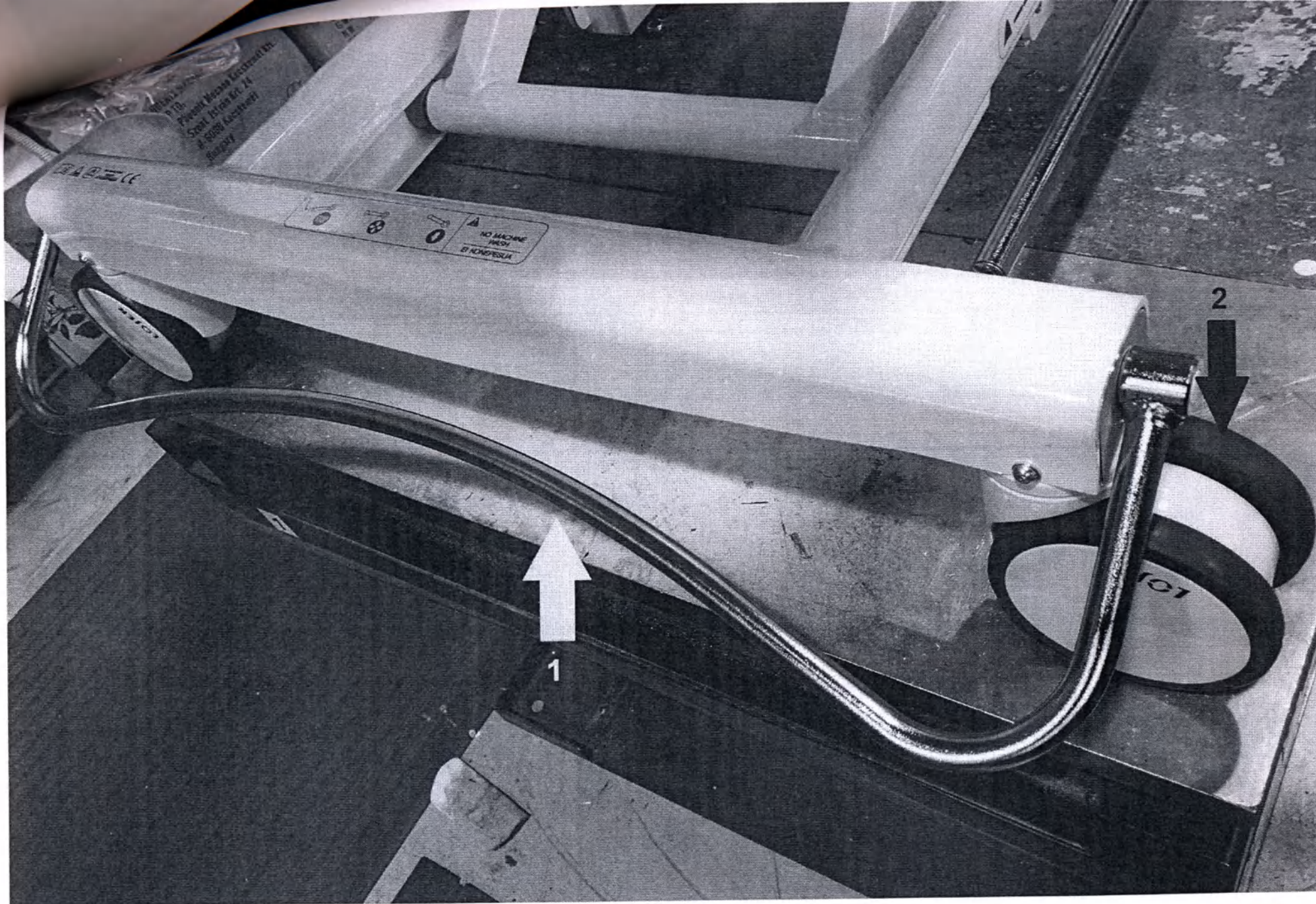
Колесо с центральной блокировкой: 1 – педаль центральной блокировки, 2 – колесо (внешний вид колеса, диаметром 125 мм, и колеса, диаметром 150 мм, совпадает)
