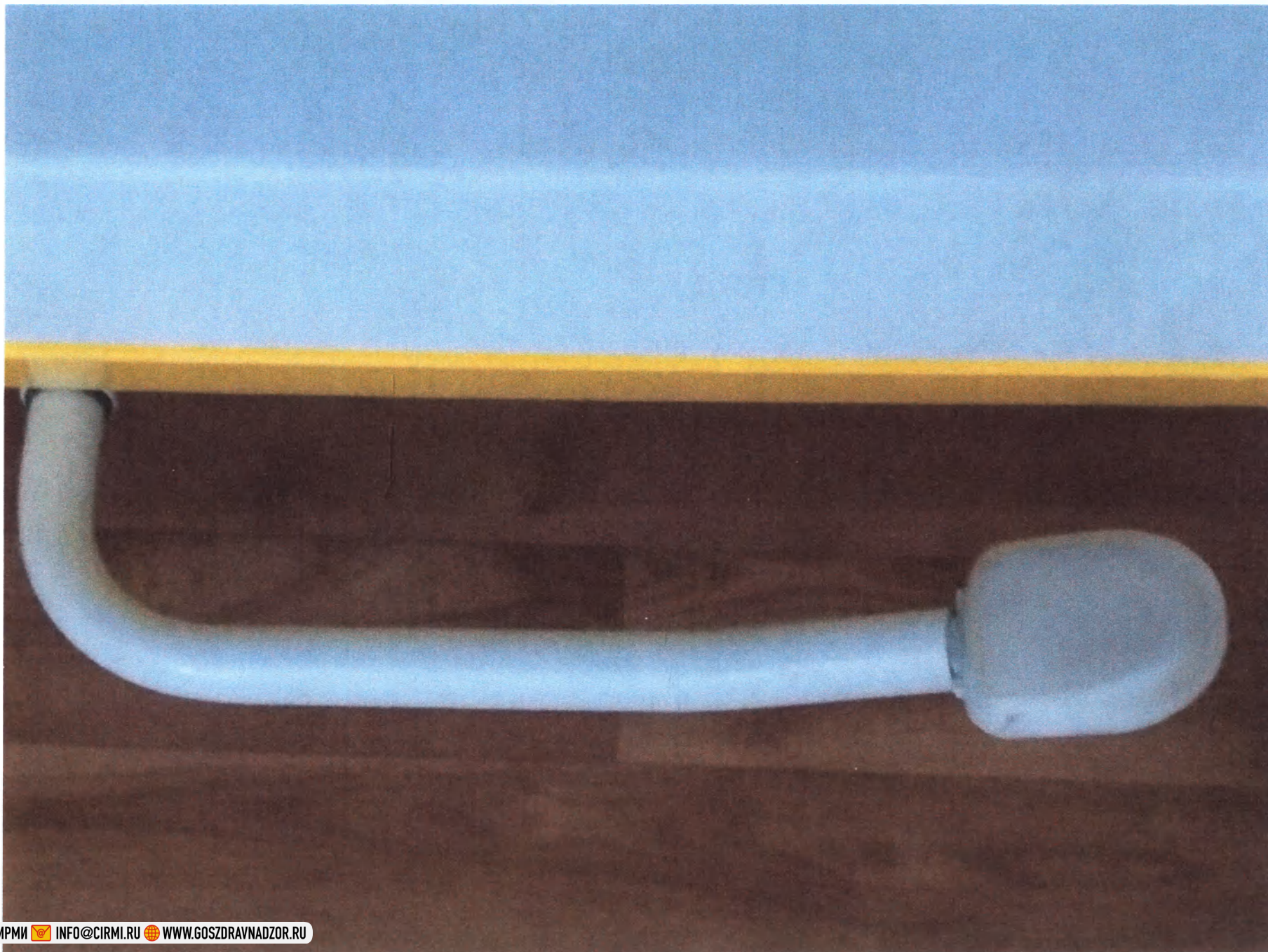
Фото 3.7. Педаль управления выдвижным пятым колесом.
