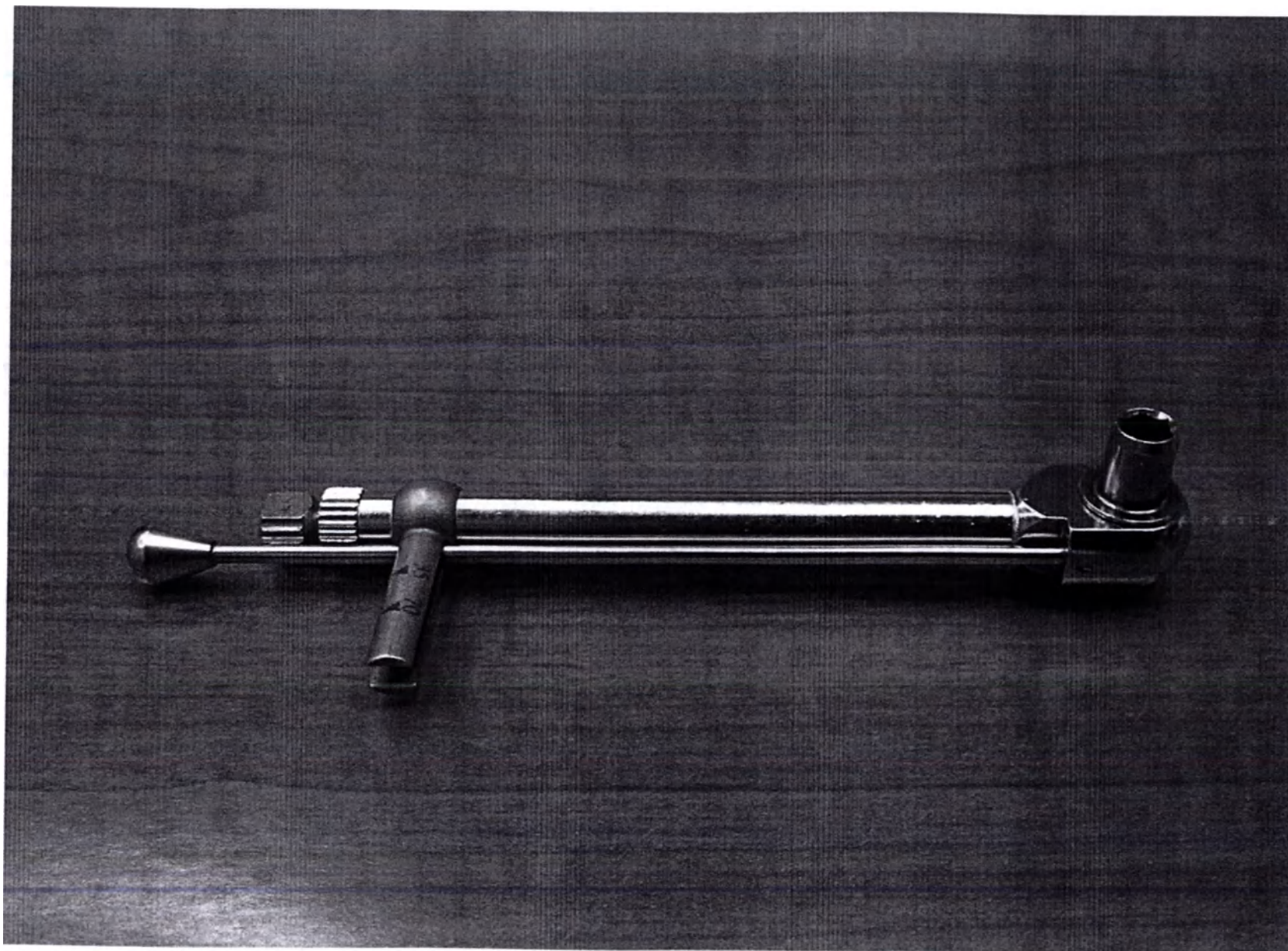
ной хирургический динамометрический ключ NobelActive Manual Torque Wrench Surgical
