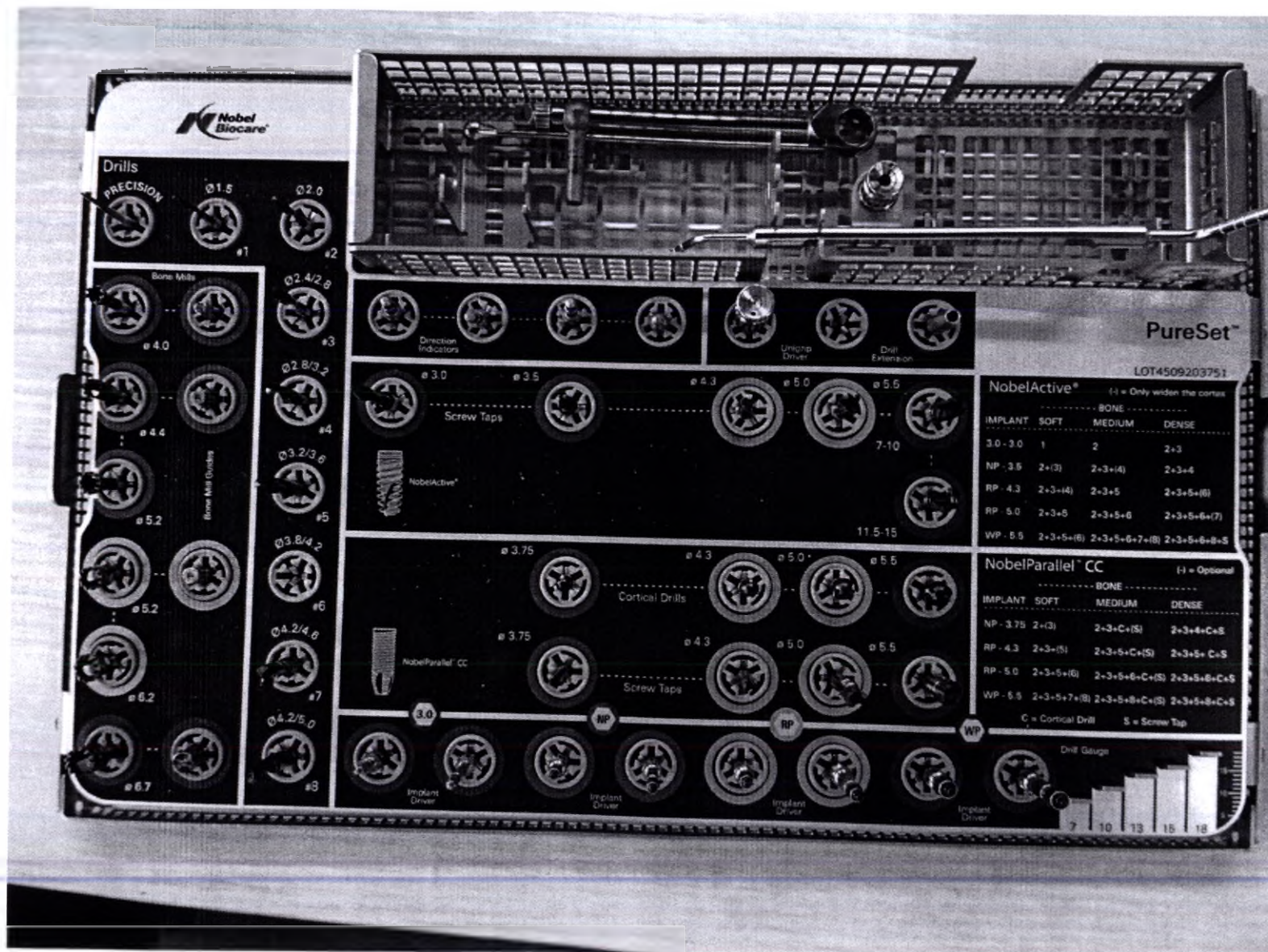
ок хирургического набора NobelActive/NobelParallel CC (NobAct/NobPrl CC) PureSet Tray
