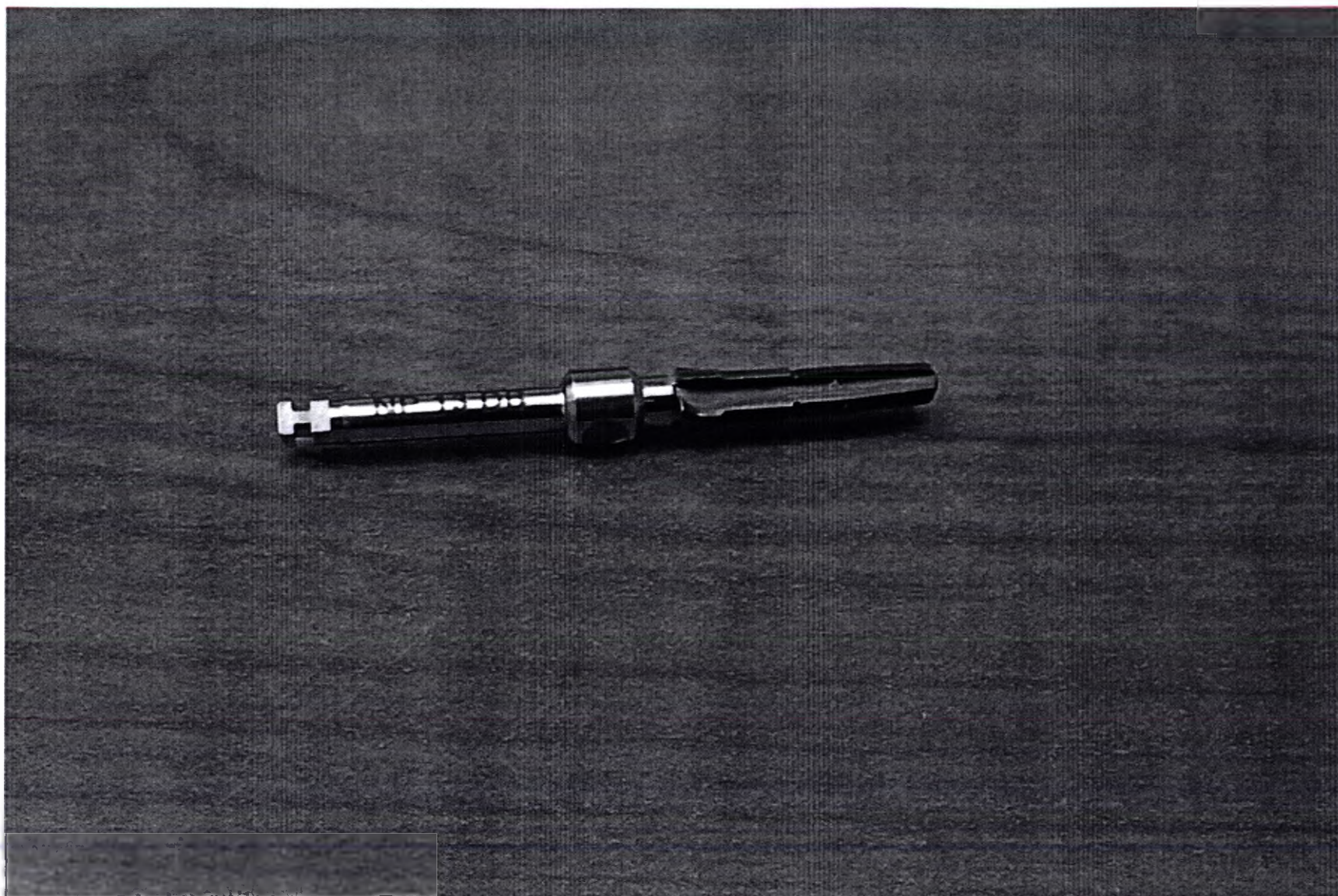
ерло Drill Tapered 3,5 x 13 мм
