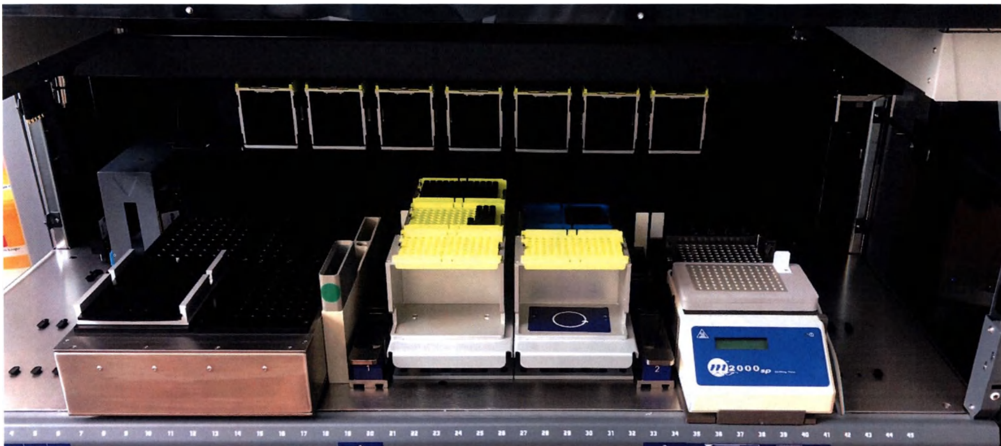
4. Рабочий стол прибора m2000sp (m2000sp Worktable Kit).
