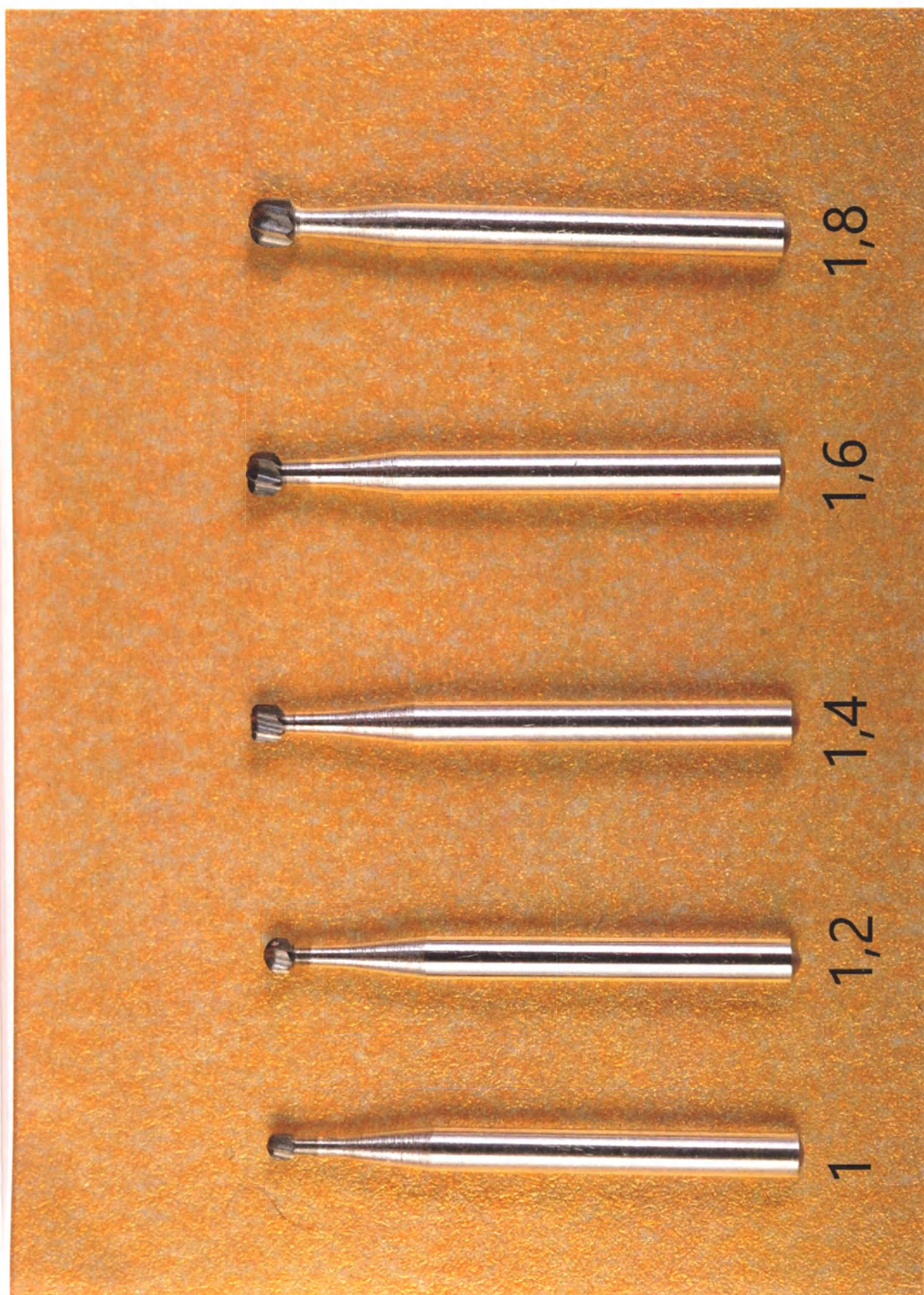
Рис. 1 Общий вид. Бор твердосплавный турбинный «шарик». БТТ-1; БТТ-1,2; БТТ-1,4; БТТ-1,6; БТТ-1,8
