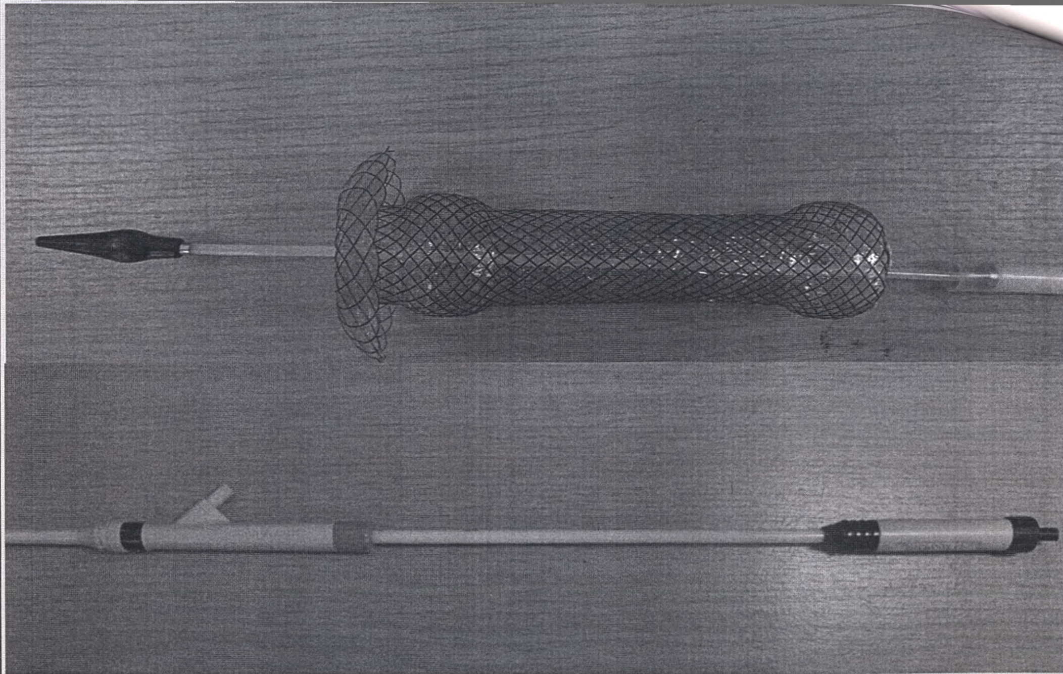
Фото 5 - Стент пищеводный для кардиального отдела желудка с частичным покрытием. Общий вид
