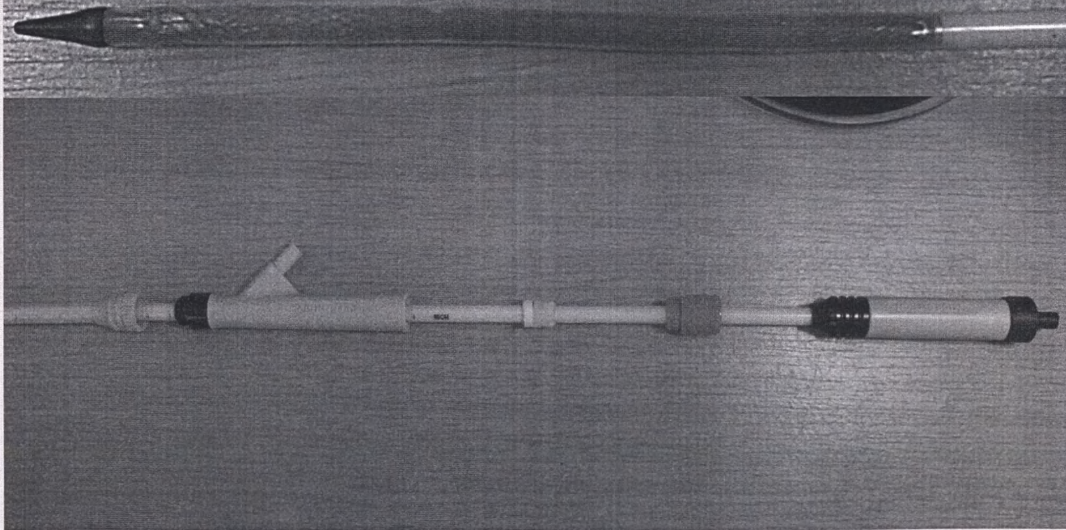
Фото 7 - Стент пищеводный для кардиального отдела желудка с покрытием по всей длине. Общий вид
