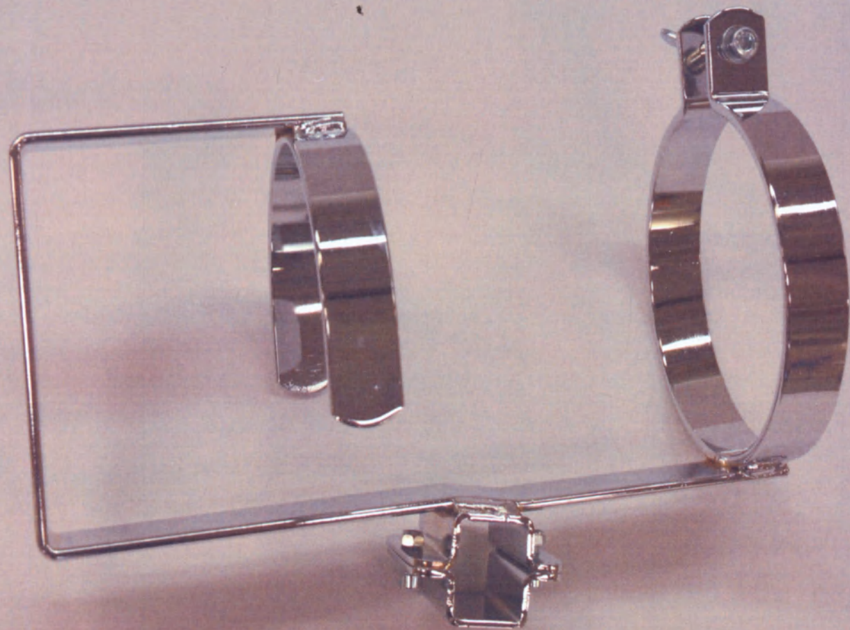
Держатель кислородного баллона 589
