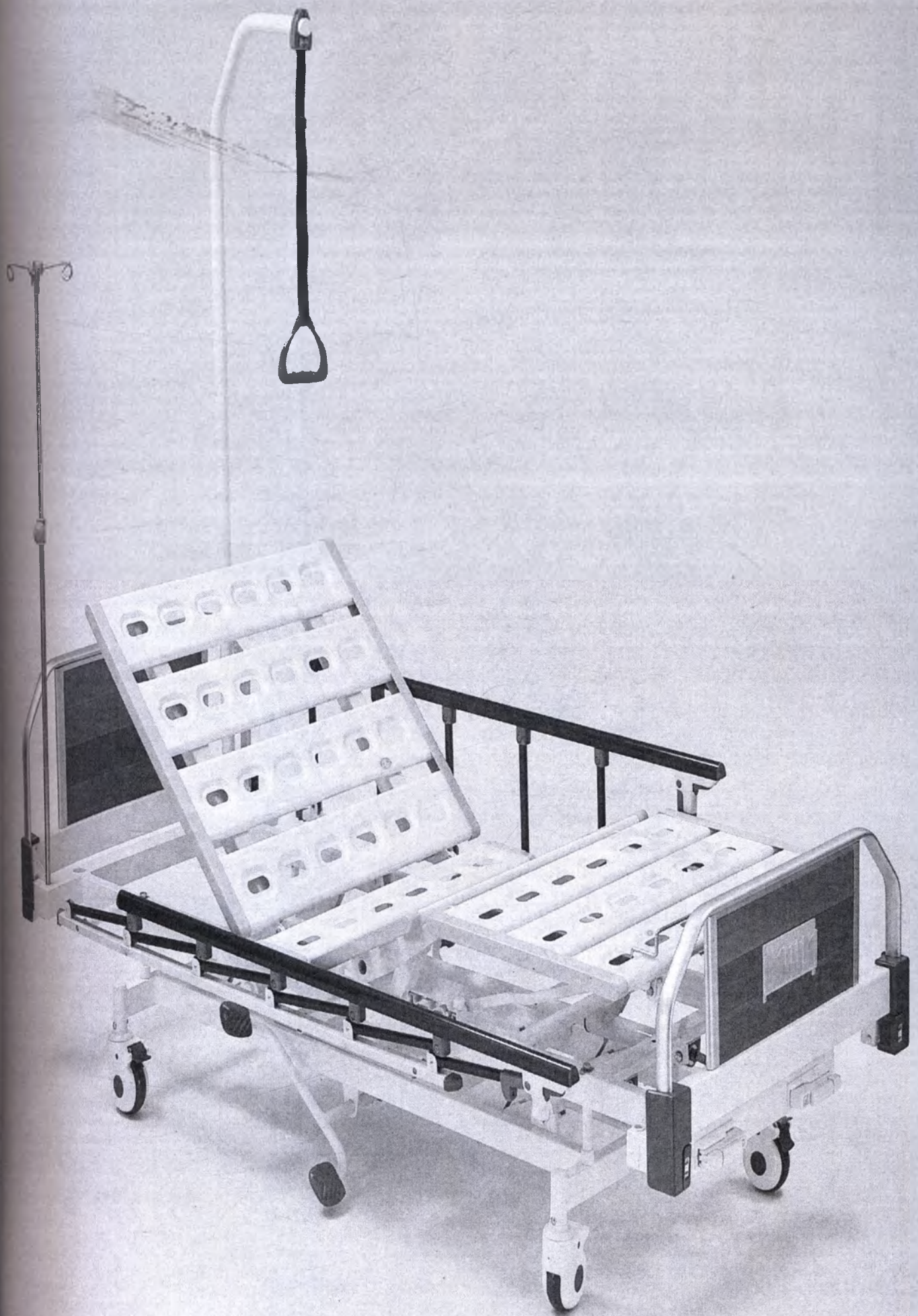
Кровать медицинская функциональная «Armed», вариант исполнения SAE-104-F
