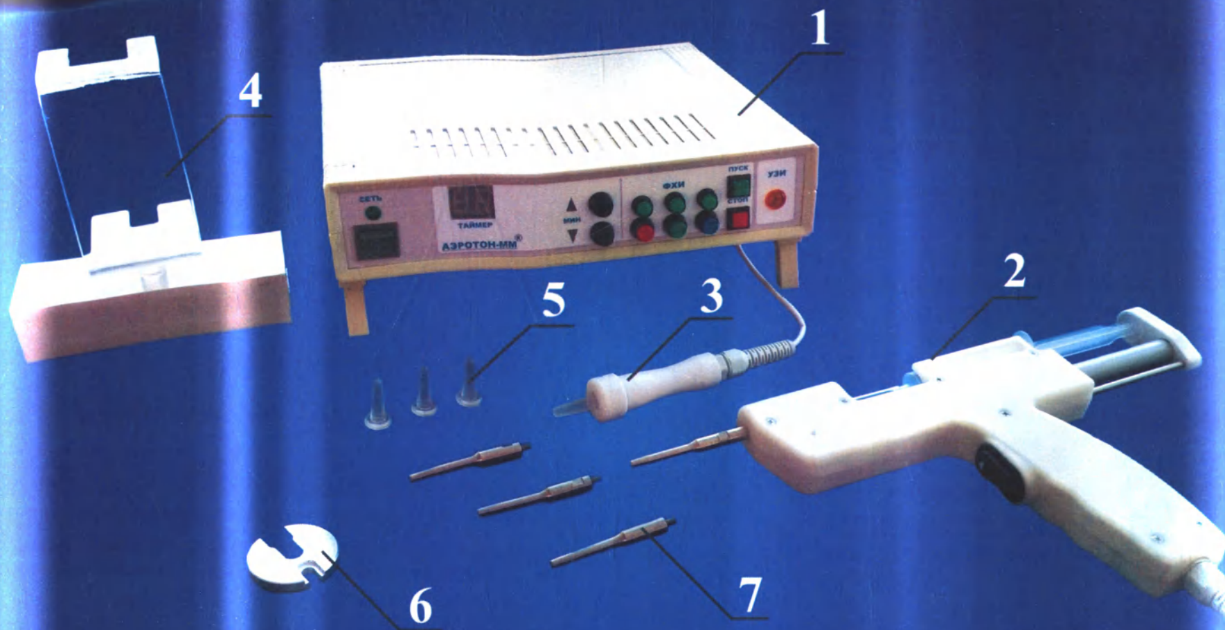
1 - блок управления; 2 - ультразвуковой инжектор; 3 - аппликатор фотохромный; 4 - держатель инжектора; 5 - насадка; 6 - ключ; 7 - волновод-инструмент
