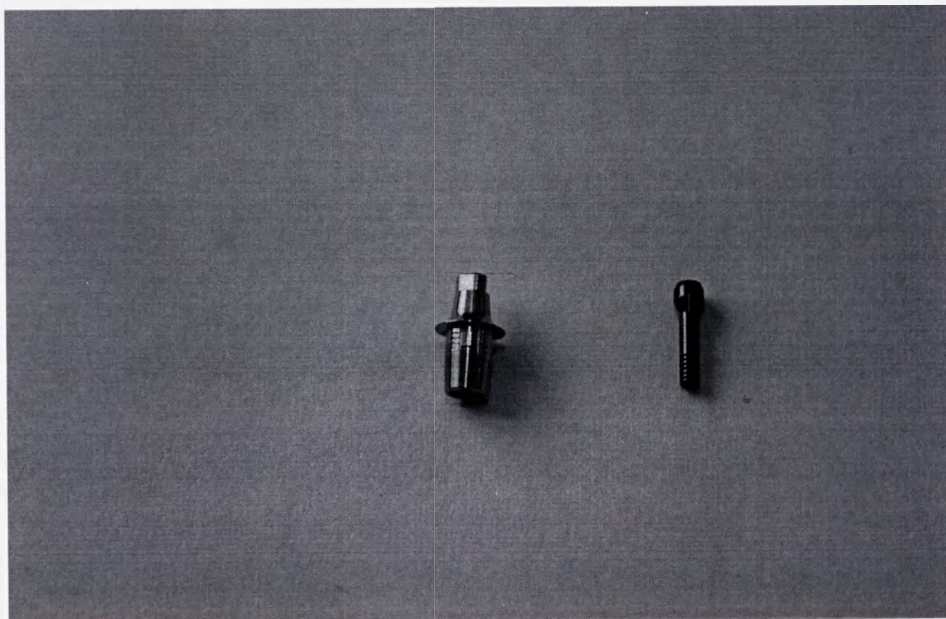
Абатмент AXIOM Tibase C/L BL, с винтом
