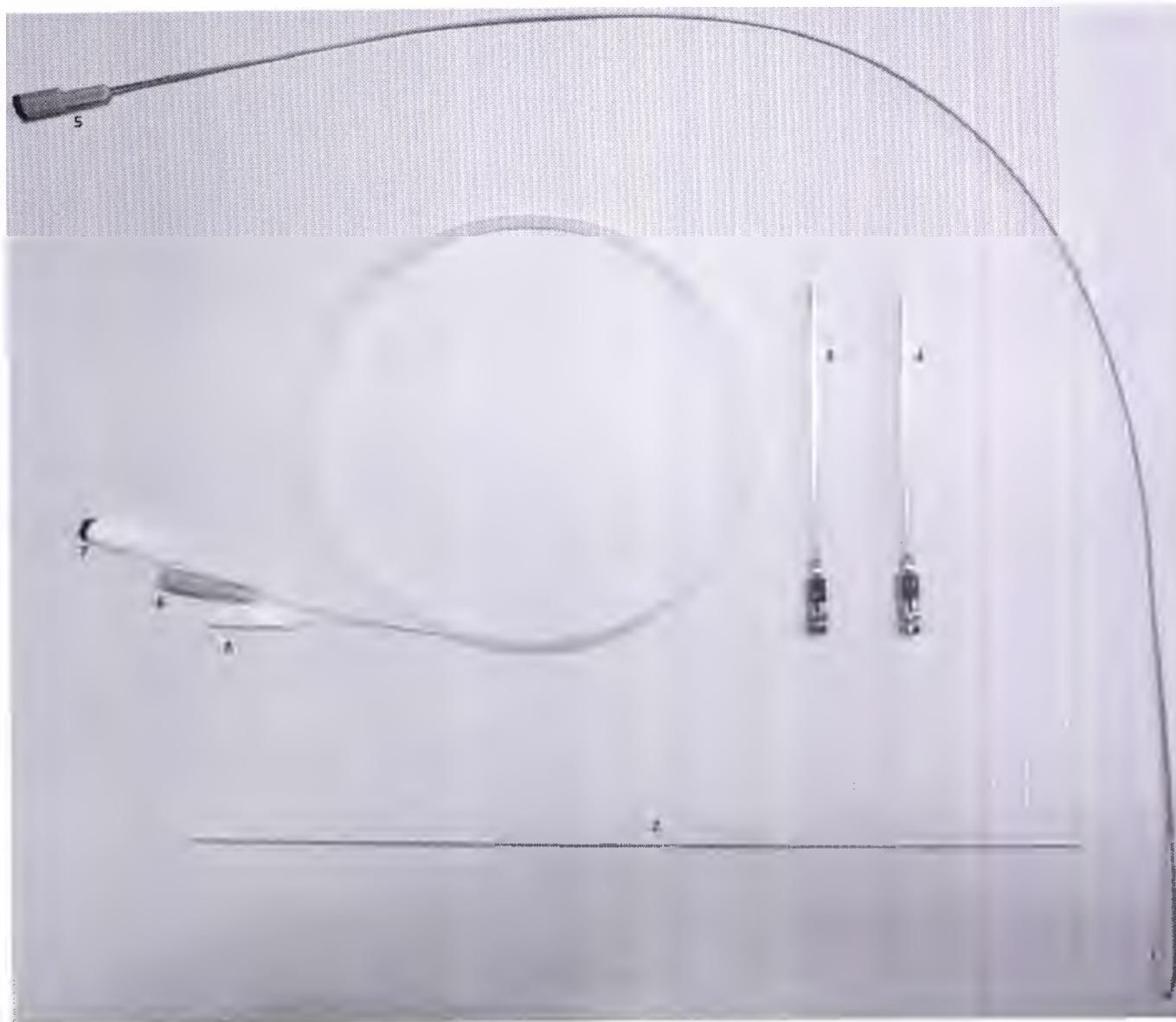
Набор электрода для пробного скрининга Vectris 1x8 Subcompact для стимуляции спинного мозга (SCS). варианты исполнения 977D160. 977D260 (комплект поставки).
