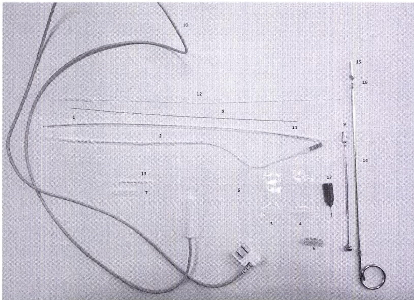
Набор с электродом для стимуляции спинного мозга и стимуляции периферических нервов PISCES-QUAD PLUS, модели 3888, варианты исполнения 3888-33, 3888-45, 3888-56 (комплект поставки).
