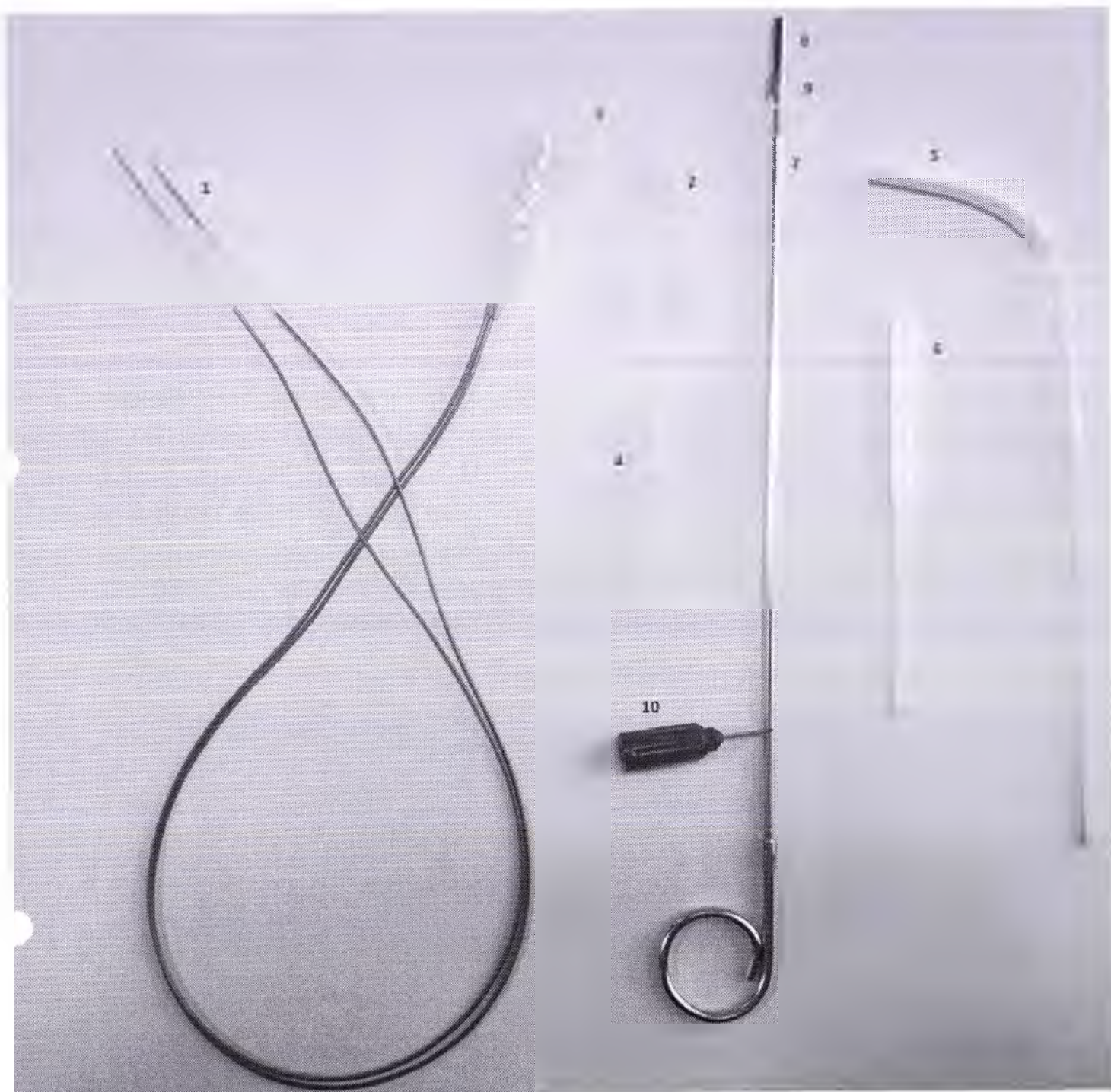
Набор электрода Specify SureScan MRI 2x8, варианты исполнения 977C265, 977C290 (комплект поставки).
