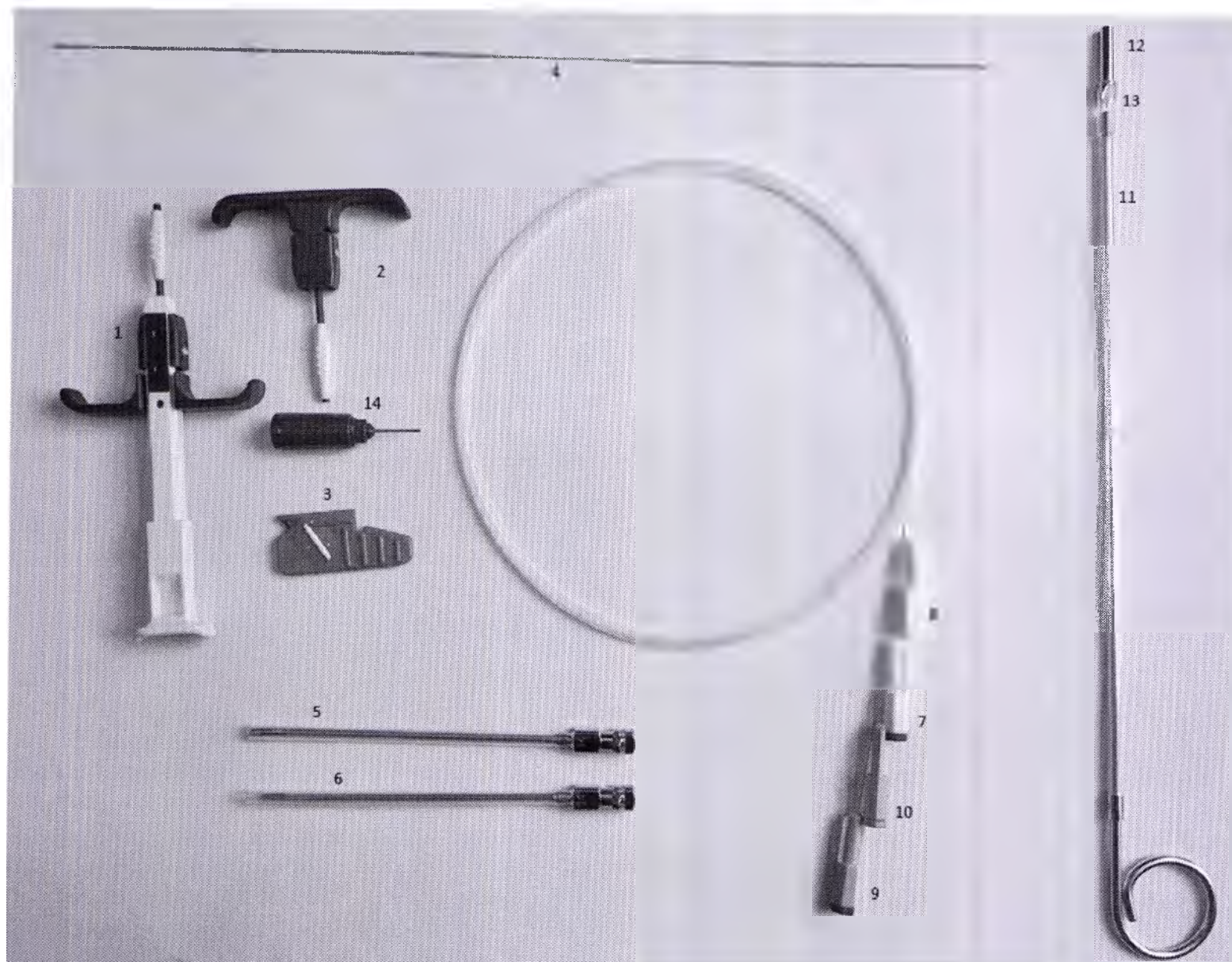
Набор принадлежностей для ревизии для чрескожных электродов Vectris SureScan MRI 1x8, модель 97790, варианты исполнения 97790-60, 97790-75, 97790-90 (комплект поставки).
