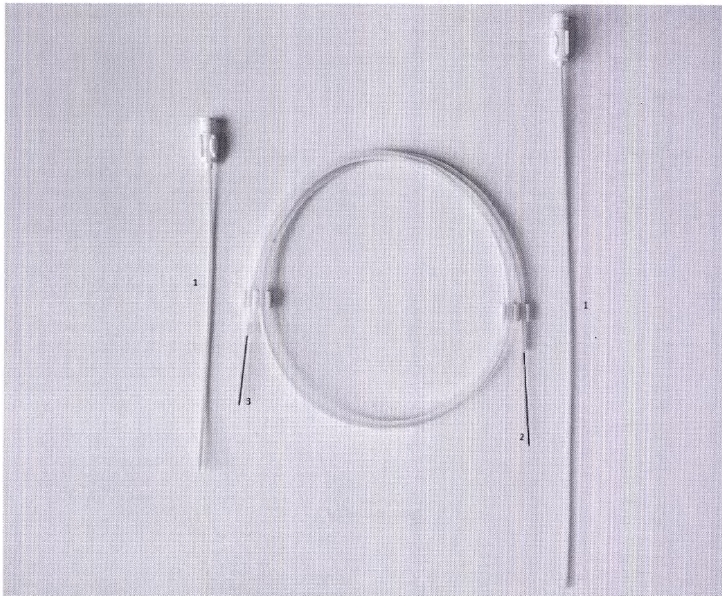
Интродьюсер для чрескожного электрода, модель 3550-63.
