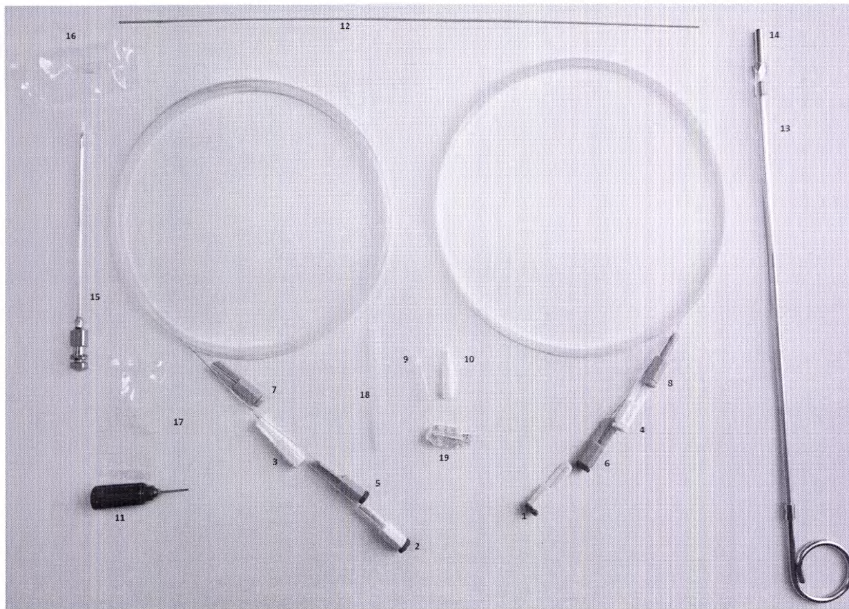
Набор принадлежностей для контроля электрода 1х8, модель 3550-27 (комплект поставки).
