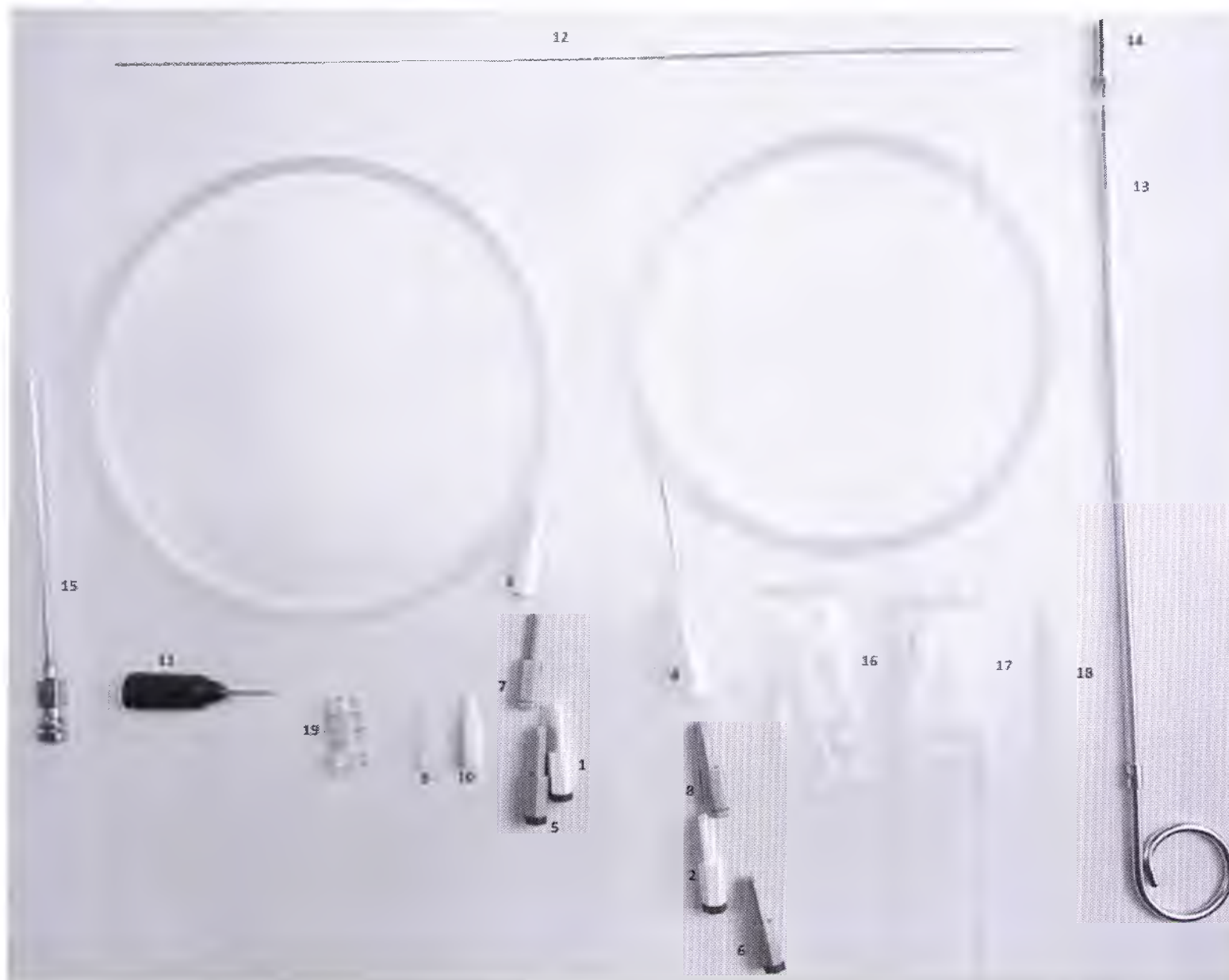
Набор принадлежностей для контроля электрода 1х8, модель 3550-26 (комплект поставки).
