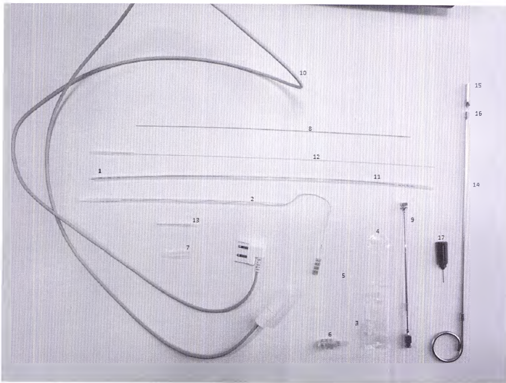
Набор с электродом для стимуляции спинного мозга и стимуляции периферических нервов PISCES-QUAD, модели 3487A, варианты исполнения 3487A-33, 3487A-45, 3487A-56 (комплект поставки).
