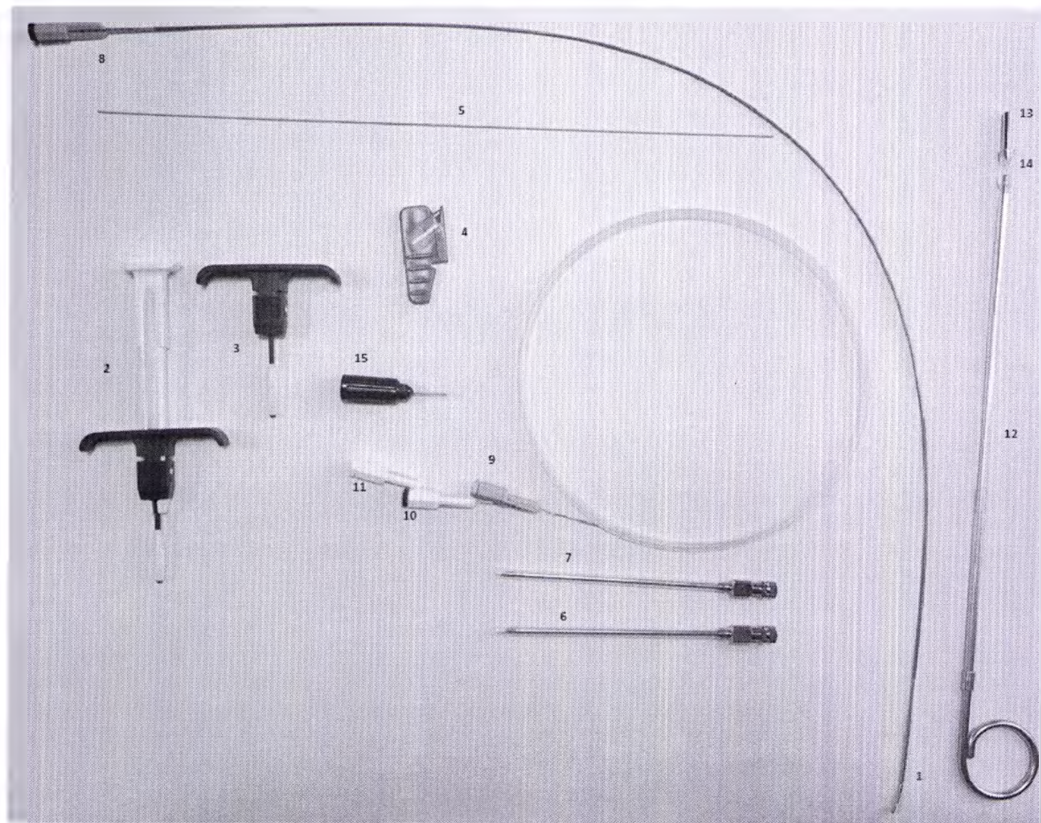
Набор для стимуляции спинного мозга Vectris SureScan MRI 1x8 Subcompact, варианты исполнения 977A160, 977A175, 977A190 (комплект поставки).
