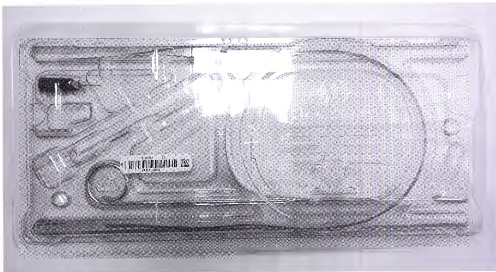
Набор электрода Specify SureScan MRI 2x8, варианты исполнения 977C265, 977C290 (стерильная упаковка).
