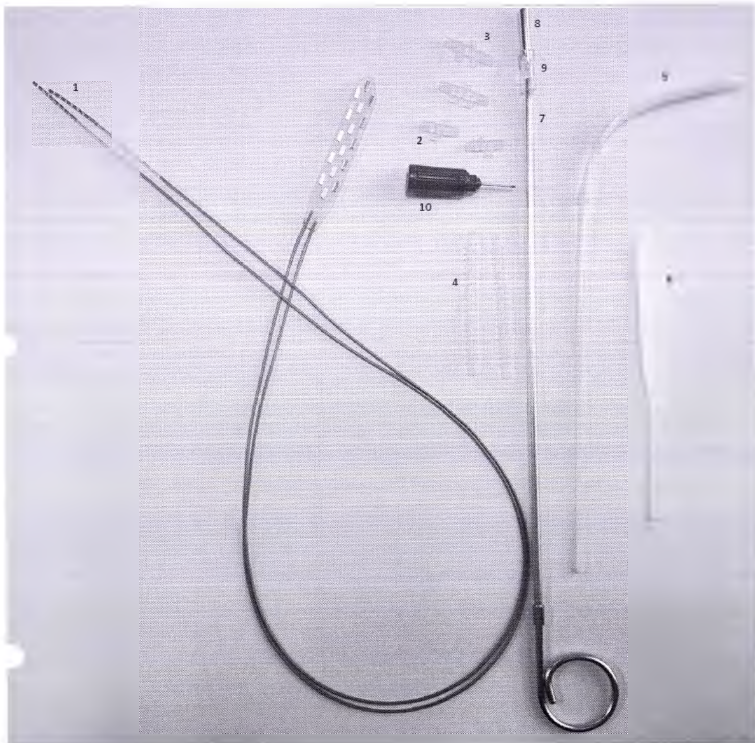
Набор электрода Specify SureScan MRI 5-6-5. варианты исполнения 977C165, 977C190 (комплект поставки).
