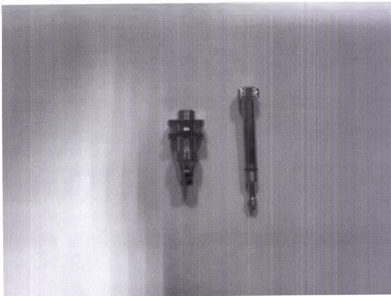
Трансфер для открытой ложки Impression Coping Open Tray Conical Connection (CC) в комплекте с винтом и кольцом O-Ring, типоразмер RP, размер 5x10 мм
