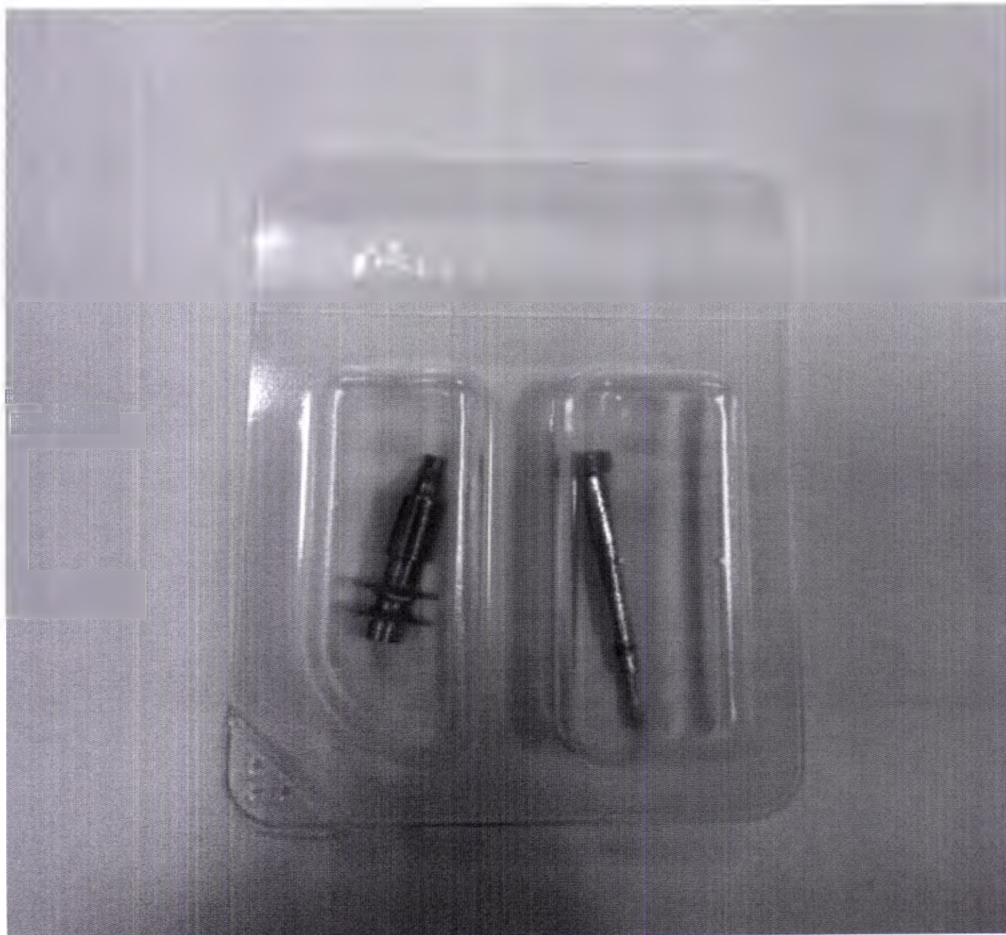
Трансфер для открытой ложки Impression Coping Open Tray Conical Connection (CC) в комплекте с винтом и кольцом O-Ring, типоразмер NP, размер 5x14 мм
