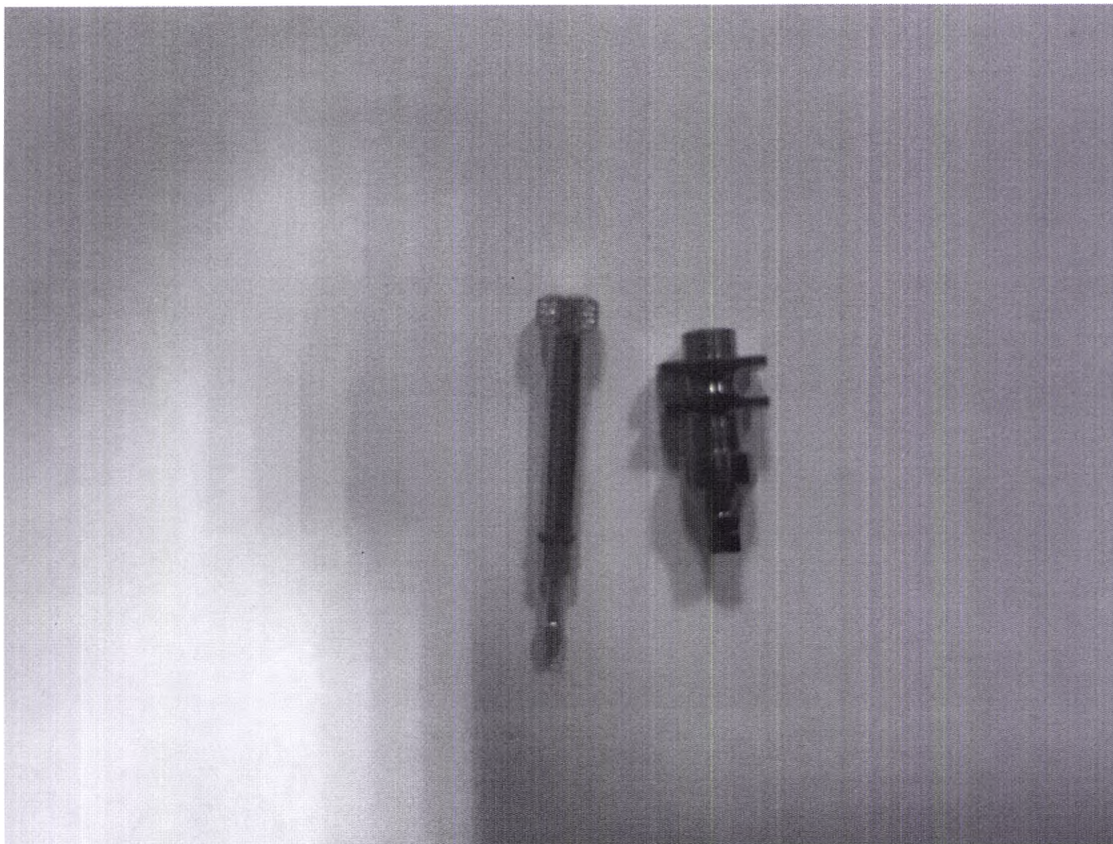
Трансфер для открытой ложки Impression Coping Open Tray Conical Connection (CC в комплекте с винтом и кольцом O-Ring, типоразмер NP, размер 5x10 мм
