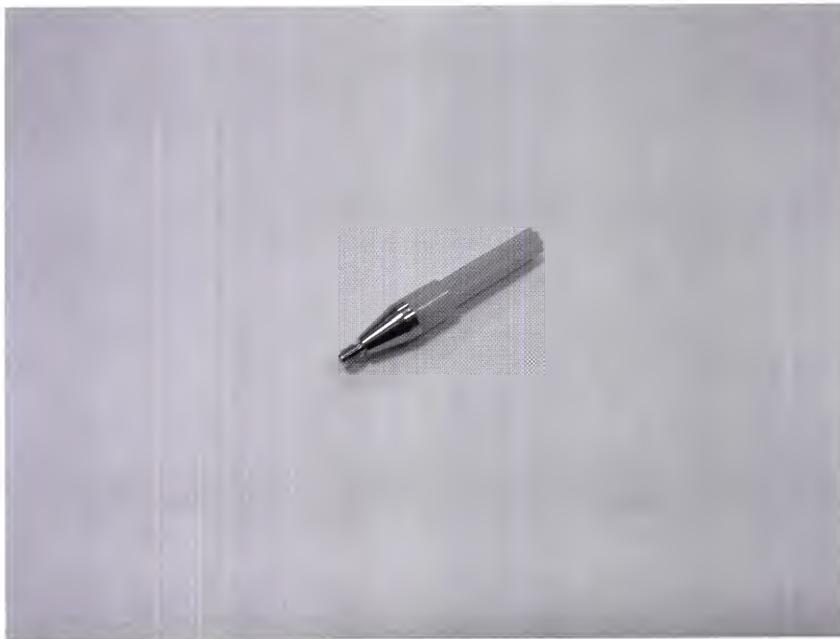
Абатмент Multi-unit Abutment Plus Conical Connection (CC), типоразмер RP, длина 4.5 мм, в комплекте с держателем
