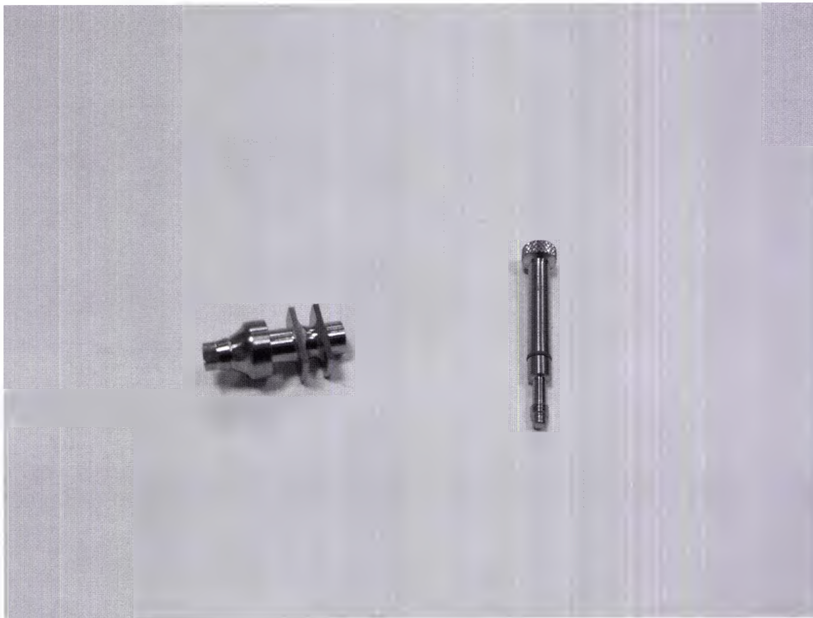
Трансфер для открытой ложки Impression Coping Open Tray Conical Connection (CC) в комплекте с винтом и кольцом O-Ring, типоразмер RP, размер 6x10 мм
