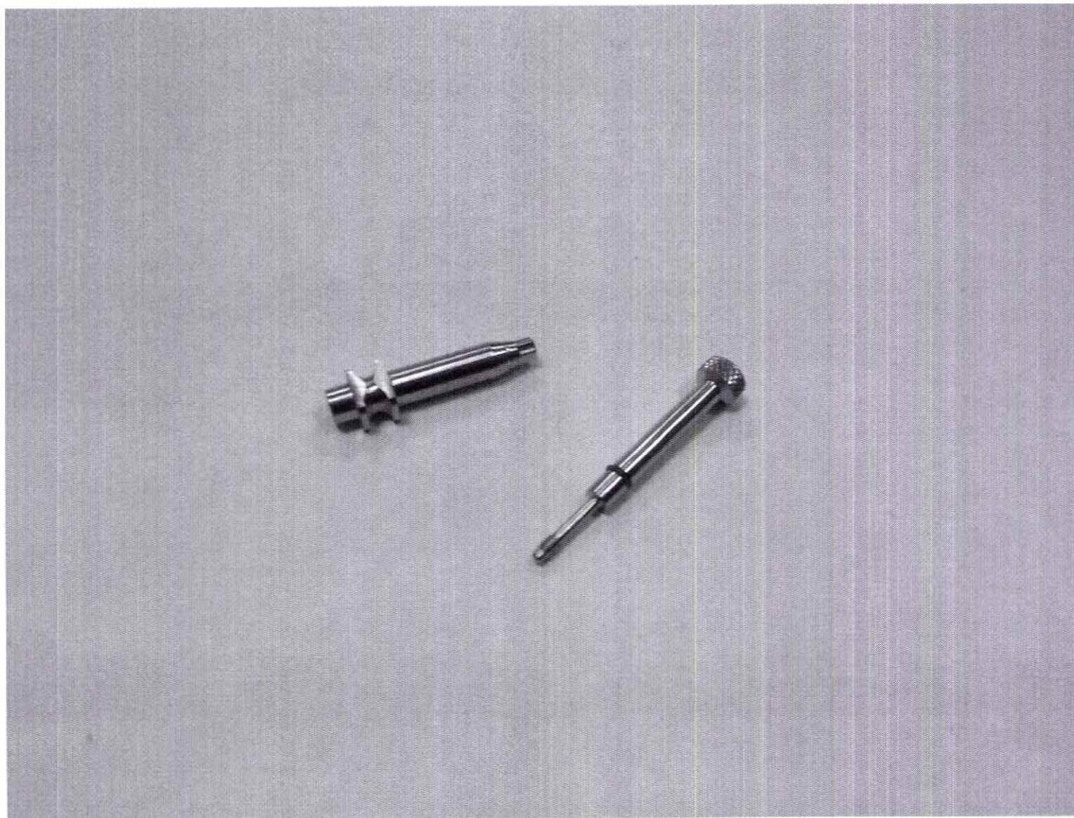
Трансфер для открытой ложки Impression Coping Open Tray Conical Connection (CC) в комплекте с винтом и кольцом O-Ring, типоразмер 3.0, размер 3.2x14 мм
