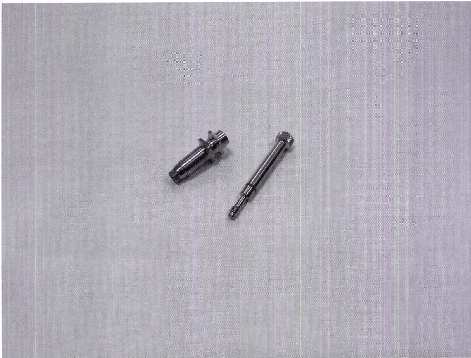
Трансфер для открытой ложки Impression Coping Open Tray Conical Connection (CC в комплекте с винтом и кольцом O-Ring, типоразмер RP, размер 3.6x10 мм
