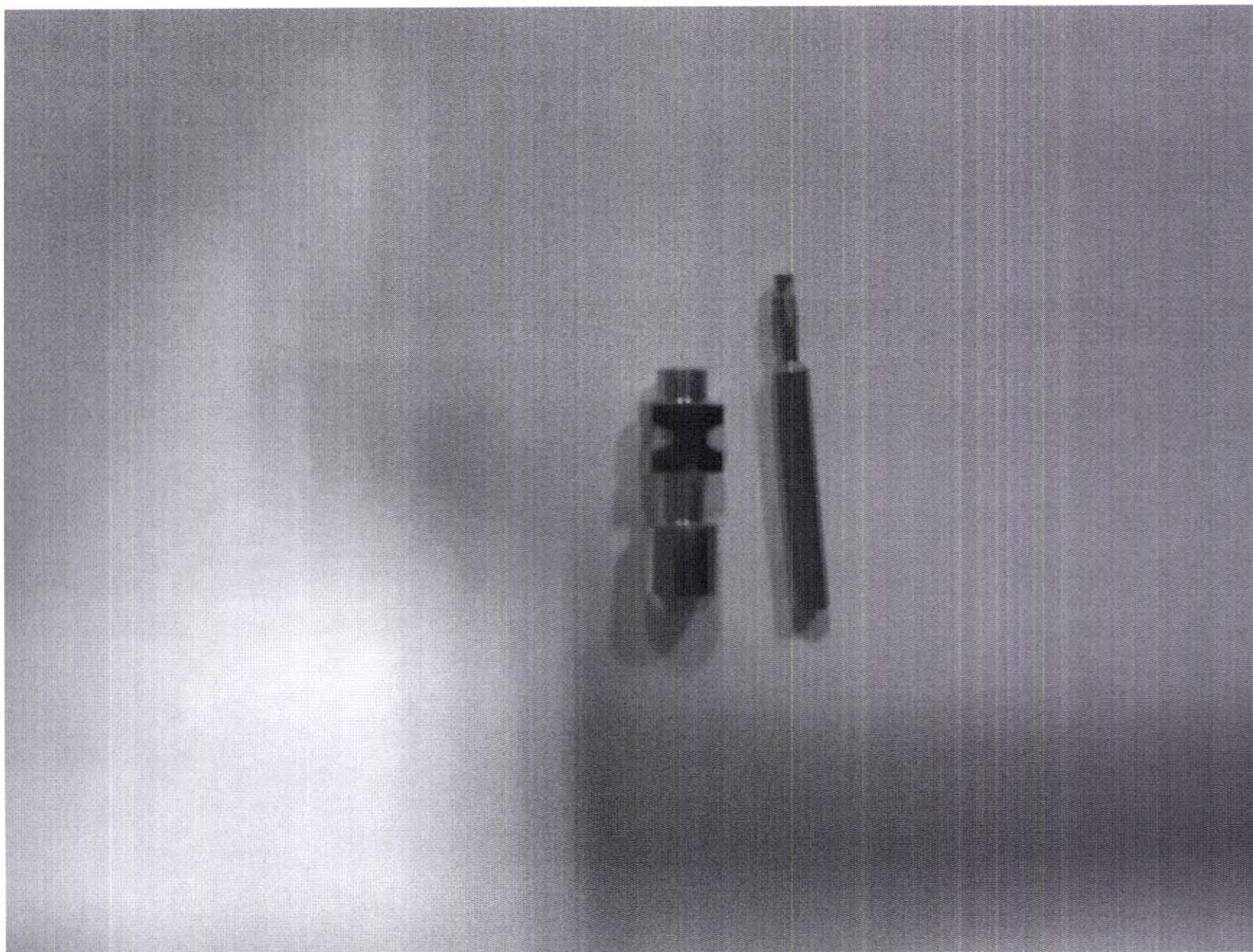
Трансфер для открытой ложки Impression Coping Open Tray Branemark System (Bmk Syst) в комплекте с пином. типоразмер NP, диаметр 4.5 мм
