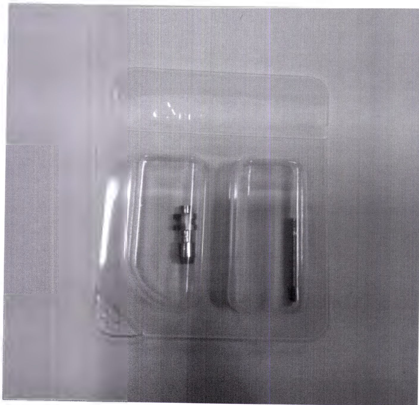
Трансфер для открытой ложки Impression Coping Open Tray Branemark System (Bmk Syst) Zygoma в комплекте с пином, диаметр 4 мм
