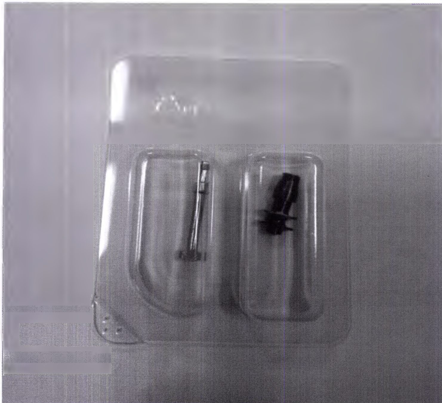
Трансфер для открытой ложки Impression Coping Open Tray Conical Connection (CC) в комплекте с винтом и кольцом O-Ring, типоразмер WP, размер 5x10 мм
