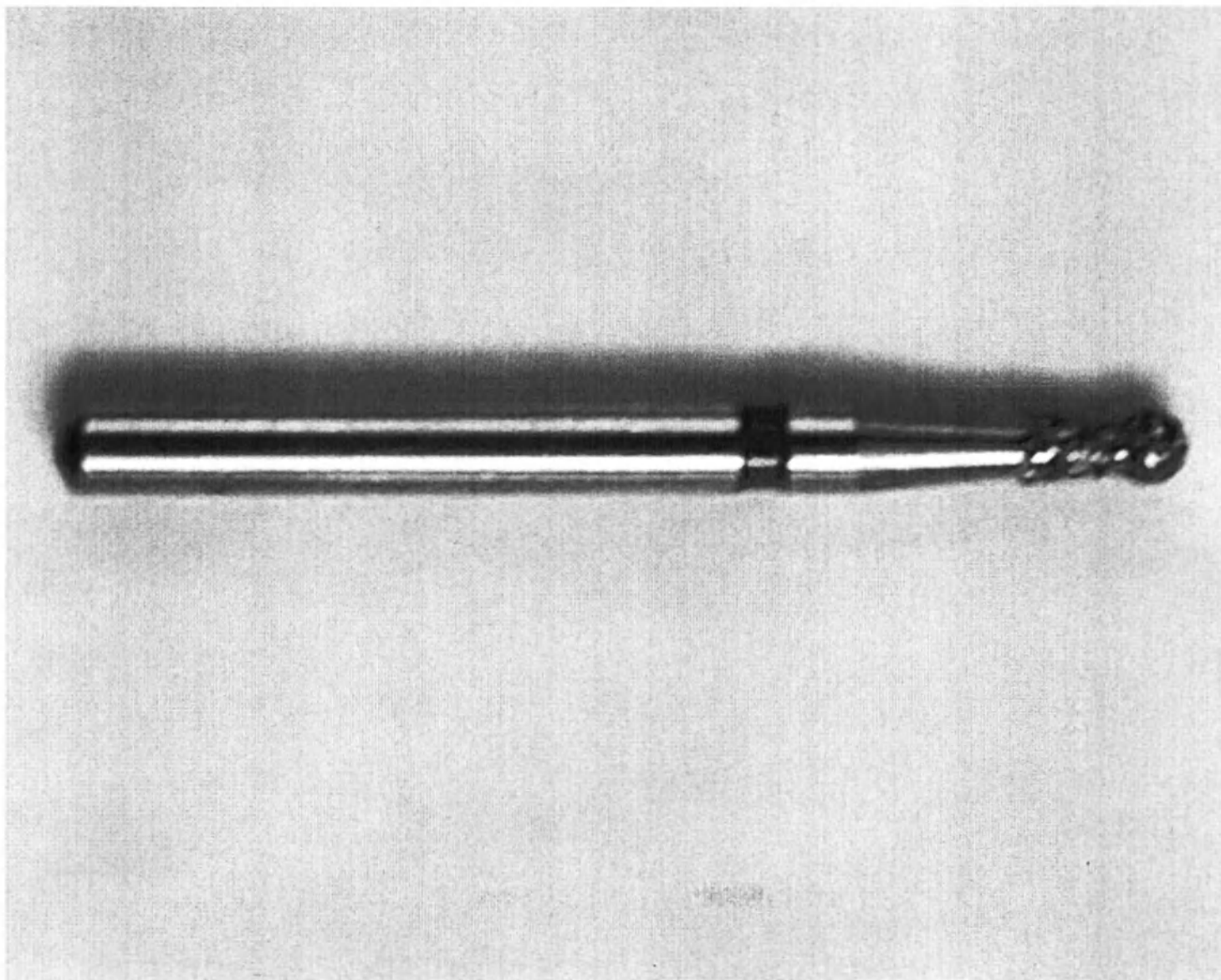
Бор алмазный шаровидный с воротничком стандартный, 802014CFG, 806314002534014
