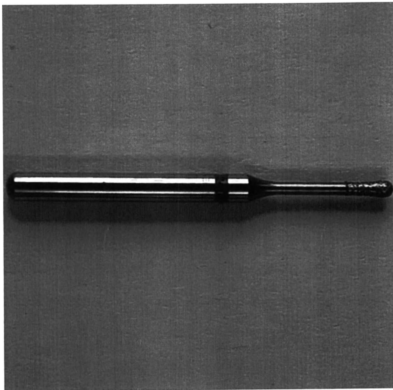
Бор алмазный грушевидный округлённый плоский стандартный, 830RS009FFG, 806RS314239514009
