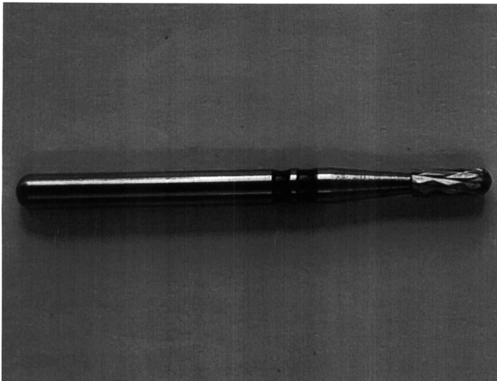
Бор твердосплавный для разрезания коронок, C4X012RA, 500204139019012
