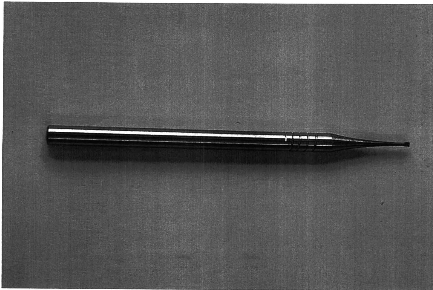
Бор твердосплавный обратный конус, H2007RA, 500204010001007
