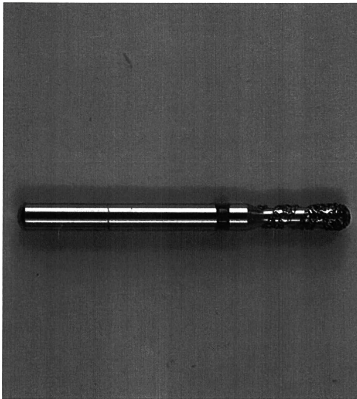
Бор алмазный Turbo грушевидный удлинённый стандартный, T830L016CFG, T806314239534016
