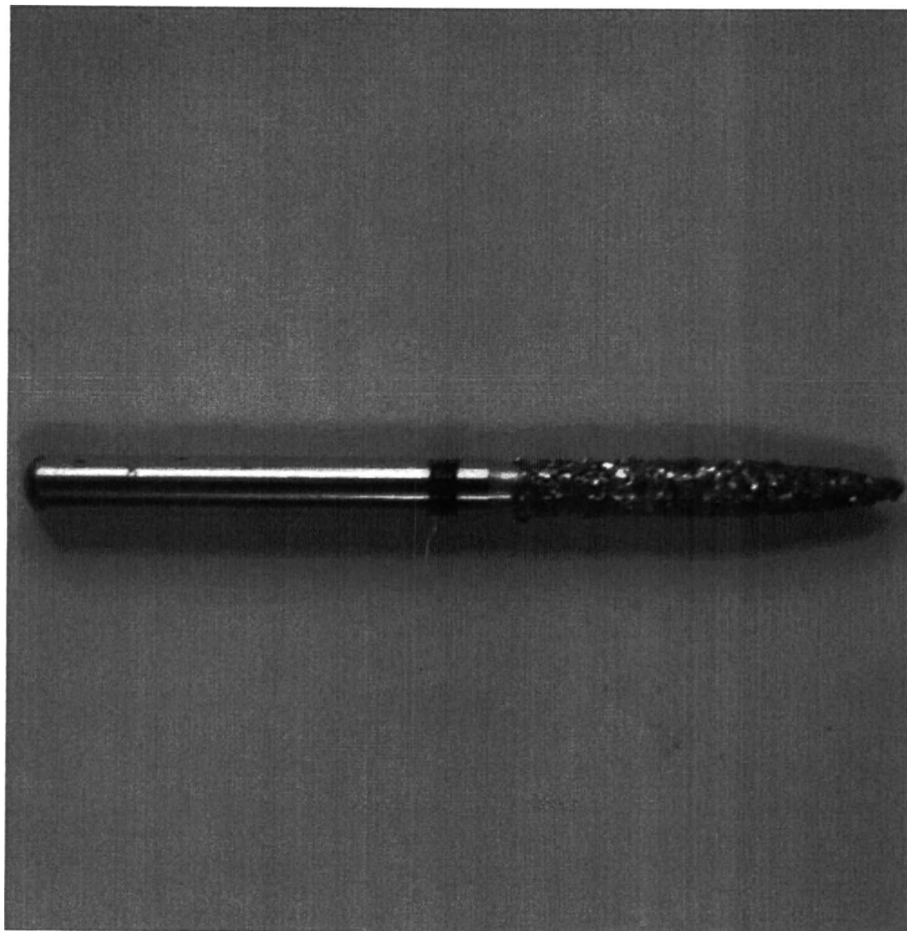
Бор алмазный Supra пламевидный стандартный, S863016CFG, S806314250534016
