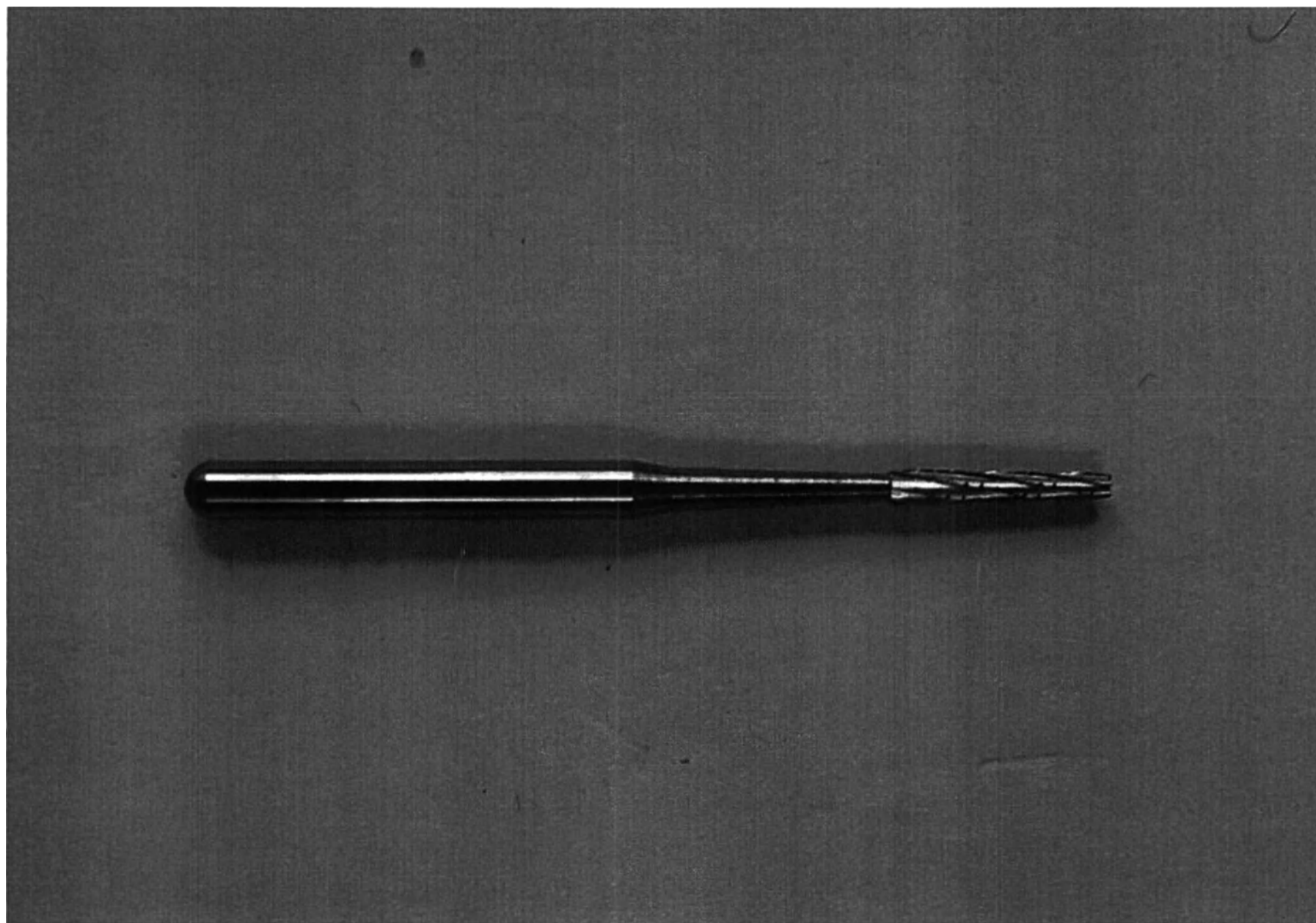
Бор твердосплавный цилиндр для пластиночных имплантатов, HF115010FGXL, 500316415296010
