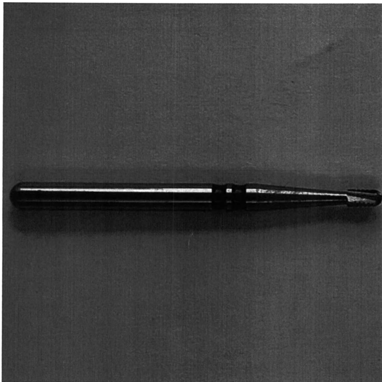
Бор твердосплавный для резания коронок, С34010FG, 500314138293010
