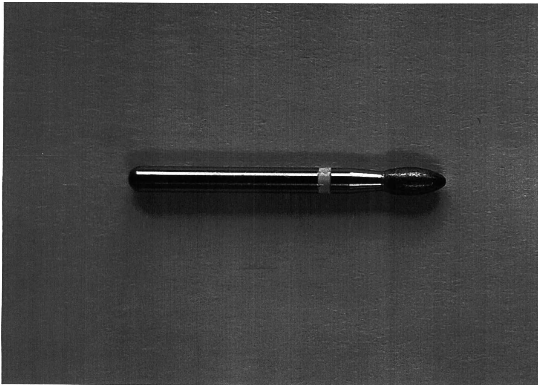
Бор алмазный почковидный стандартный, 379018UFFG, 806314277494018
