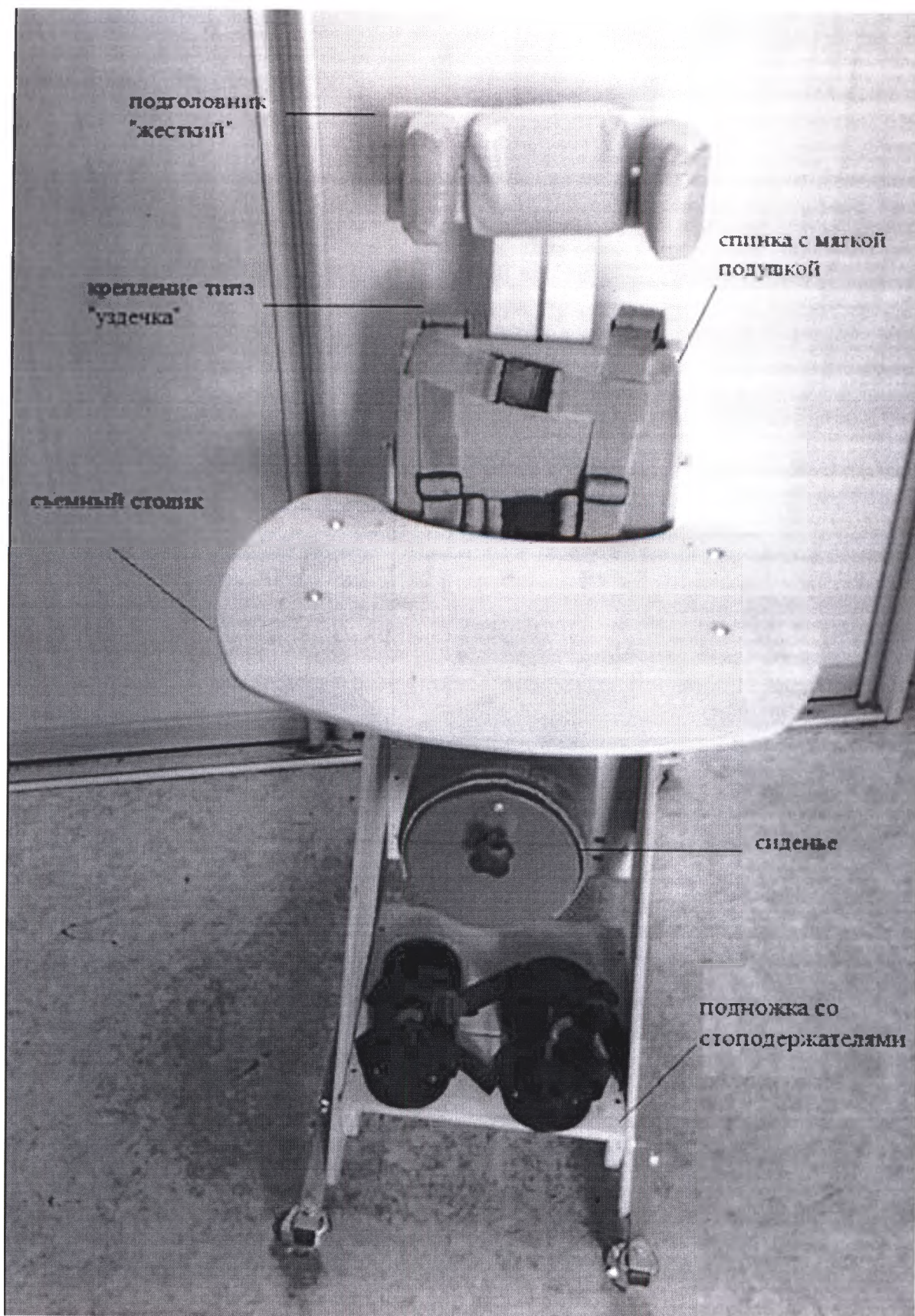
4-Опора функциональная для сидения для детей-инвалидов «Я МОГУ!», исполнение ОС-002. Принадлежности: съемный подголовник «жесткий»
