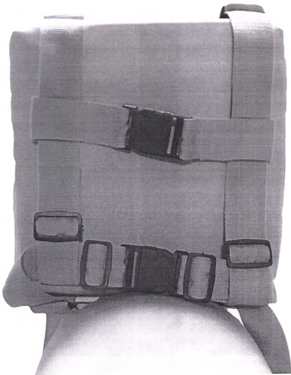
35-Съемный упор-спинка с системой крепления тела типа «уздечка»
