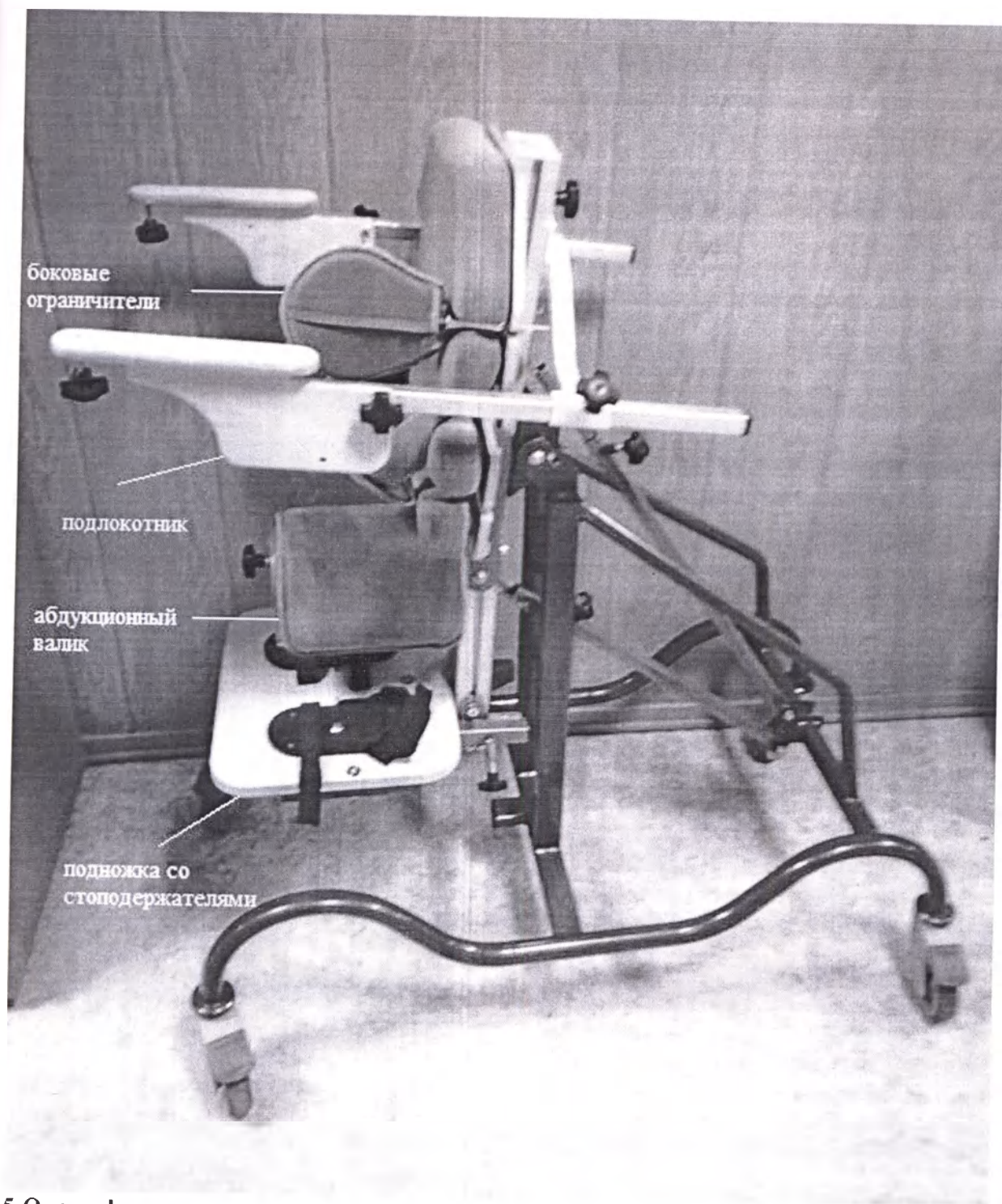
15-Опора функциональная для сидения для детей-инвалидов «Я МОГУ!», исполнение ОС-023. Принадлежности: съемные боковые ограничители, съемный абдукционный валик
