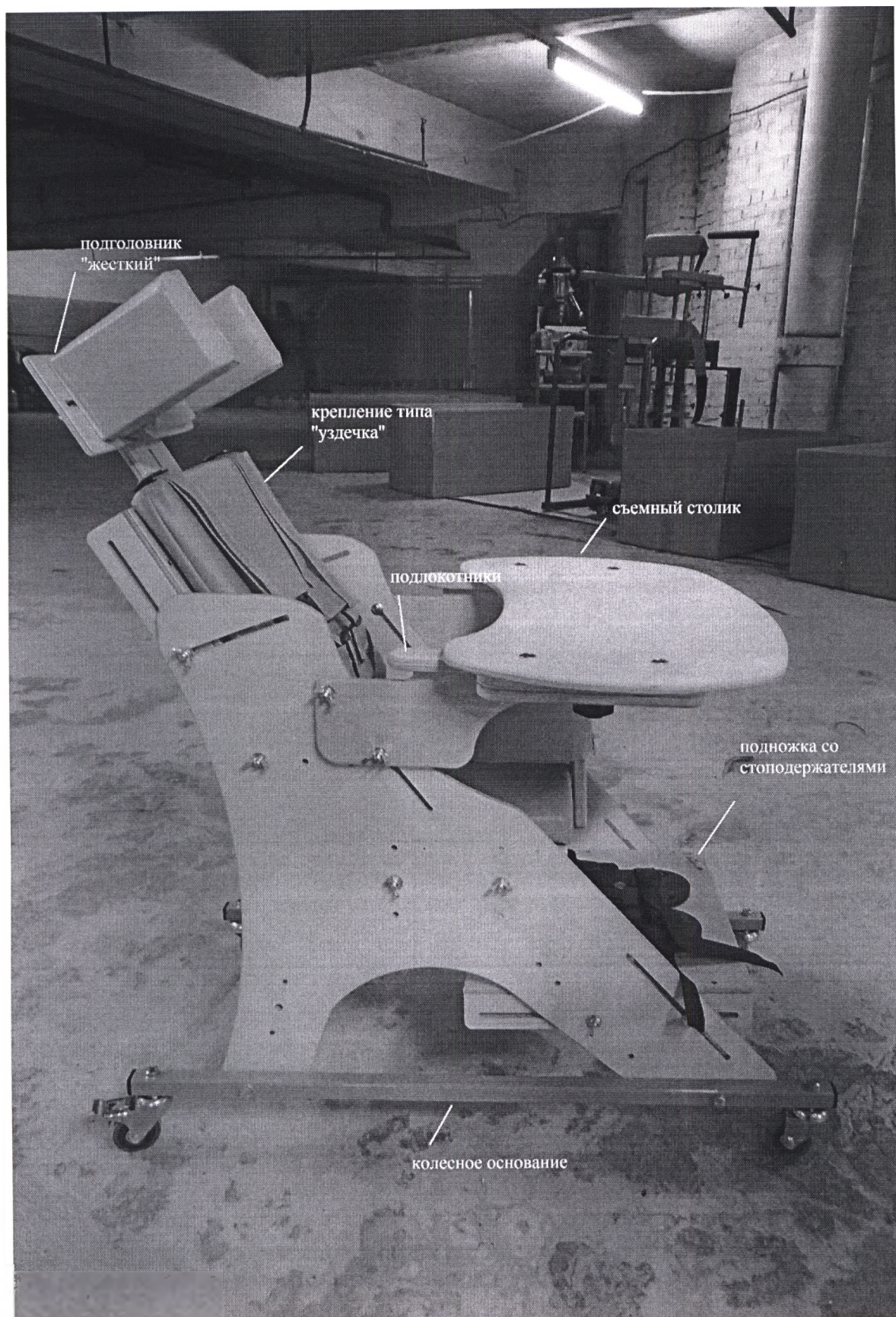
1-Опора функциональная для сидения для детей-инвалидов «Я МОГУ!», исполнение ОС-001 на примере размера 1. Принадлежности: съемный столик, съемный подголовник «жесткий»
