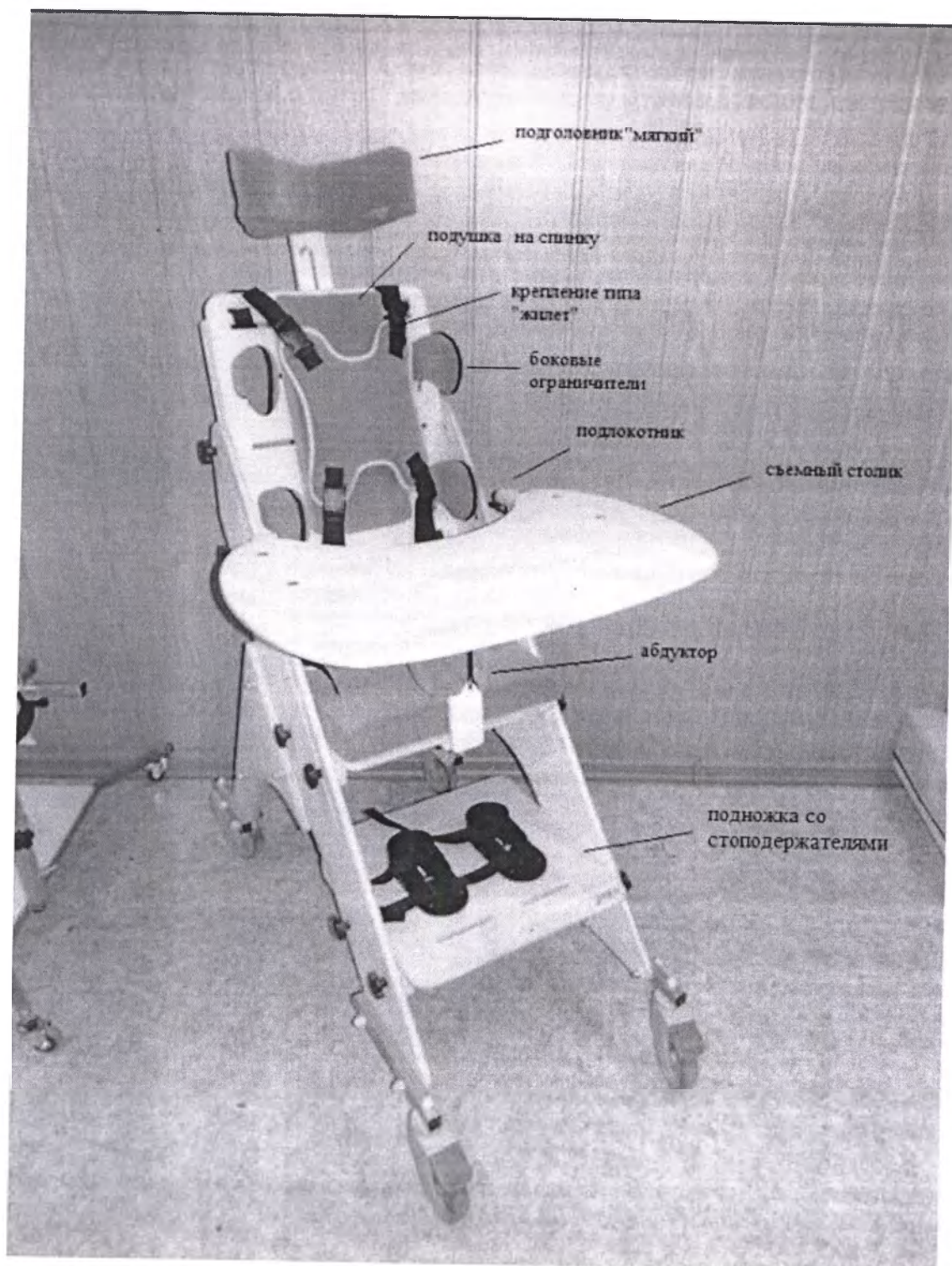
8-Опора функциональная для сидения для детей-инвалидов «Я МОГУ!», исполнение ОС-005. Принадлежности: съемный столик, съемный подголовник «мягкий», съемное крепление тела типа «жилет», съемная подушка на спинку, съемные боковые ограничители
