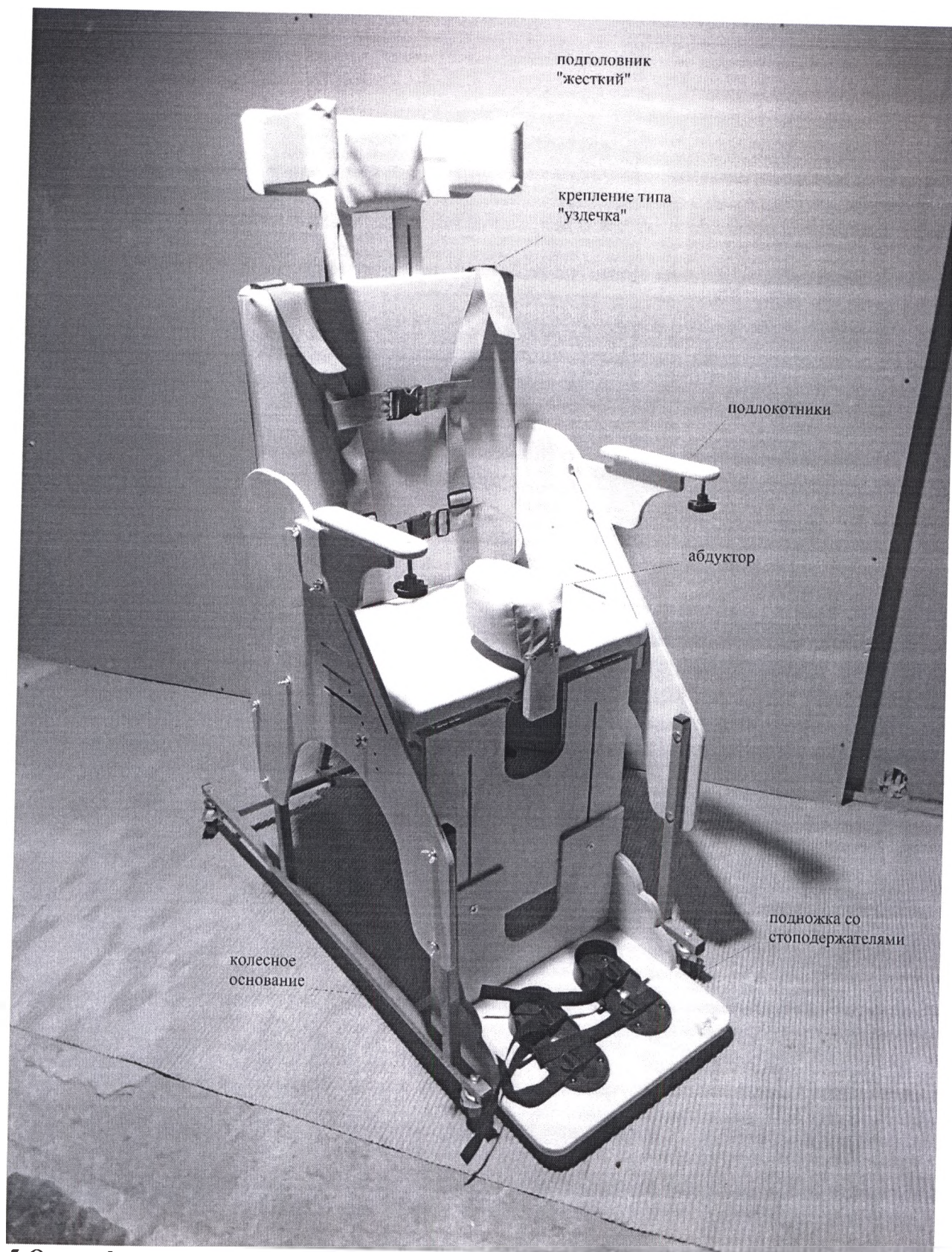
5-Опора функциональная для сидения для детей-инвалидов «Я МОГУ!», исполнение ОС-003. Принадлежности: съемный подголовник «жесткий»
