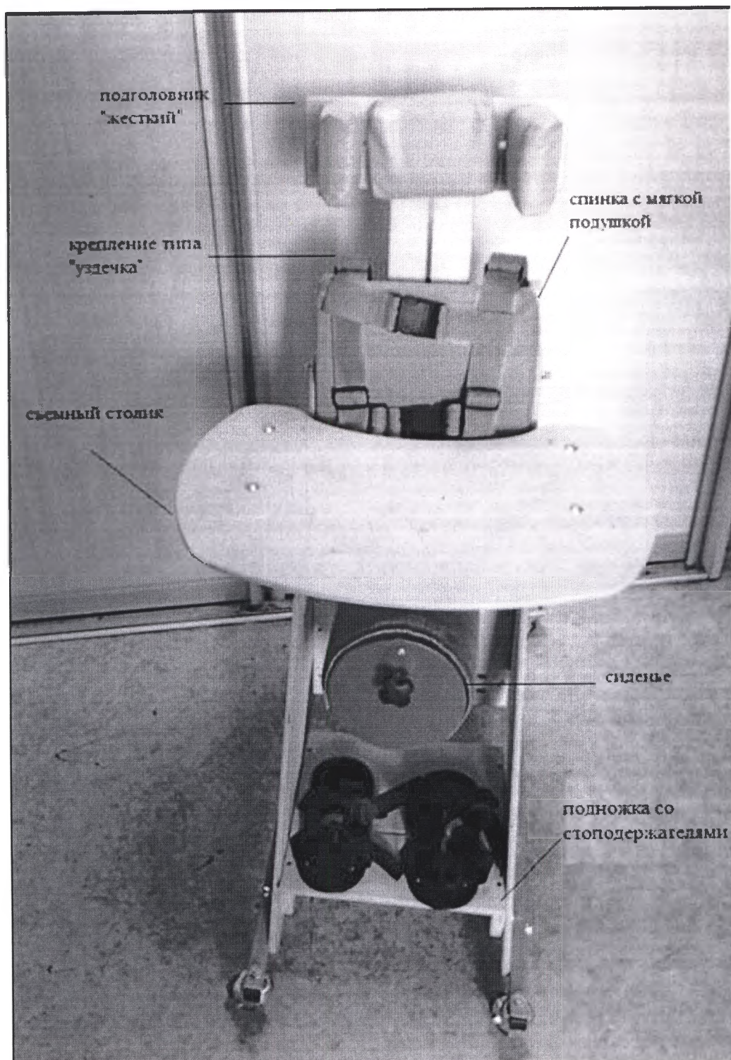
3-Опора функциональная для сидения для детей-инвалидов «Я МОГУ!», исполнение ОС-002. Принадлежности: съемный столик, съемный подголовник «жесткий»
